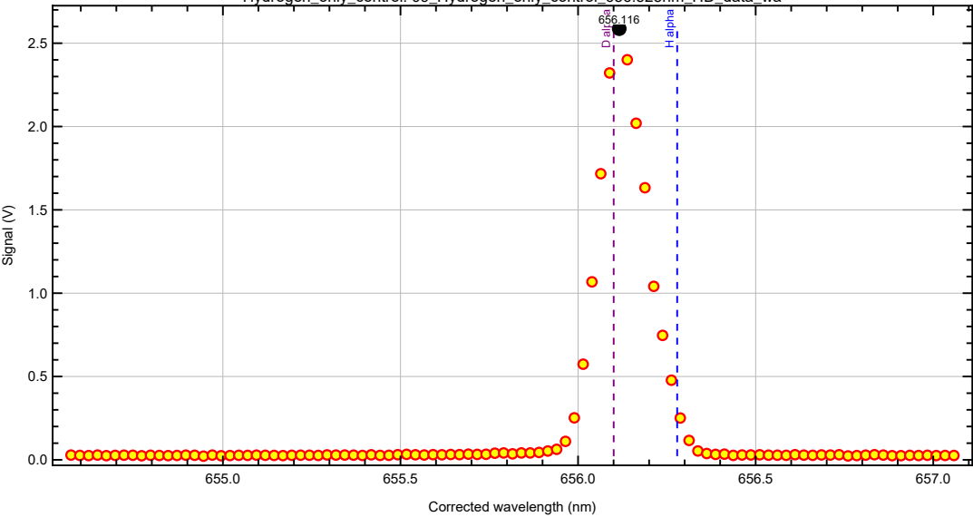
Hydrogen_only_control: 09_Hydrogen_only_control_656.525nm_HD_data_wa
