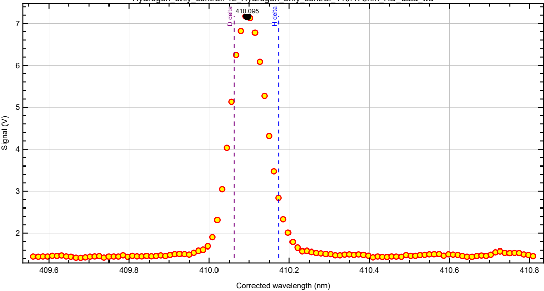
Hydrogen_only_control_12_Hydrogen_only_control_410.470nm_HD_data_wa
