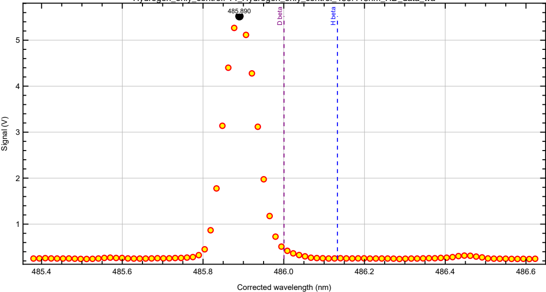
Hydrogen_only_control: 14_Hydrogen_only_control_486.418nm_HD_data_wa
