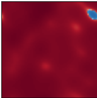
Gauss
