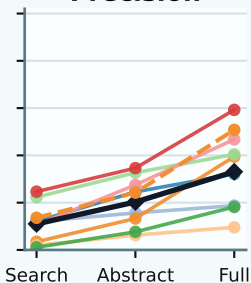
Precision
