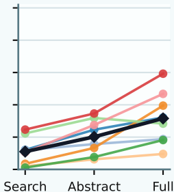
Precision
