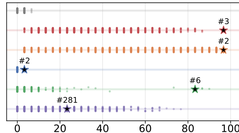
Llama-3.3-70B
