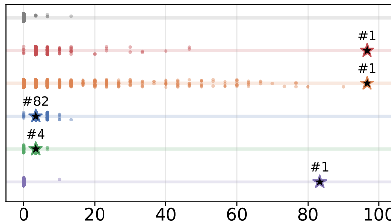
Gemma-3-12B
