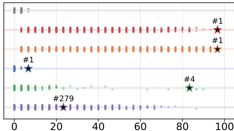
Llama-3.1-8B
