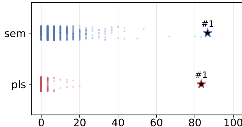
Llama-3.3-70B
