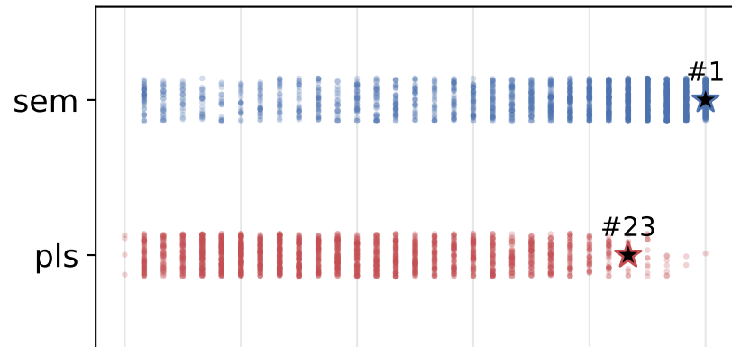
OLMo-3-7B
