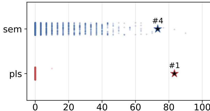
Gemma-3-12B
