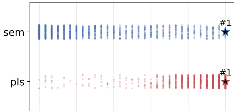
Qwen3-4B
