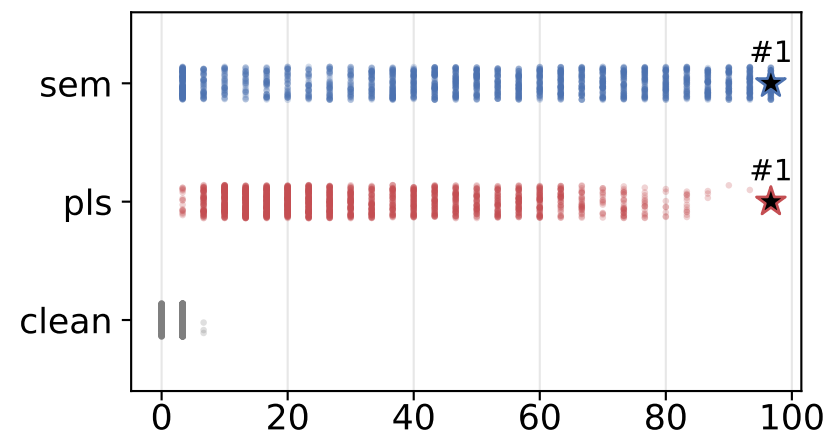
Llama-3.1-8B
