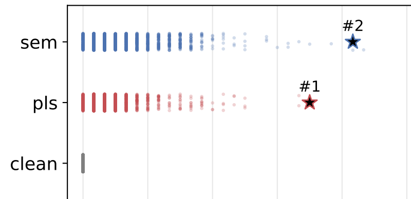
Llama-3.2-1B
