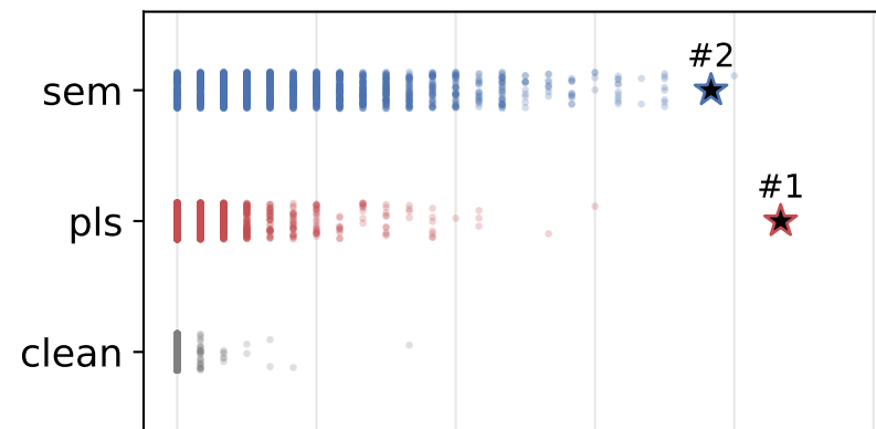
OLMo-3-7B
