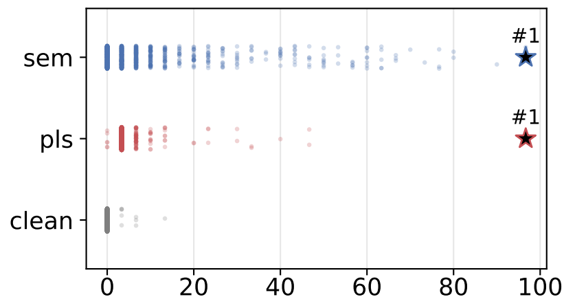
Gemma-3-12B
