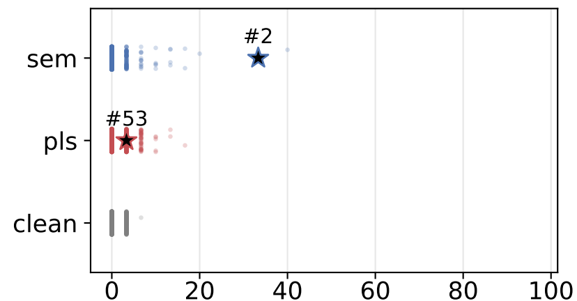
Llama-3.3-70B
