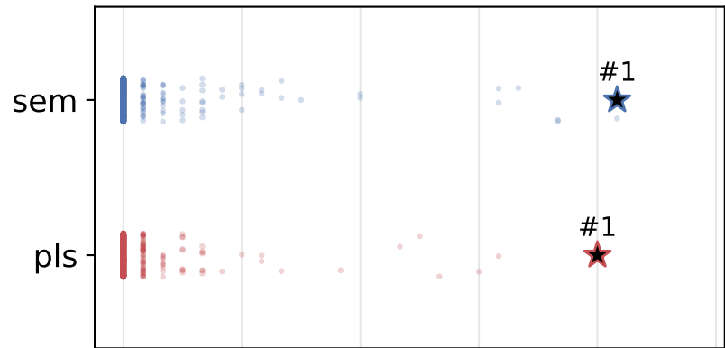
Llama-3.2-1B
