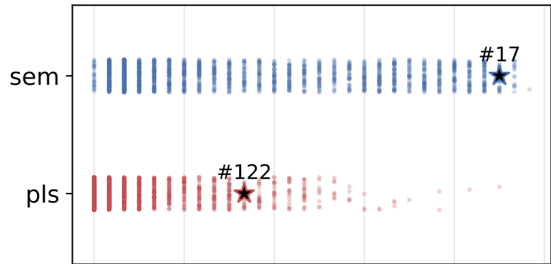
Qwen3-4B
