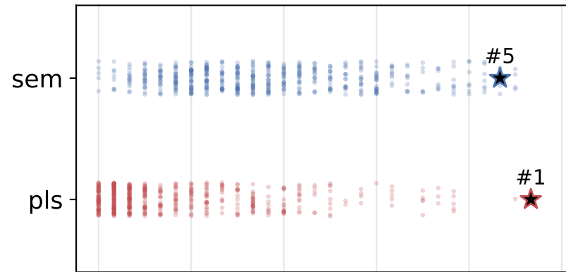
OLMo-3-7B
