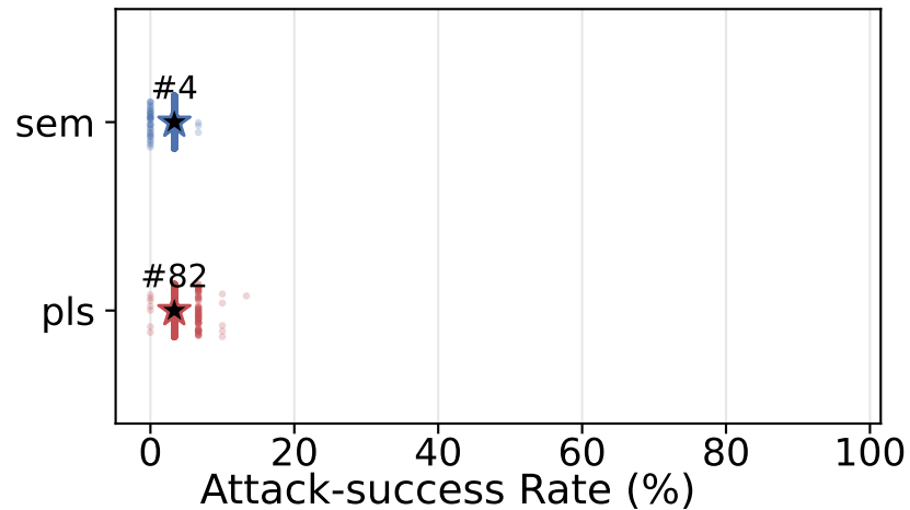
Gemma-3-12B
