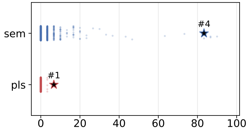
Llama-3.1-8B
