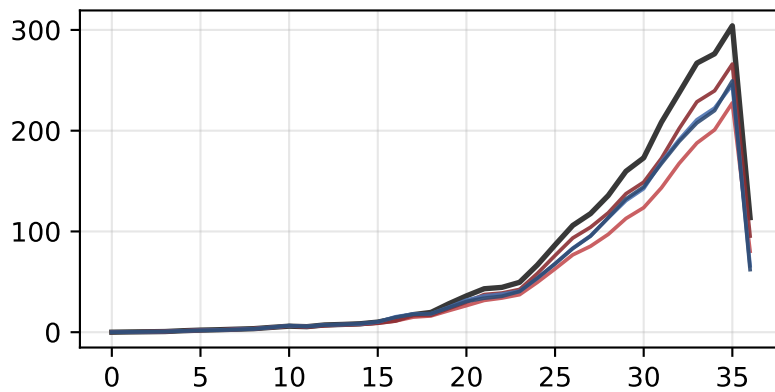
Gemma-3-12B
