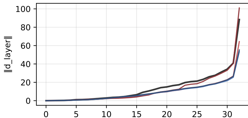
Llama-3.1-8B
