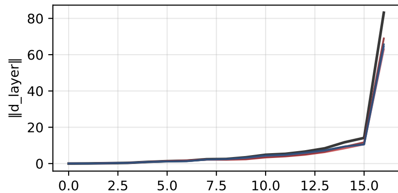
Llama-3.1-8B
