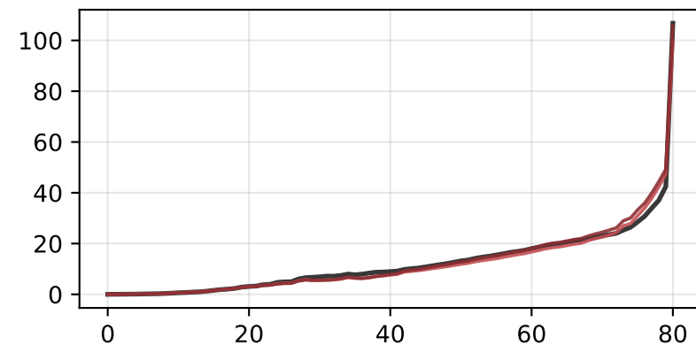
Llama-3.3-70B
