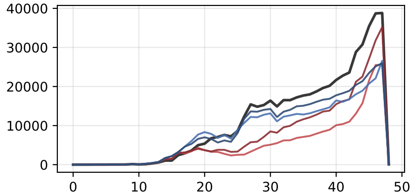
Gemma-3-12B
