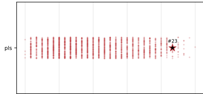
OLMo-3-7B
