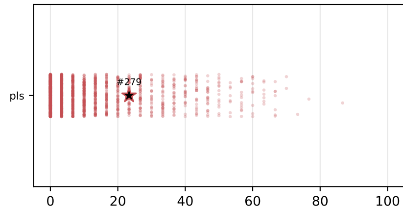
Llama-3.1-8B
