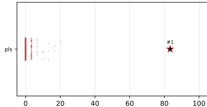
Llama-3.3-70B
