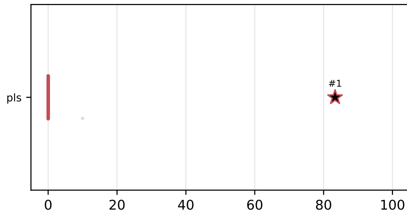
Gemma-3-12B
