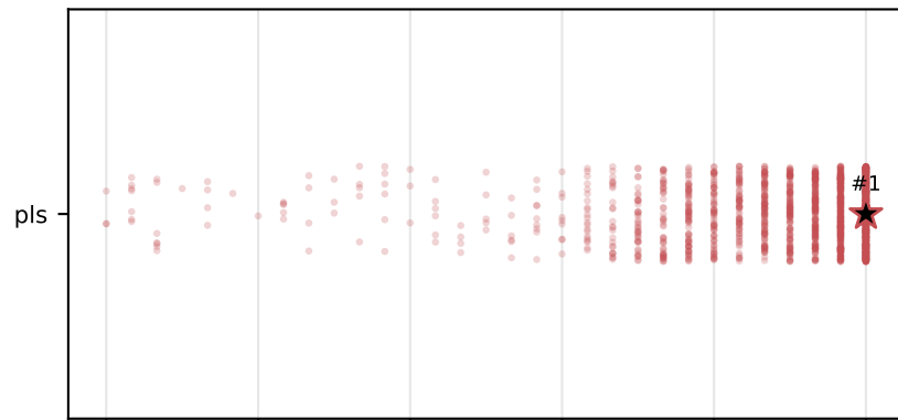
Qwen3-4B
