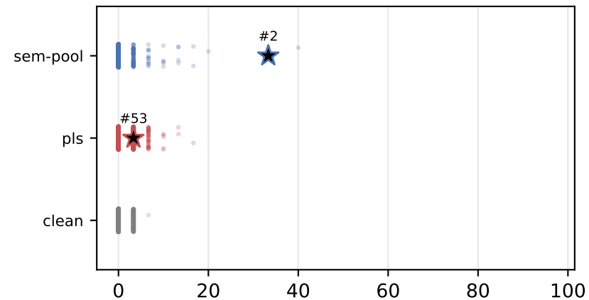
Llama-3.3-70B
