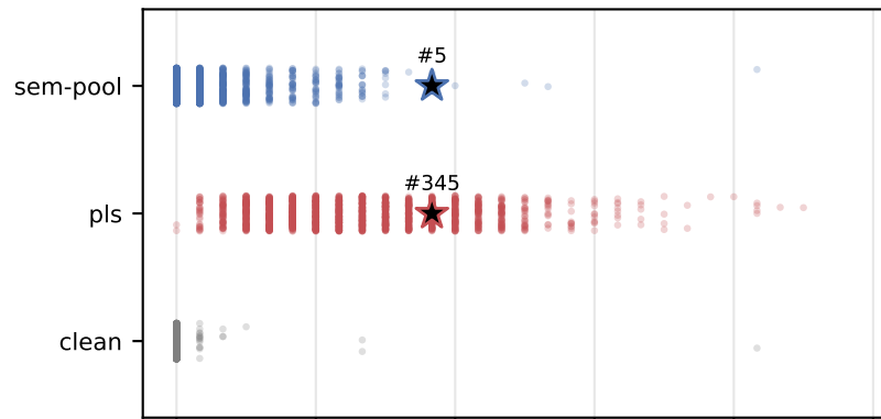
Qwen3-4B
