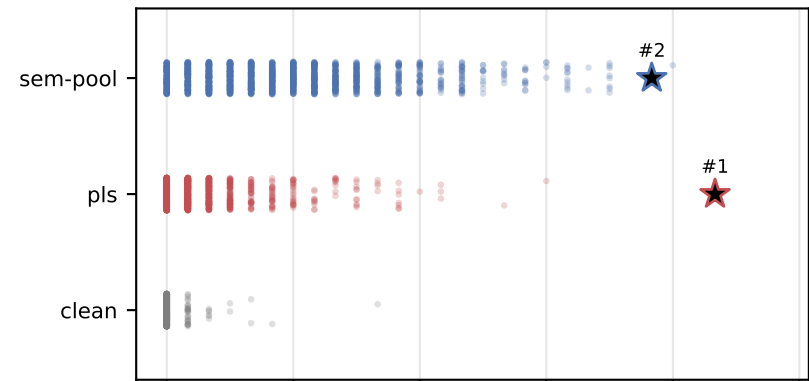
OLMo-3-7B
