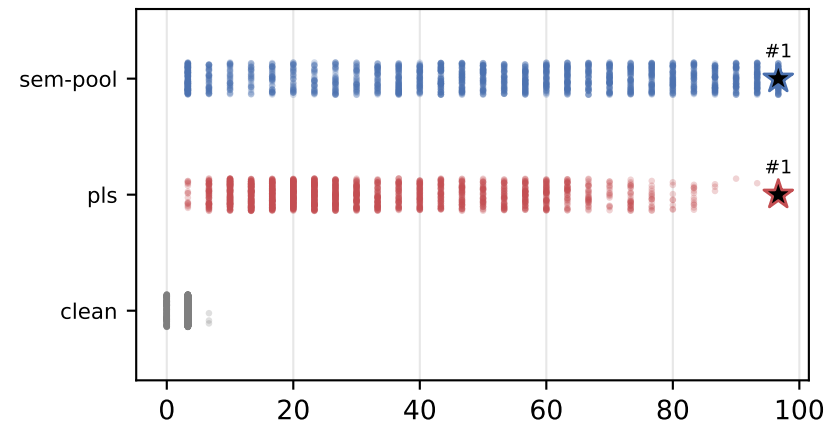
Llama-3.1-8B
