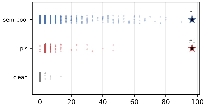
Gemma-3-12B
