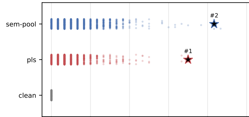
Llama-3.2-1B
