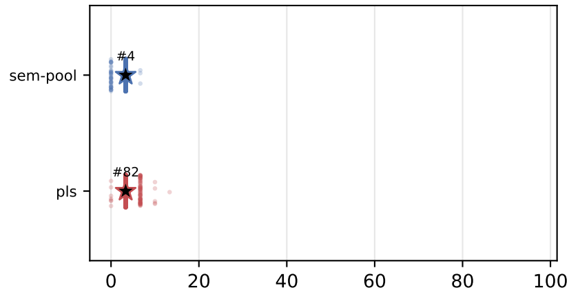
Gemma-3-12B
