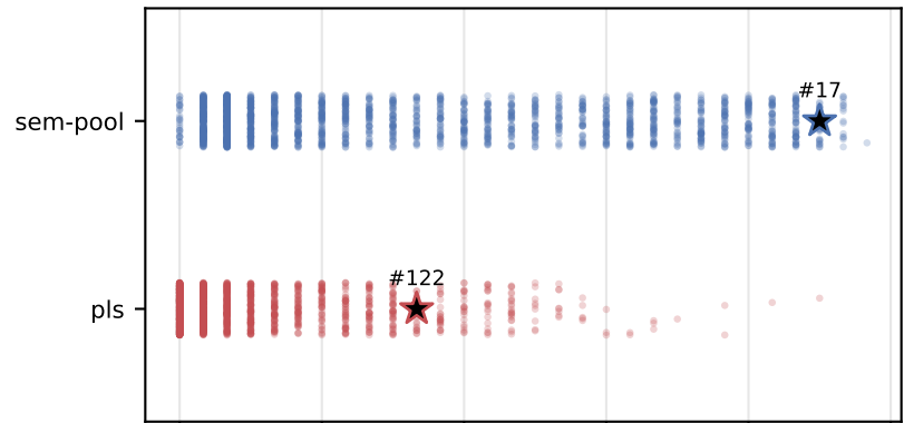
Gemma-3-12B
