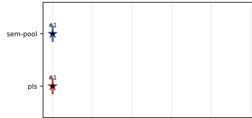
OLMo-3-7B
