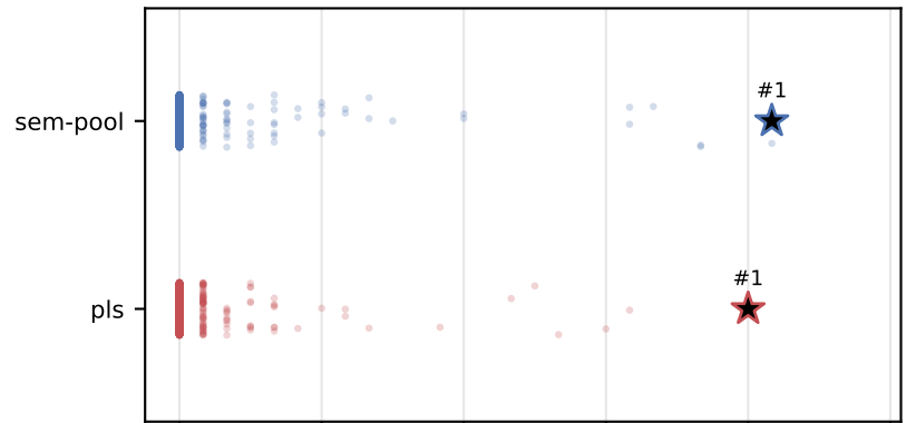
Llama-3.1-8B
