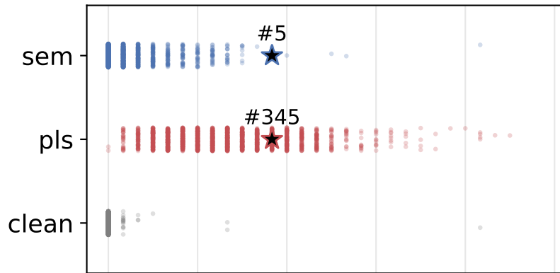
Qwen3-4B
