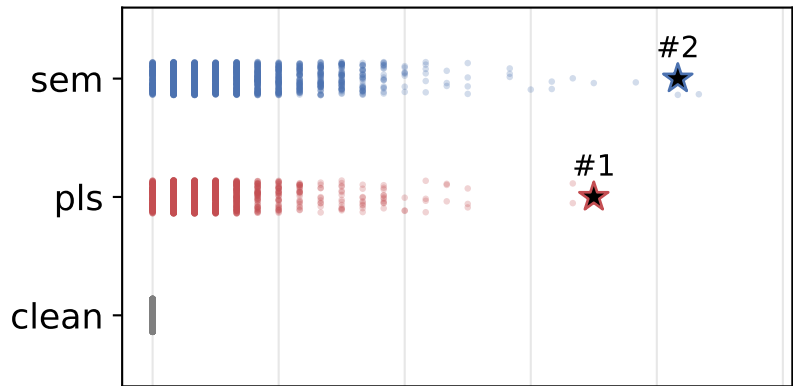
Llama-3.2-1B
