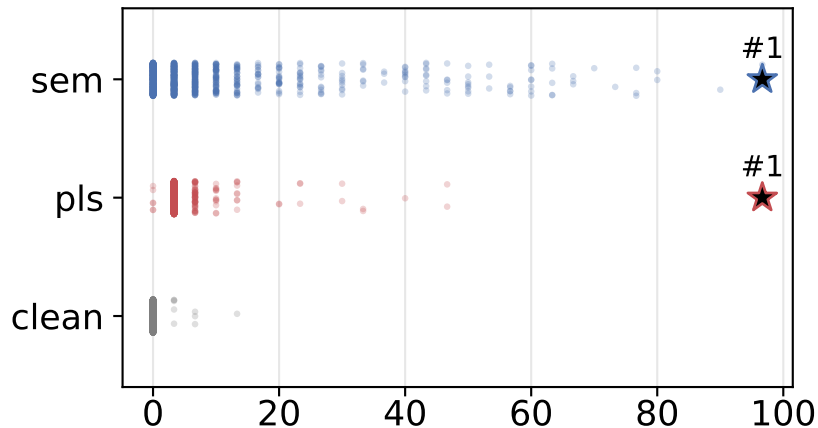
Gemma-3-12B
