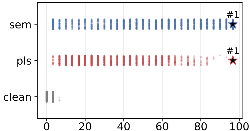
Llama-3.1-8B
