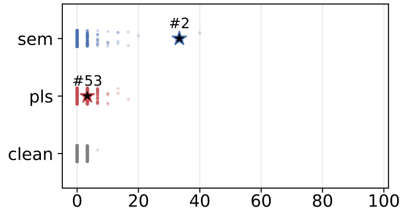
Llama-3.3-70B
