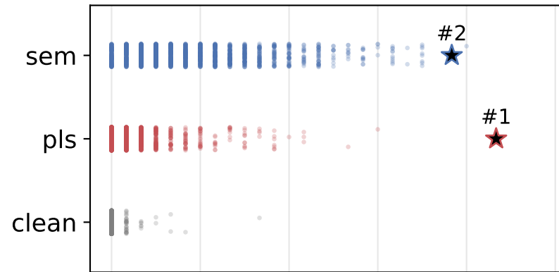
OLMo-3-7B
