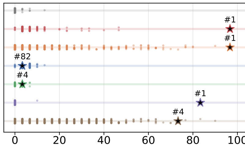
Gemma-3-12B
