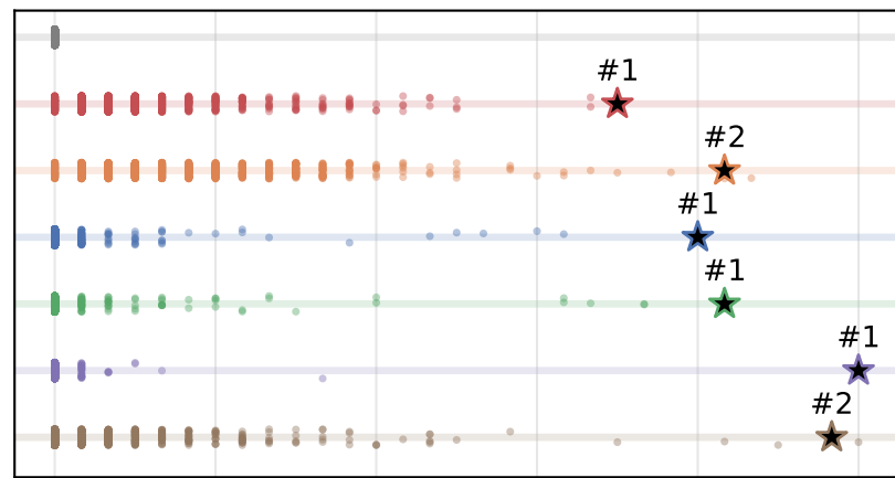
Llama-3.2-1B
