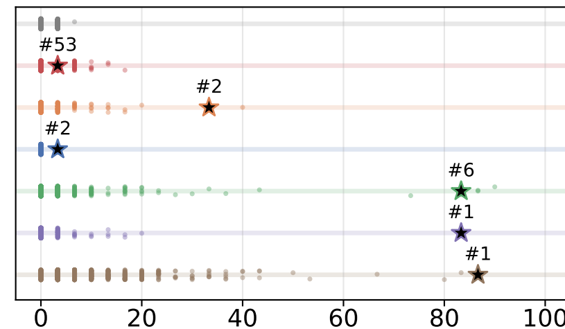
Llama-3.3-70B
