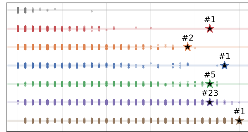
OLMo-3-7B
