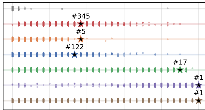
Qwen3-4B
