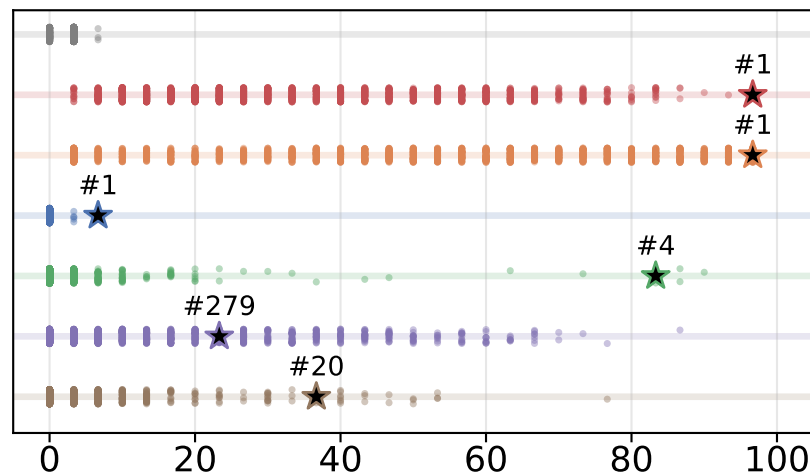
Llama-3.1-8B
