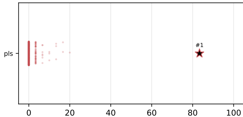
Llama-3.3-70B
