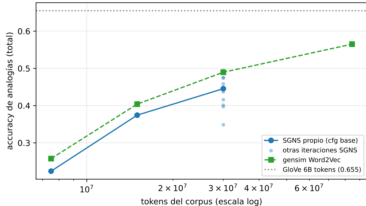
Analogías vs tamaño del corpus
