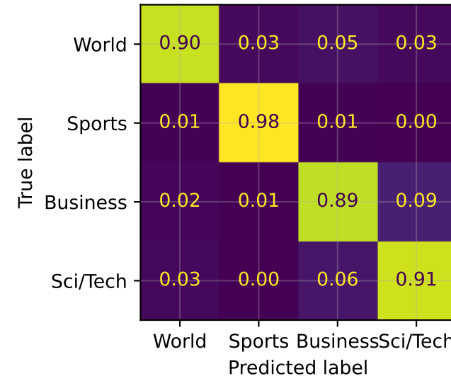
GloVe fine-tuning F1 test = 0.9183
