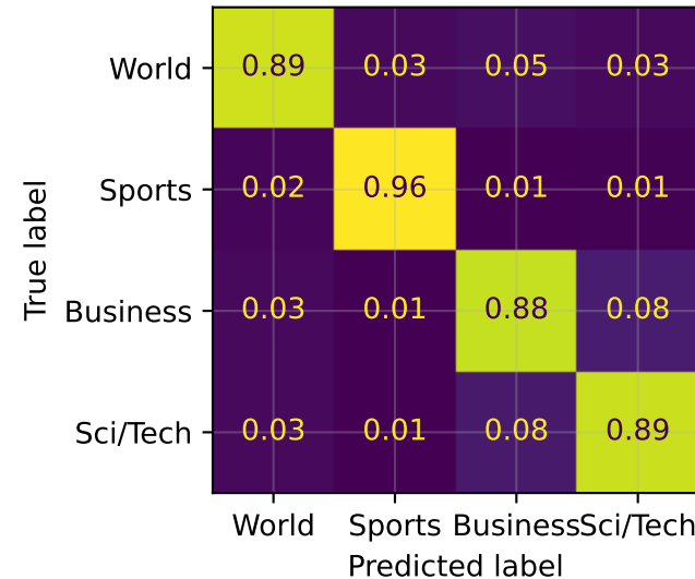
Aleatorio F1 test = 0.9055
