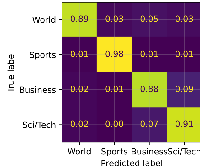
gensim fine-tuning F1 test = 0.9136
