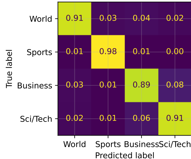
TF-IDF + LogReg F1 test = 0.9211
