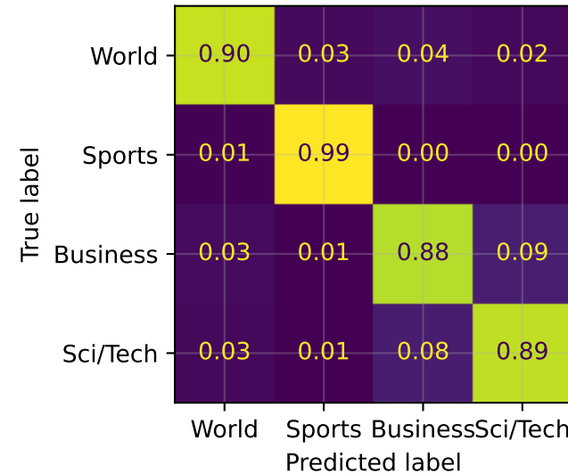
SGNS fine-tuning F1 test = 0.9139
