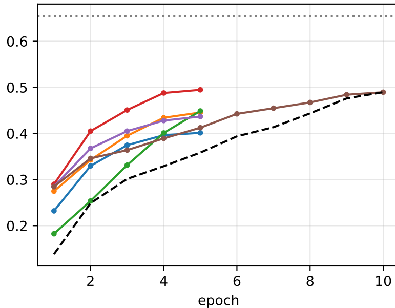
Accuracy de analogías (total)
