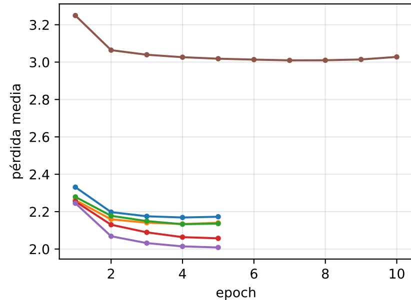
Pérdida SGNS por epoch
