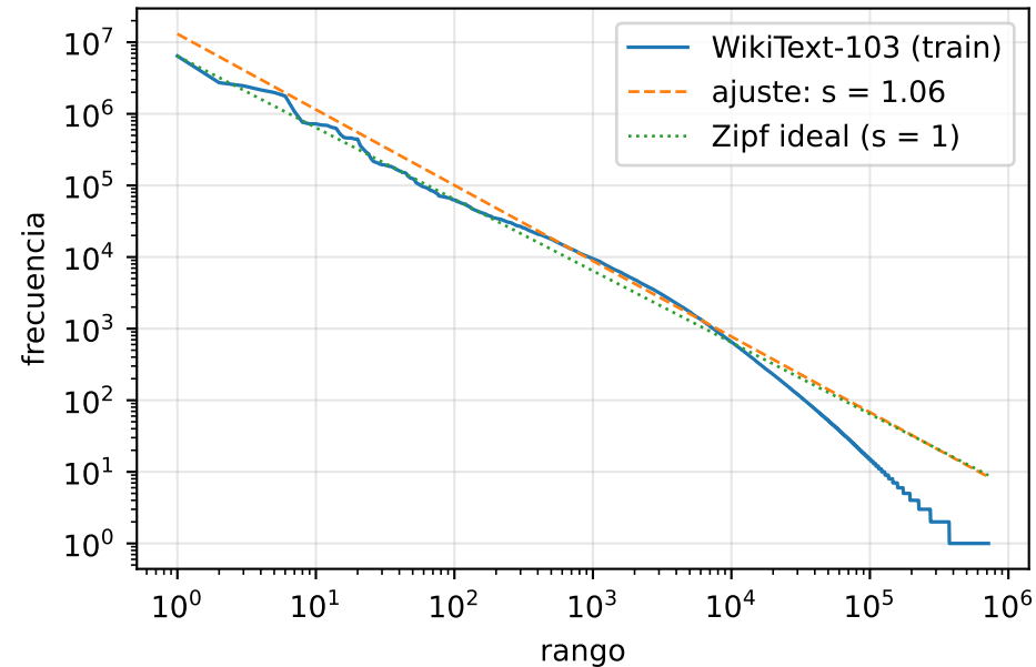
Frecuencia vs rango (log-log)
