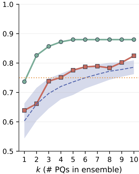
GPT-5.1
