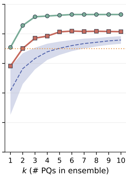
Claude Sonnet 4.6
