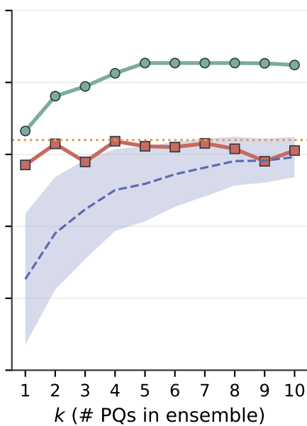
GPT-5.4
