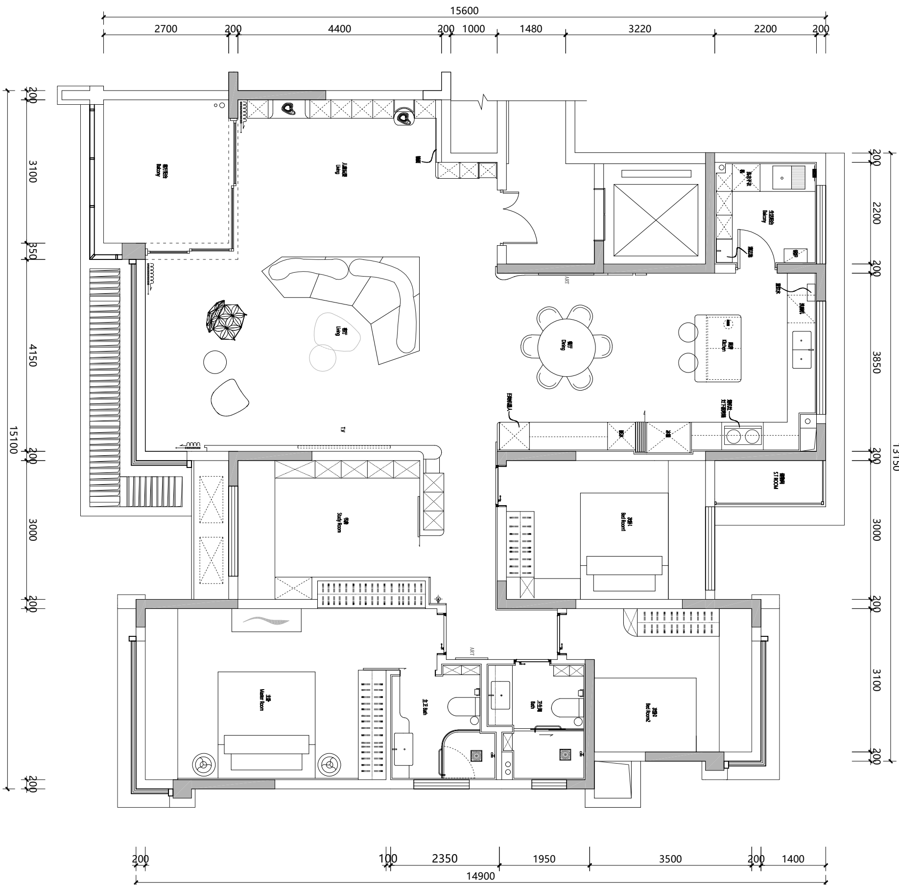
平面布置图 SCALE 1:80
