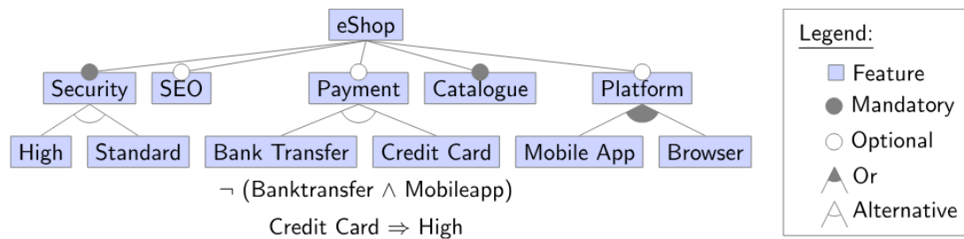
Figura 2.2: Ejemplo de modelo de características. Extraído de [14].
