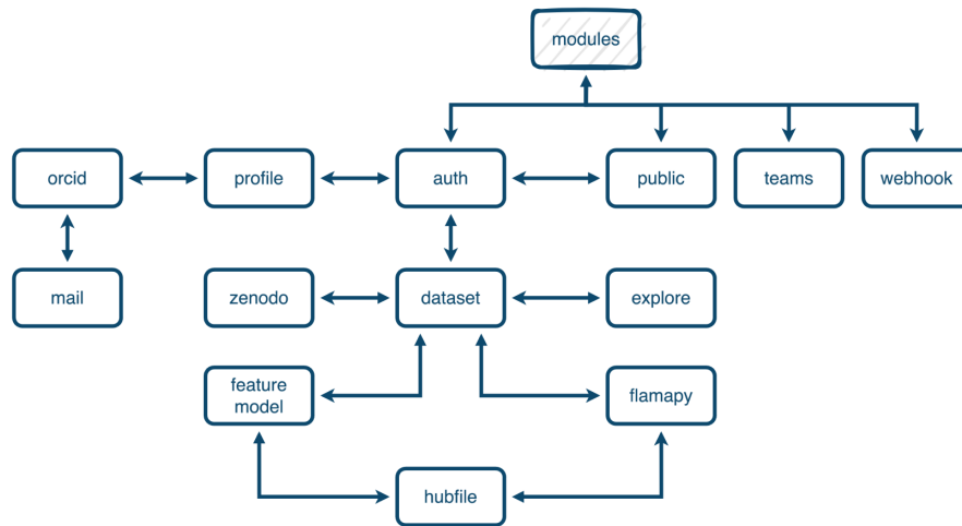
Figura 2.6: Arquitectura general de UVLHub y sus integraciones principales. Extraído de [16]
