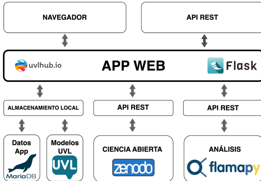
Figura 2.5: Arquitectura general de UVLHub y sus integraciones principales. Extraído de [16]
