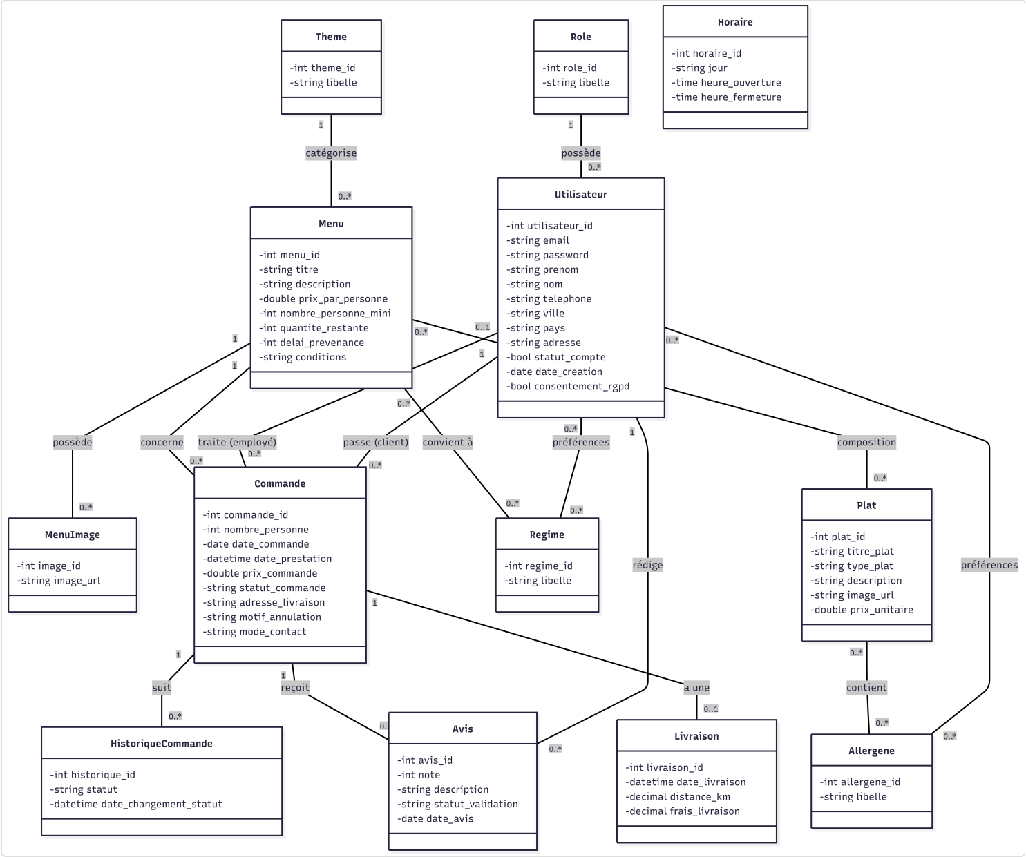
Modèle conceptuel de données (diagramme de classes) — 18 tables, dont 6 tables de liaison pour les relations Plusieurs-à-Plusieurs.
