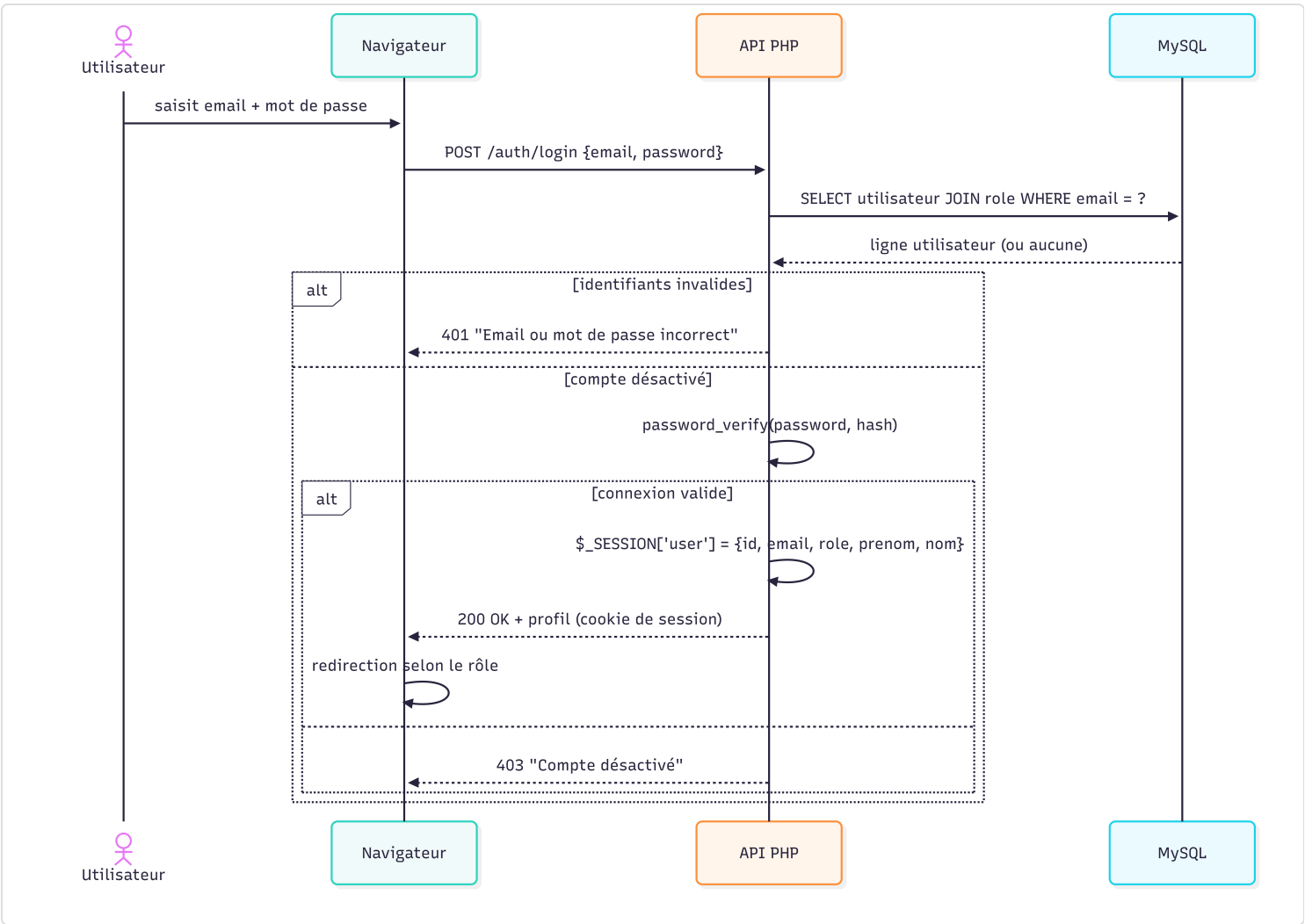
Diagramme de séquence — parcours de connexion sécurisé.
