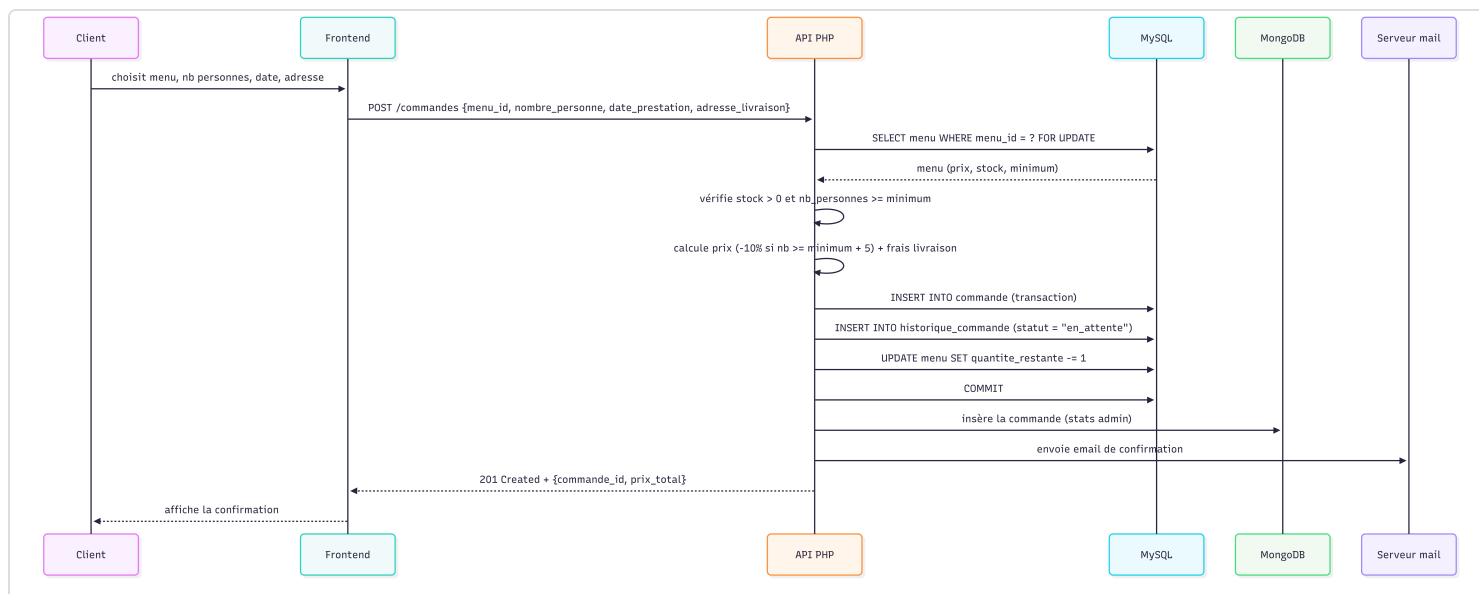
Diagramme de séquence — création d'une commande (transaction et double persistance).
