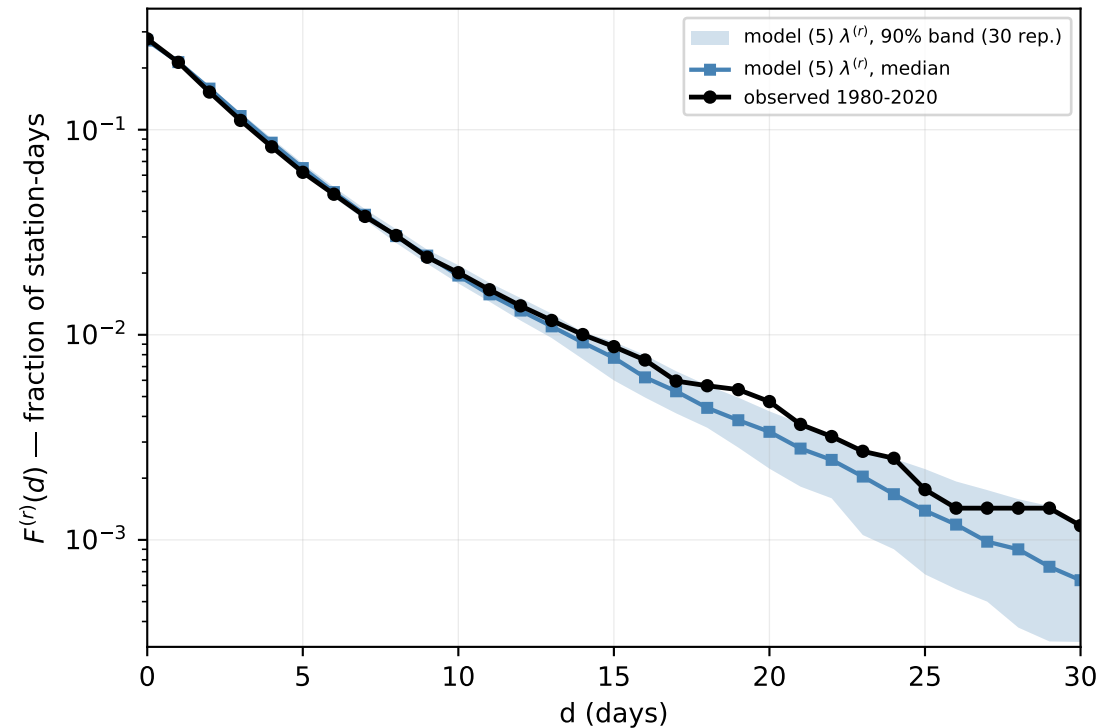
wet spells
