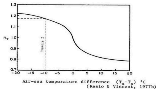
Fig. 6. – Ratio d'amplification permettant de prendre en compte les différences de température air-mer (U.S. Army Corps of Engineers, Coastal Engineering Research Center, 1984, p. 3-31)
