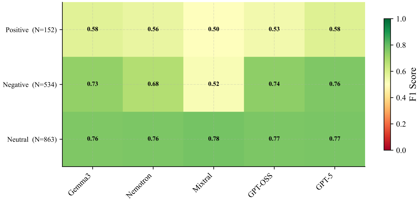
Per-Class F1 Scores — Sentiment
