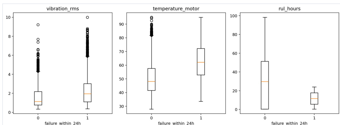
FIGURE 17 – Distribution des variables clés selon le statut de panne. La séparation nette des médianes (température, vibration, RUL) justifie leur pouvoir prédictif observé plus loin.
