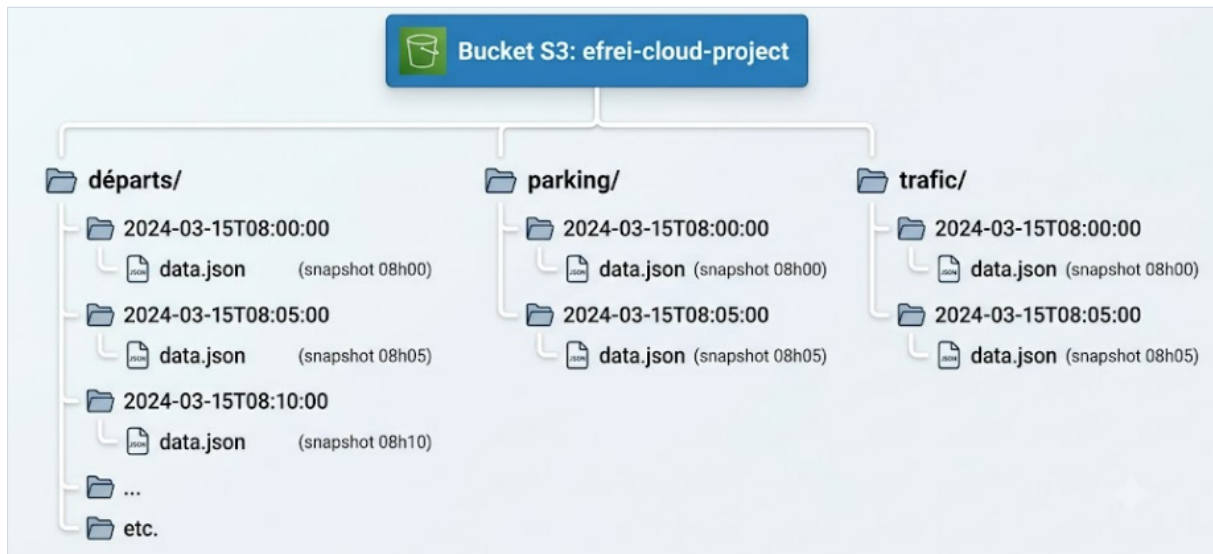
FIGURE 10 – Organisation du bucket S3 efrei-cloud-project : un préfixe par source ( départs , parking , trafic ) et, sous chacun, un dossier horodaté par snapshot contenant le fichier data.json .
