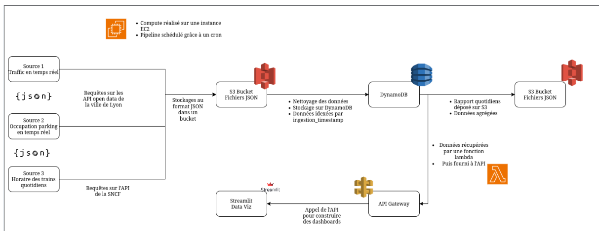
FIGURE 9 – Architecture technique du projet cloud . Les trois sources open data sont collectées par un pipeline ordonné par crontab sur EC2, stockées en JSON dans S3, nettoyées et indexées dans DynamoDB, agrégées dans un rapport quotidien, puis exposées via une fonction Lambda et une API Gateway consommée par le dashboard Streamlit.
