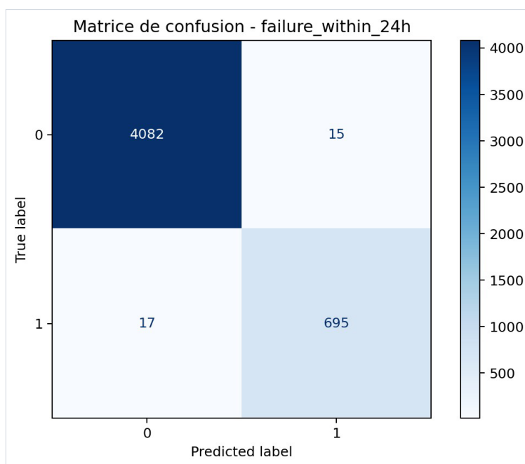
FIGURE 21 – Matrice de confusion de la tâche binaire (modèle gradient_boosting ). Sur le jeu de test, seuls 17 faux négatifs et 15 faux positifs subsistent face à 4 082 vrais négatifs et 695 vrais positifs.
