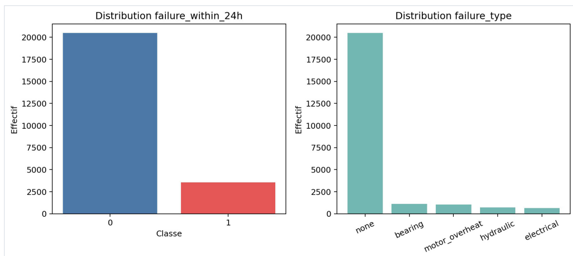
FIGURE 16 – Distribution des deux cibles. La classe positive failure_within_24h=1 ne représente que 14,8 % des observations, et la cible failure_type est dominée par la classe none (85 %). Ce déséquilibre impose le F1-score et la PR-AUC comme métriques, ainsi qu'un split stratifié .
