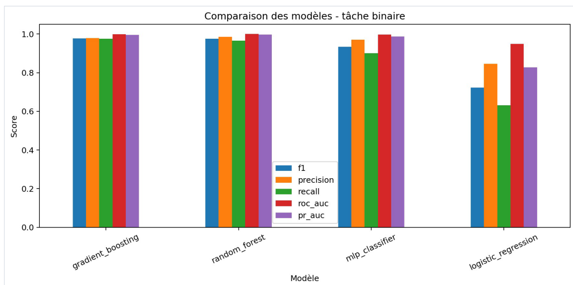
FIGURE 19 – Comparaison visuelle des quatre modèles sur la tâche binaire (F1, précision, rappel, ROC-AUC, PR-AUC). Les deux modèles d'ensemble dominent ; la régression logistique décroche nettement sur le rappel et la PR-AUC.
