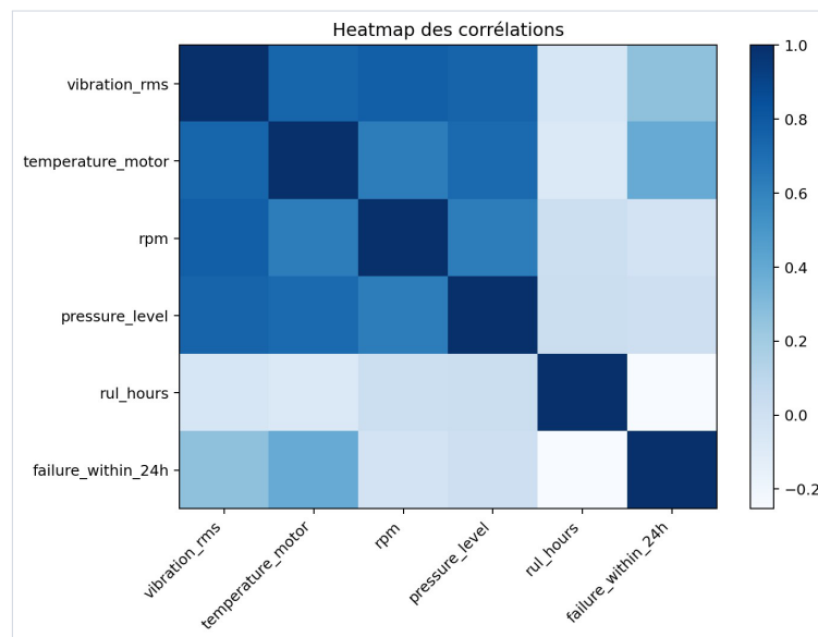
FIGURE 18 – Carte de chaleur des corrélations. La température moteur (+0,39), la vibration (+0,26) et la durée de vie résiduelle (−0,25) sont les plus corrélées à la cible binaire.
