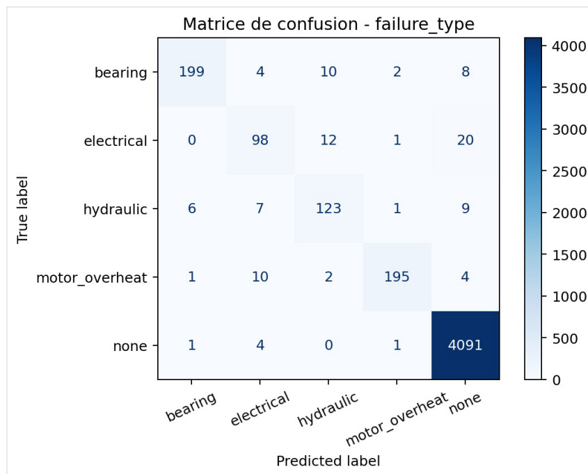
FIGURE 22 – Matrice de confusion de la tâche multiclass (modèle random_forest , 5 classes). La diagonale dominante confirme la qualité globale ; les erreurs se concentrent sur les classes minoritaires.
