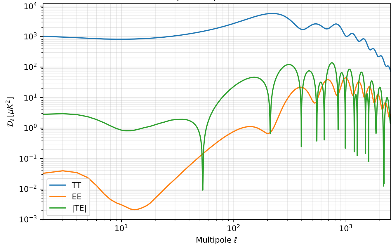
Scalar CMB power spectra (tutorial code)
