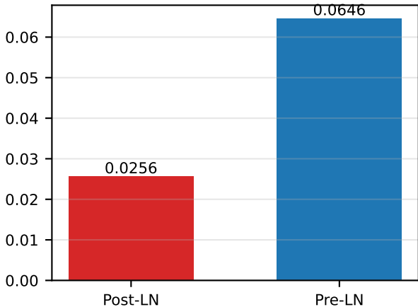
BLEU Score
