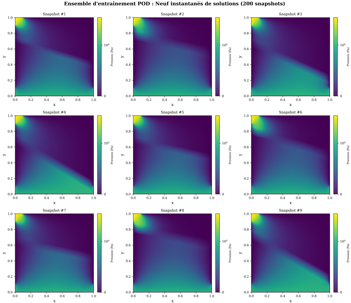
FIGURE 2 – Neuf snapshots représentatifs de l'ensemble d'entraînement. Bien que la position et la conductivité de la fracture varient considérablement, le champ de pression conserve une topologie globale similaire, ce qui garantit le succès de l'approche POD.
