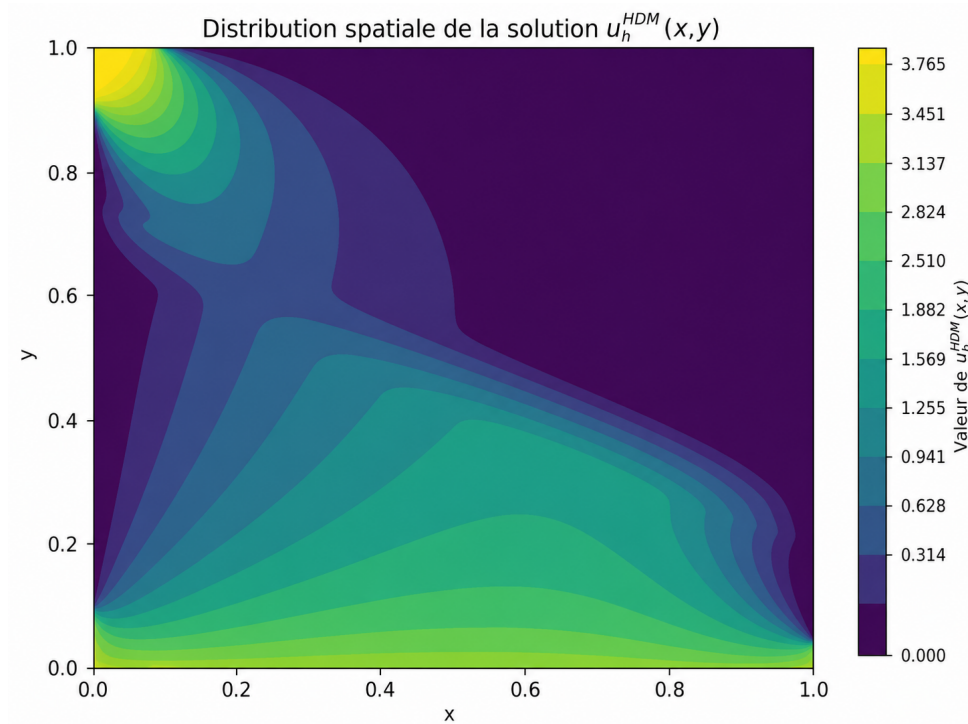
FIGURE 1 – Solution de pression du modèle haute fidélité (HDM). Champ de pression obtenu par éléments finis sur le maillage de référence.
