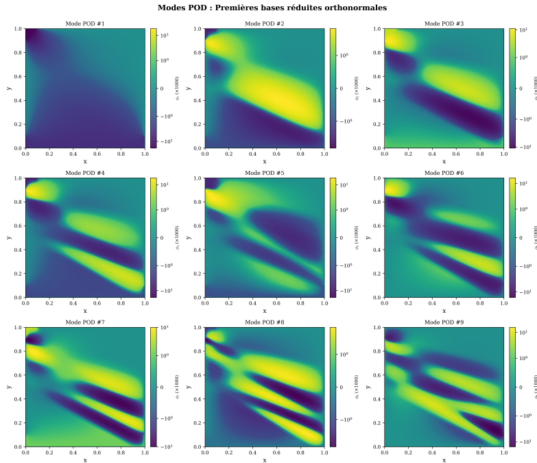
FIGURE 4 – Les 9 premiers modes POD spatiaux. Le mode 1 représente le profil de pression dominant. Les modes 2 à 9 ajoutent des détails structuraux autour de la zone de fracture paramétrée.
