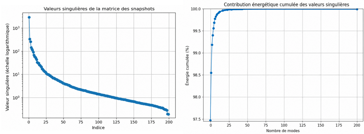
FIGURE 3 – Spectre singulier et énergie cumulée (200 snapshots). La décroissance abrupte des valeurs singulières (gauche) confirme la forte compressibilité des solutions de ce problème paramétrique.
