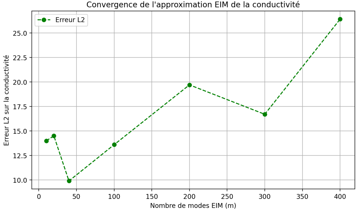
FIGURE 13 – Erreur d'approximation de l'EIM pour la conductivité k .
