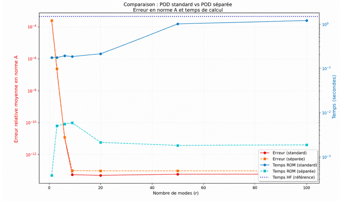
FIGURE 10 – Comparaison entre la POD standard et la POD séparée dans le cas affine. La précision reste équivalente, mais la séparation affine réduit fortement le temps de calcul online.
