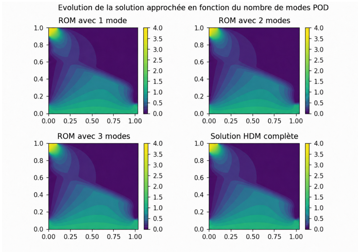
FIGURE 11 – Évolution de la solution approchée en fonction du nombre de modes POD. Quelques modes suffisent à reproduire correctement la solution haute fidélité dans le cas affine.
