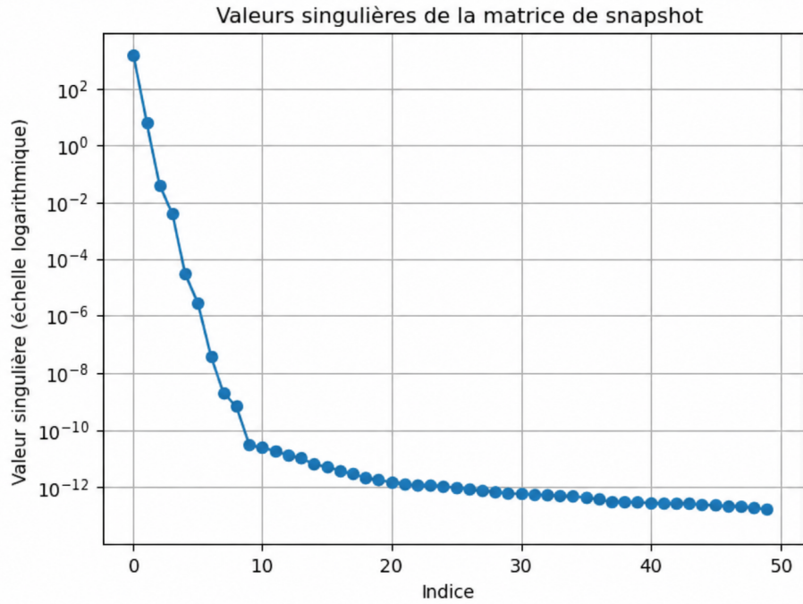
FIGURE 9 – Valeurs singulières de la matrice des snapshots dans le cas affine. La décroissance rapide du spectre montre la forte compressibilité des solutions.
