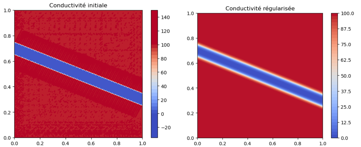
FIGURE 14 – Comparaison entre la conductivité originale k et la conductivité régularisée k_\alpha pour \alpha = 150 .
