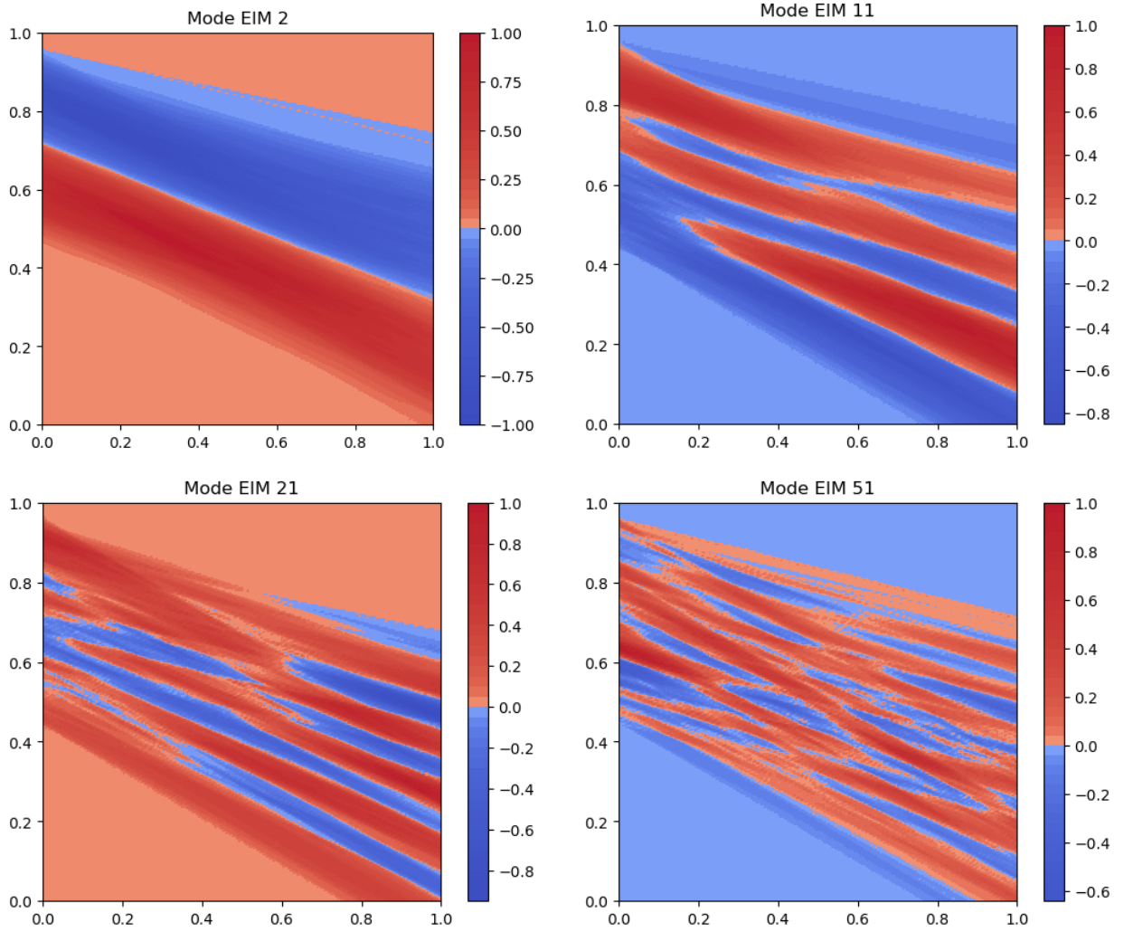
FIGURE 12 – 4 modes de la base EIM. Visualisation des modes principaux extraits par SVD (puis normalisés pour la norme L^\infty ) des snapshots de conductivité.
