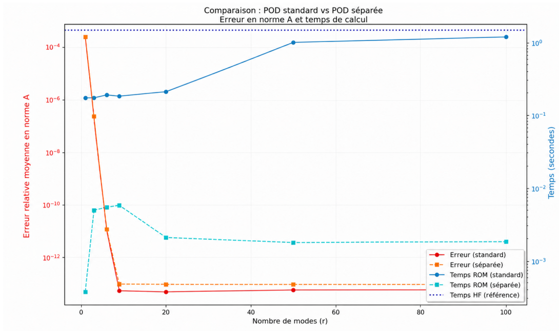
FIGURE 10 – Comparaison entre la POD standard et la POD séparée dans le cas affine. La précision reste équivalente, mais la séparation affine réduit fortement le temps de calcul online.
