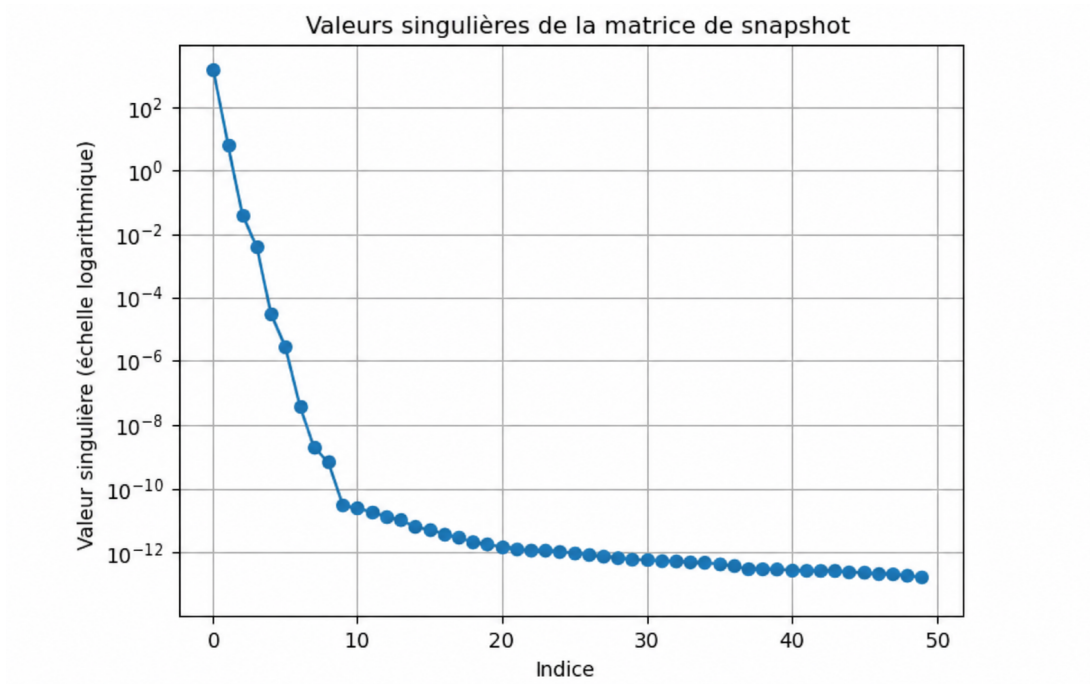
FIGURE 9 – Valeurs singulières de la matrice des snapshots dans le cas affine. La décroissance rapide du spectre montre la forte compressibilité des solutions.
