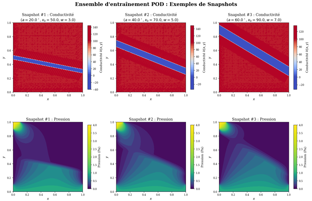
FIGURE 5 – Trois snapshots représentatifs de l'ensemble d'entraînement.
