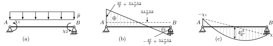
Figura 15.32. Soluzione generale (sistema principale, a): taglio T = T_0 + \chi_1 T_1 + \chi_2 T_2 (b), retta T_0 traslata della costante (\chi_1 + \chi_2)/l ; momento M = M_0 + \chi_1 M_1 + \chi_2 M_2 (c), parabola M_0 appesa alla retta di chiusura da -\chi_1 in A a \chi_2 in B . I diagrammi (b)–(c) sono tracciati per la scelta illustrativa \chi_1 = \chi_2 = \bar{p} \ell^2/12 ; i valori effettivi si ottengono imponendo la congruenza (Vol. II).
