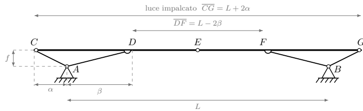
Figura 17.26. Parametri geometrici dell'arco a tre cerniere: ribassamento f , sbalzo esterno \alpha e interno \beta , luce degli appoggi L . Ne discendono \overline{CG} = L + 2\alpha e \overline{DF} = L - 2\beta ; il criterio \overline{DF} > \frac{1}{2}\overline{CG} assicura impalcato compresso sotto peso proprio.
