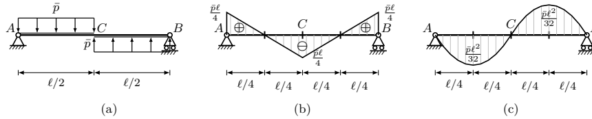
Figura 15.9. Trave appoggiata con carico distribuito emisimmetrico di intensità \bar{p} , verso il basso nel tratto AC e verso l'alto nel tratto CB (mezzera C = \ell/2 ): (a) schema strutturale; (b) diagramma del taglio T(z) , lineare a tratti e simmetrico, con valori \bar{p}\ell/4 in A , -\bar{p}\ell/4 in C e \bar{p}\ell/4 in B , e zeri in \ell/4 e 3\ell/4 ; (c) diagramma del momento flettente M(z) , parabolico a tratti ed emisimmetrico, con massimo \bar{p}\ell^2/32 in \ell/4 e minimo -\bar{p}\ell^2/32 in 3\ell/4 .
