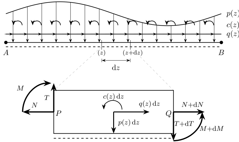
Figura 14.8. Trave con carichi distribuiti p(z) , q(z) , c(z) (in alto) e concio infinitesimo di lunghezza dz tra le sezioni P e Q (ingrandimento in basso). Le risultanti dei carichi distribuiti p(z)dz , q(z)dz , c(z)dz sono applicate al centro del concio. Sulla faccia P le caratteristiche della sollecitazione agiscono con verso negativo; sulla faccia Q con verso positivo incrementate di dN , dT , dM .
