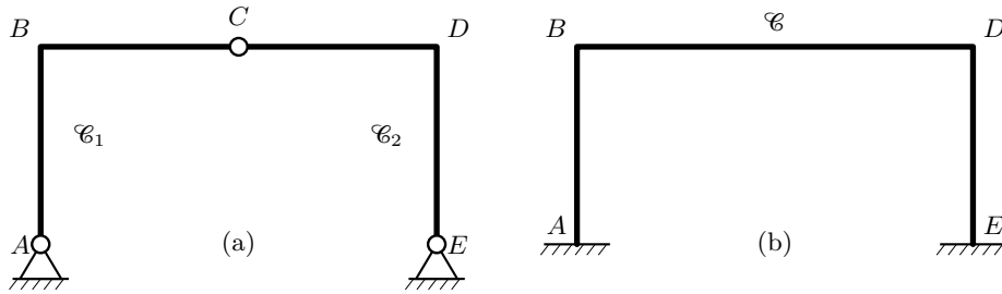
Figura 12.12. (a) Portale a tre cerniere e (b) e portale incastrato.
