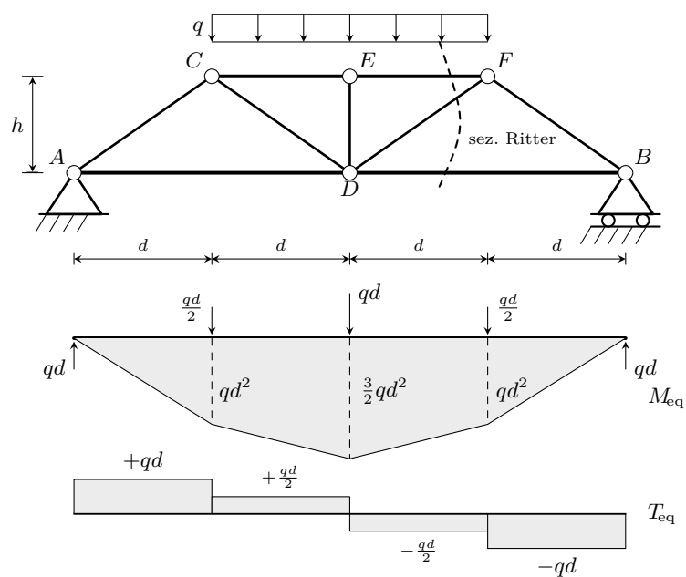
Figura 18.20. Travatura a correnti paralleli con carico distribuito sul corrente superiore. In alto: schema strutturale con sezione di Ritter tratteggiata nel pannello centrale. In basso: trave equivalente con diagrammi M_{eq} e T_{eq} .
