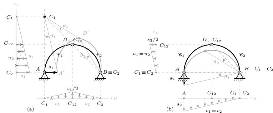
Figura 11.2. Soluzione grafica per i cedimenti esterni in A. (a) cedimento s_1 (orizzontale): tre centri distinti, C_1 all'intersezione fra la verticale per A e la retta BD. (b) cedimento s_2 (verticale): caso degenero, C_1 \equiv C_2 \equiv B , e il sistema ruota rigidamente attorno a B.
