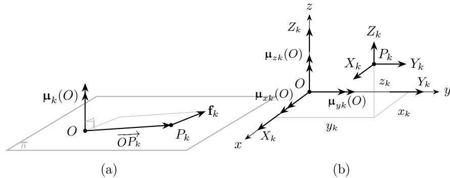
Figura 7.1. (a) Momento \boldsymbol{\mu}_k(O) rispetto al polo O della forza (P_k, \mathbf{f}_k) , definito come \boldsymbol{\mu}_k^O = \overrightarrow{OP_k} \times \mathbf{f}_k . (b) Componenti cartesiane x_k, y_k, z_k del vettore posizione \overrightarrow{OP_k} e componenti X_k, Y_k, Z_k della forza \mathbf{f}_k .
