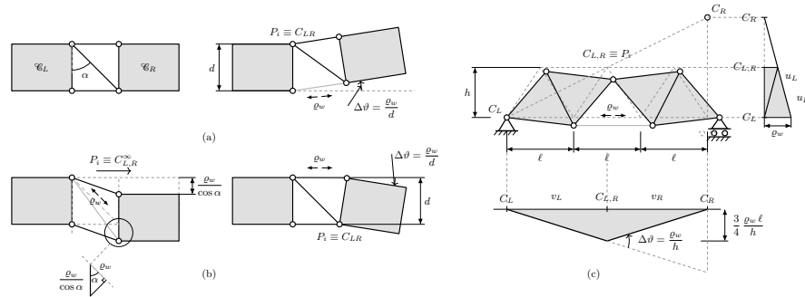
Figura 18.11. Effetto di una distorsione estensionale \varrho_w in una travatura reticolare piana. (a) caso generale, con polo proprio C \equiv P_i e rotazione relativa \Delta\vartheta = \varrho_w/d ; (b) polo improprio (a sinistra) e distorsione nel corrente superiore (a destra); (c) effetto globale su travatura vincolata: configurazione deformata, centri di rotazione C_L , C_{L,R} \equiv P_i , C_R e campi degli spostamenti verticali v^* e orizzontali u^* .
