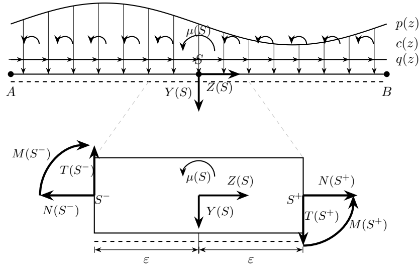
Figura 14.7. Trave con carichi distribuiti e forze concentrate Z(S) , Y(S) , \mu(S) in S (in alto). Concio di lunghezza 2\epsilon centrato in S (ingrandimento in basso): nel limite \epsilon \rightarrow 0 i carichi distribuiti scompaiono e rimangono solo le forze concentrate. L'equilibrio fornisce le equazioni di salto (14.17).
