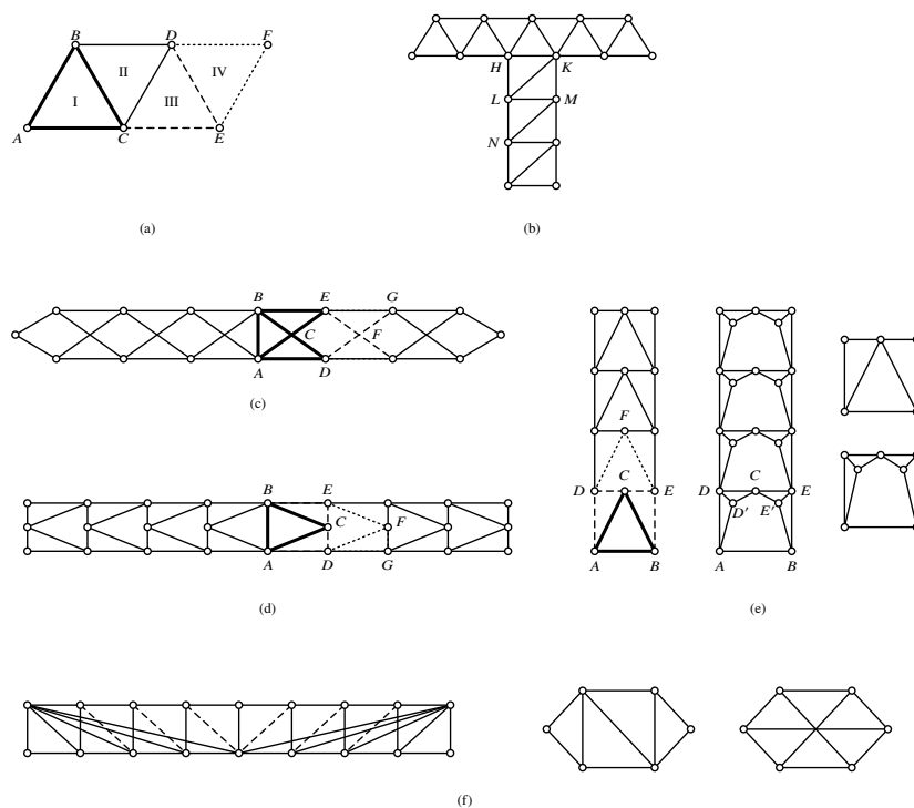
Figura 18.4: Tipologie di maglie nelle travature reticolari piane isostatiche. (a): composizione gerarchica a maglie triangolari; i nodi sono aggiunti progressivamente e le aste nuove sono tratteggiate. (b): travatura ramificata, ottenuta avviando la composizione da un'asta intermedia anziché da un nodo. (c): maglie romboidali; le diagonali si incrociano senza nodo strutturale. (d): maglie a K, con i montanti spezzati a metà altezza dal nodo su cui convergono le diagonali. (e): varianti a torre della maglia a K, con nodo sul traverso e a diagonali simmetriche; a fianco le rispettive maglie elementari. (f): schemi ibridi con aste di parete non standard: nello schema a ventaglio le aste tratteggiate sono le diagonali dello schema triangolare di partenza, soppresse e sostituite dalle aste uscenti a ventaglio dai nodi estremi del corrente superiore.
