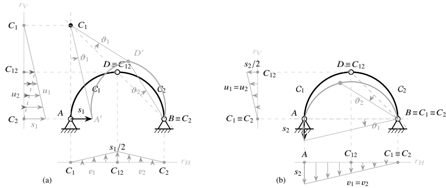
Figura 11.2: Soluzione grafica per i cedimenti esterni in A. (a) cedimento s_1 (orizzontale): tre centri distinti, C_1 all'intersezione fra la verticale per A e la retta BD . (b) cedimento s_2 (verticale): caso degenero, C_1 \equiv C_2 \equiv B , e il sistema ruota rigidamente attorno a B.
