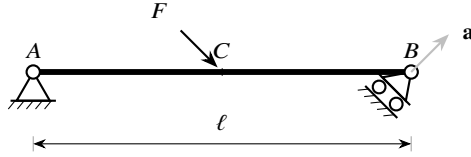
Figura 10.5: Trave appoggiata con carrello inclinato (Esempio 10.2 e Esempio 10.3): cerniera in A, carrello in B con asse \mathbf{a} a 45^\circ rispetto alla verticale, polo O \equiv A . Nel dato statico è applicata in C = (\ell/2, 0) una forza F inclinata di 45^\circ sull'orizzontale.
