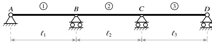
Figura 17.17: Trave continua a tre campate di luci \ell_1, \ell_2, \ell_3 ( n_e = 3, n_a = 4 ): cerniera in A , appoggi intermedi in B e C , carrello in D . Il cerchio in A e D indica il perno della connessione; il semicerchio in B e C indica che la trave scorre sull'appoggio senza interruzione della continuità rotazionale. Gradi di libertà n = 9 , vincoli m = 11 , grado di iperstaticità g = 2 pari al numero di appoggi intermedi.
