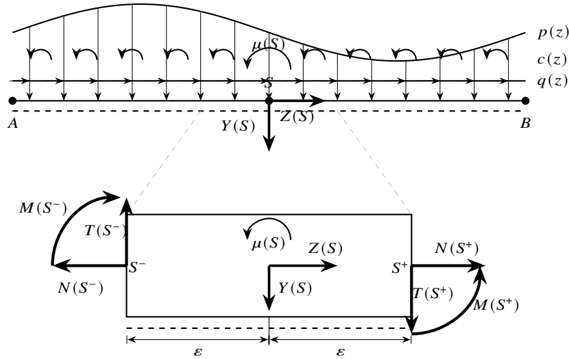
Figura 14.7: Trave con carichi distribuiti e forze concentrate Z(S), Y(S), \mu(S) in S (in alto). Concio di lunghezza 2\varepsilon centrato in S (ingrandimento in basso): nel limite \varepsilon \rightarrow 0 i carichi distribuiti scompaiono e rimangono solo le forze concentrate. L'equilibrio fornisce le equazioni di salto (14.17).
