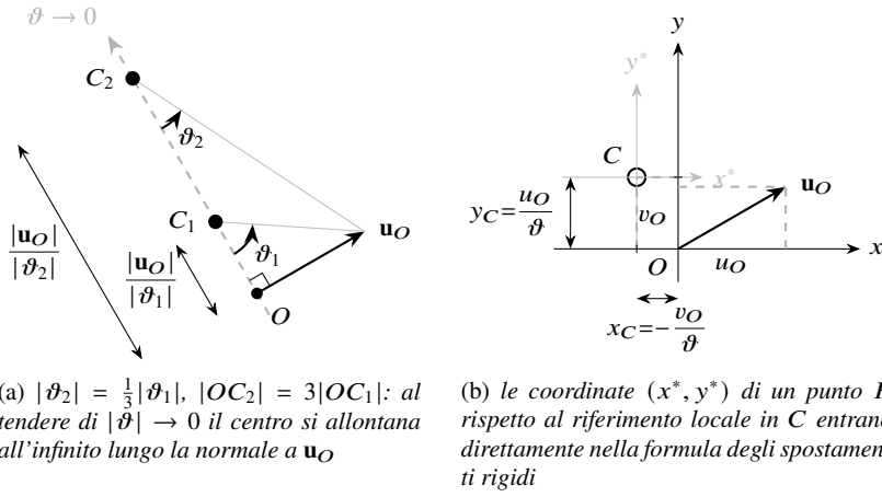
Figura 6.6: Centro di rotazione nel caso piano. (a) Costruzione geometrica: C si ottiene ruotando \mathbf{u}_O di 90^\circ nel verso di \vartheta e riscalando di 1/|\vartheta| . (b) Riferimento locale con origine in C e assi x^*, y^* paralleli a x, y : le coordinate (x^*, y^*) di un punto P entrano direttamente nella (6.38).
