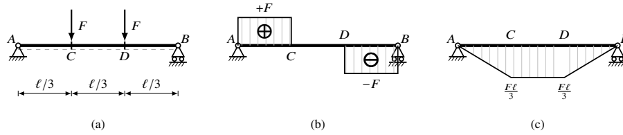
Figura 15.4: Trave appoggiata con due forze concentrate simmetriche Y(C) = Y(D) = F , C a distanza \ell/3 da A e D a distanza \ell/3 da B : (a) schema strutturale e, nel riquadro, convenzioni di segno per T (positivo orario sul concio) e M (positivo per fibre inferiori tese); (b) diagramma del taglio T(z) , uniforme a tratti ed emisimmetrico, con valori +F in AC , nullo in CD e -F in DB , e salti -F in C e in D ; (c) diagramma del momento flettente M(z) , simmetrico, lineare crescente da 0 a F\ell/3 in AC , uniforme pari a F\ell/3 in CD e lineare decrescente da F\ell/3 a 0 in DB .
