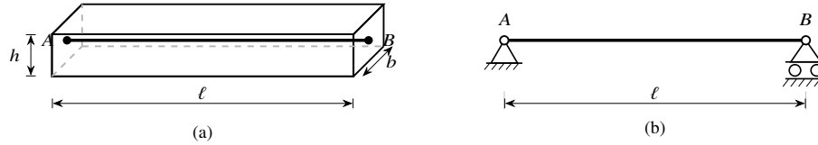
Figura 14.1: Dalla trave reale alla schematizzazione strutturale. (a) Trave reale: corpo rigido con lunghezza \ell e dimensioni trasversali b, h con b, h \ll \ell . La linea d'asse (tratteggiata spessa) è il luogo dei baricentri delle sezioni trasversali; gli estremi A e B sono i punti della linea d'asse corrispondenti alle facce terminali. (b) Schematizzazione strutturale: si traccia la sola linea d'asse; i vincoli (cerniera in A , carrello in B ) sono posizionati sui punti corrispondenti. Questa è la rappresentazione adottata in tutte le figure del capitolo.
