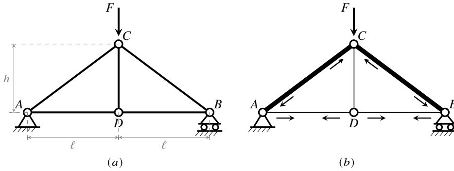
Figura 18.14: Capriata triangolare con carico al colmo. (a): schema strutturale con denominazione dei nodi. (b): stato di sollecitazione qualitativo. Tratto spesso: aste compresse AC e CB (puntoni); le frecce mostrano la compressione interna, con le estremità spinte verso l'esterno. Tratto sottile: aste tese AD e DB (tiranti); le frecce mostrano la trazione interna, con le estremità tirate verso il centro. In grigio il monaco CD : sforzo nullo per simmetria con carico al colmo.
