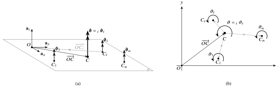
Figura 6.7: Composizione di n rotazioni infinitesime nel piano. (a) Vista tridimensionale: le rotazioni sono vettori assiali \boldsymbol{\vartheta}_i ortogonali al piano \pi , che si sommano nella risultante \boldsymbol{\vartheta} = \sum \boldsymbol{\vartheta}_i in C . (b) Vista nel piano (x, y) : ampiezze \vartheta_i come archi orientati (positivi se antiorari) e centro risultante C nel baricentro dei C_i . Il centro C è individuato da \overrightarrow{OC} = (\sum \vartheta_i \overrightarrow{OC_i}) / \vartheta o, in forma equivalente, da \sum \vartheta_i \overrightarrow{CC_i} = \mathbf{0} (freccie grigie in (b)).
