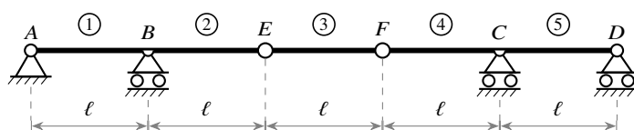
Figura 17.14: Trave di Gerber su quattro appoggi ( n_a = 4 , n_e = 5 ) con due cerniere interne ( n_c = 2 ) in E e F , collocate a \ell dagli appoggi B e C . Gradi di libertà n = 15 , vincoli m = 15 , sistema isostatico ( \nu = 0 ).
