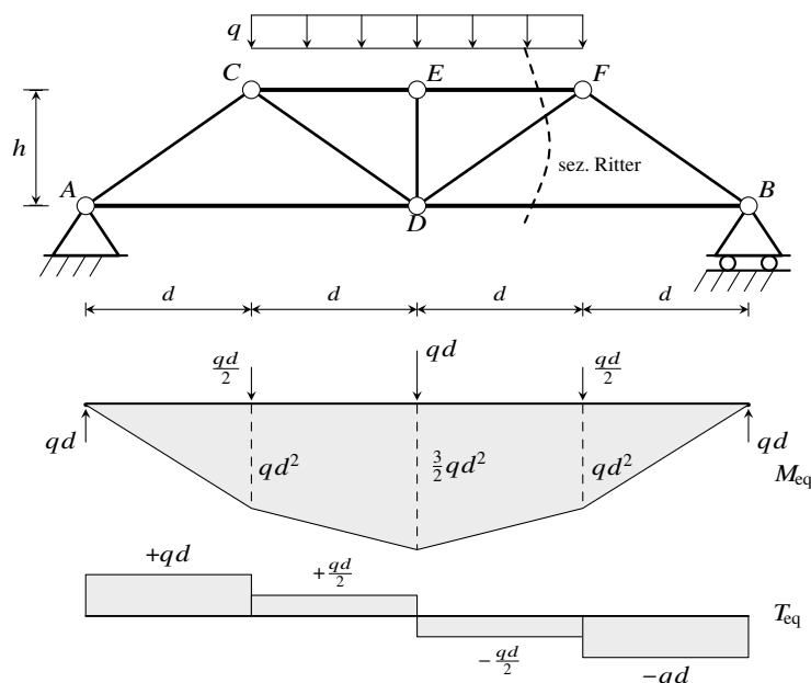
Figura 18.20: Travatura a correnti parallele con carico distribuito sul corrente superiore. In alto: schema strutturale con sezione di Ritter tratteggiata nel pannello centrale. In basso: trave equivalente con diagrammi M_{eq} e T_{eq} .
