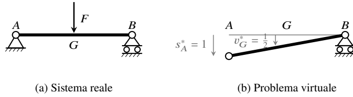
Figura 20.1: TSV per il calcolo della reazione R_A in una trave semplicemente appoggiata sotto carico F in mezzzeria.
