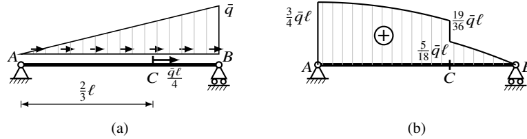
Figura 15.2: Trave con carico longitudinale triangolare q(z) = \bar{q}z/\ell e forza concentrata Z(C) = \bar{q}\ell/4 in C: (a) schema strutturale; (b) diagramma dello sforzo normale N(z) , parabolico in entrambi i tratti, con un salto -\bar{q}\ell/4 in C.
