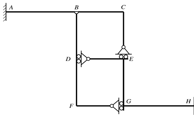
Figura 12.10: Struttura mista: due mensole ad asse spezzato S_1 = ABCE (incastrata in A) e S_2 = HGED (incastrata in H), collegate da una trave appoggiata S_3 = BDFG (cerniera in B, carrello in G). I carrelli in D ed E aggiungono due vincoli semplici allo schema isostatico di riferimento: v = -2 , iperstatica di grado 2.
