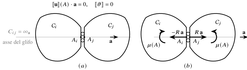
Figura 9.9: Glifo interno fra i corpi C_i e C_j con asse \mathbf{a} . Prestazione cinematica (a): le equazioni di vincolo [\mathbf{u}](A) \cdot \mathbf{a} = 0 e [\vartheta] = 0 impongono l'uguaglianza delle componenti di spostamento dei due corpi lungo \mathbf{a} e l'uguaglianza delle rotazioni \vartheta_i e \vartheta_j ; lo scorrimento relativo lungo \mathbf{a}^\perp resta libero. Il centro di rotazione relativo è all'infinito sulla retta dell'asse, C_{ij} = \infty_{\mathbf{a}} . Prestazione statica (b): i due corpi si scambiano una forza R \mathbf{a} diretta lungo l'asse e una coppia \mu(A) , uguali e opposte, in dualità rispettivamente con la componente di spostamento relativo lungo \mathbf{a} e con la rotazione relativa bloccate, in accordo con la molteplicità due.
