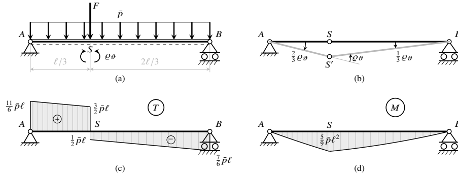
Figura 14.9: Trave appoggiata AB con distorsione rotazionale \varrho_\theta > 0 in S = \ell/3 , carico distribuito uniforme p_0 e forza concentrata F = 2\bar{p}\ell in S . (a) Schema con geometria, vincoli, carichi e distorsione. (b) Configurazione deformata prodotta dalla sola distorsione \varrho_\theta : i carichi non modificano la cinematica del corpo rigido. (c) Diagramma del taglio T(z) : lineare a tratti, con salto -F in S . (d) Diagramma del momento flettente M(z) : parabolico a tratti, continuo in S , nullo agli estremi. La distorsione non contribuisce ai diagrammi (c) e (d): in un sistema isostatico le distorsioni producono spostamenti ma non sollecitazioni (Oss. ??).
