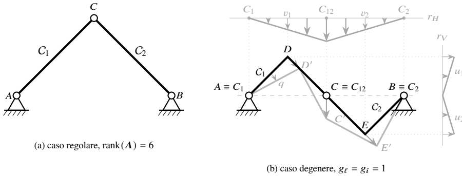
Figura 12.8: Arco a tre cerniere: (a) caso regolare, portale con A, C, B non collineari ( \text{rank}(A) = 6 , isostatico); (b) caso degenere, struttura poligonale con A, C, B collineari ( g_\ell = g = 1 ), meccanismo parametrizzato da q e rette di proiezione r_H, r_V .
