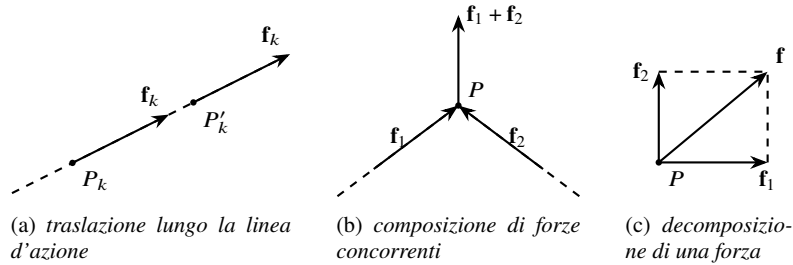
Figura 7.5: Operazioni elementari di equivalenza (I). (a) Traslazione della forza \mathbf{f}_k lungo la propria linea d'azione da P_k a P'_k : risultante e momento risultante restano invariati. (b) Composizione di due forze concorrenti in P : il sistema è equivalente alla risultante \mathbf{f}_1 + \mathbf{f}_2 applicata in P . (c) Decomposizione della forza \mathbf{f} applicata in P nelle componenti \mathbf{f}_1 e \mathbf{f}_2 secondo due direzioni indipendenti: operazione inversa alla composizione.
