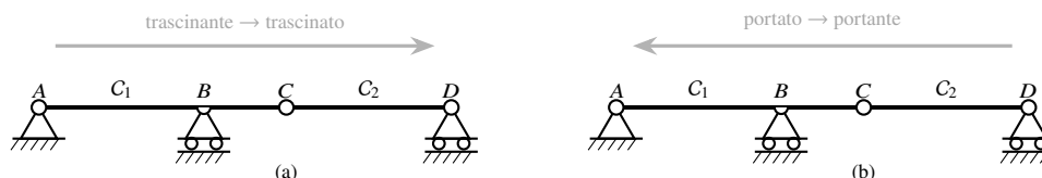
Figura 11.13: Gerarchia strutturale della trave di Gerber: (a) cascata cinematica, dal trascinante C_1 al trascinato C_2 (freccia da sinistra a destra); (b) cascata statica, dal portato C_2 al portante C_1 (freccia da destra a sinistra). Le due cascate percorrono la stessa gerarchia in direzioni opposte.
