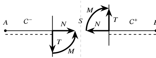
Figura 14.4: Caratteristiche della sollecitazione nella sezione S : sulla faccia destra di C^- (normale uscente +z^e ) agiscono N , T , M nel verso positivo convenuto; sulla faccia sinistra di C^+ le stesse grandezze agiscono con verso opposto per il terzo principio.
