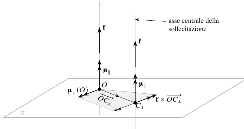
Figura 7.4: Costruzione geometrica dell'asse centrale del sistema di forze. Il momento rispetto a O si scompone nella componente \mathbf{m}_\parallel^O , parallela a \mathbf{f} e invariante per tutti i poli, e nella componente \mathbf{m}_\perp^O , giacente nel piano \pi ortogonale a \mathbf{f} . Il punto C_\perp , intersezione dell'asse centrale con \pi , è determinato dalla condizione \mathbf{f} \times \overrightarrow{OC}_\perp = -\mathbf{m}_\perp^O ; l'asse centrale è la retta per C_\perp parallela a \mathbf{f} .
