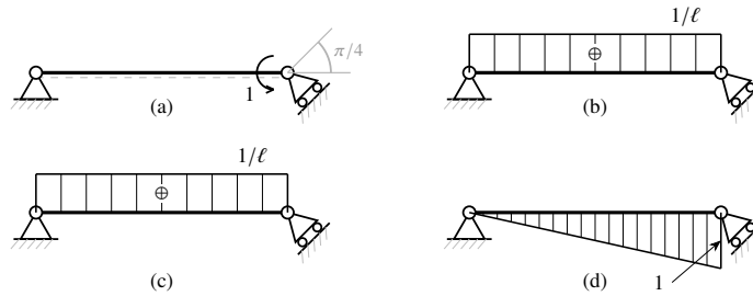
Figura 15.36: Problema “2”: coppia unitaria in B (a); sforzo normale N_2 (b); taglio T_2 (c); momento flettente M_2 (d).
