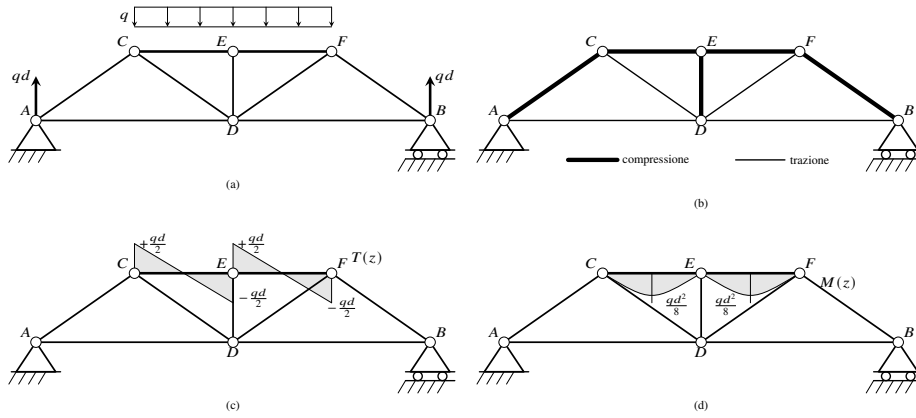
Figura 18.21: Travatura a correnti parallele con carico distribuito q su CE ed EF . (a): schema di carico. (b): funzionamento strutturale — aste compresse a tratto spesso, aste tese a tratto sottile. (c): diagramma del taglio T(z) sulle aste CE ed EF . (d): diagramma del momento M(z) sulle aste CE ed EF .
