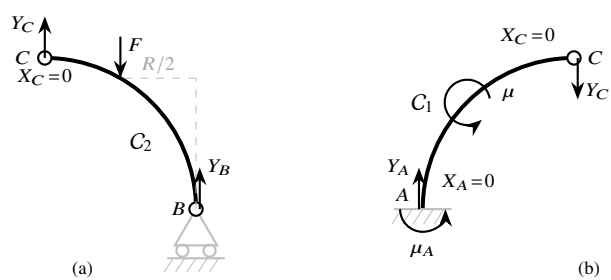
Figura 11.16: Arco a tutto sesto con incastro: schemi dei corpi liberi di C_2 (a) e C_1 (b). La cascata statica procede da C_2 a C_1 , in ordine inverso rispetto alla cinematica; polo di momento in C per C_2 , in A per C_1 .
