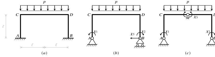
Figura 19.4: Portale doppiamente incastrato: schema iperstatico e due scelte del sistema principale. (a) Schema originale, grado di iperstaticità g_i = 3 ( g^{\text{est}} = 3 , g^{\text{int}} = 0 ): colonne incastrate in A e B, traverso CD con carico uniforme p . (b) Sistema principale “portale appoggiato”: gli incastrati sono sostituiti da una cerniera in A e da un carrello a reazione verticale in B; le incognite iperstatiche sono la coppia \chi_1 (momento rimosso in A, antioraria), la coppia \chi_2 (momento rimosso in B, oraria) e la forza orizzontale \chi_3 (reazione orizzontale rimossa in B, diretta verso A). (c) Sistema principale “portale a tre cerniere”: gli incastrati sono sostituiti da cerniere esterne in A e B; una cerniera interna in M (mezzeria del traverso) rilascia la continuità del momento flettente; le incognite iperstatiche sono la coppia \chi_1 in A, la coppia \chi_2 in B e la coppia \chi_3 in M.
