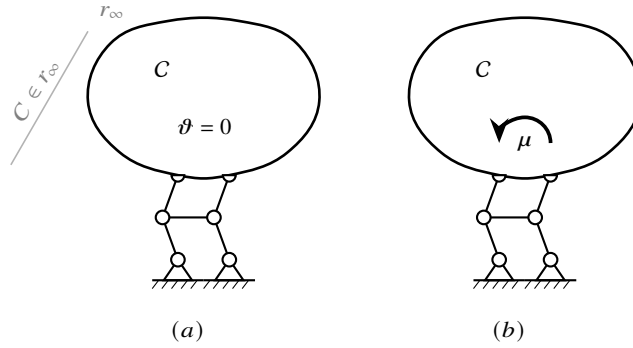
Figura 9.4: Bipendolo esterno applicato al corpo C , realizzato meccanicamente come pantografo a doppio parallelogramma. Prestazione cinematica (a): l'equazione di vincolo \vartheta = 0 annulla la rotazione del corpo, lasciando libere le due componenti di traslazione, non rappresentate; il centro di rotazione assoluto giace sulla retta impropria r_\infty . Prestazione statica (b): la reazione vincolare si riduce alla sola coppia \mu , in dualità con la rotazione bloccata; la forza risultante è identicamente nulla, in accordo con la molteplicità uno.
