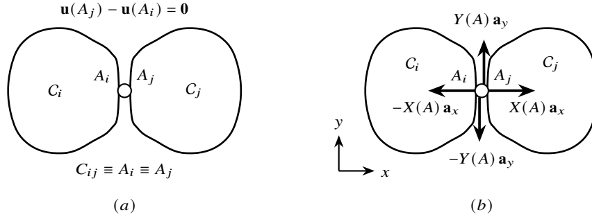
Figura 9.7: Cerniera interna fra i corpi C_i e C_j , applicata nel punto A che si identifica con i punti di applicazione A_i \in C_i e A_j \in C_j . Prestazione cinematica (a): l'equazione di vincolo \mathbf{u}(A_j) - \mathbf{u}(A_i) = \mathbf{0} impone l'uguaglianza degli spostamenti dei due corpi in A ; le rotazioni dei due corpi restano libere e non sono rappresentate. Il centro di rotazione relativo coincide con il punto di applicazione, C_{ij} \equiv A_i \equiv A_j . Prestazione statica (b): i due corpi si scambiano una forza generica X(A)\mathbf{a}_x + Y(A)\mathbf{a}_y applicata in A , in dualità con le due componenti di spostamento relativo bloccate; la coppia scambiata è identicamente nulla, in accordo con la molteplicità due.
