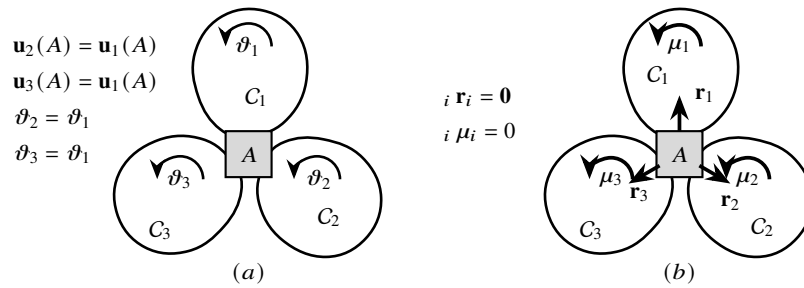
Figura 9.13: Incastro multiplo fra i corpi C_1, C_2, C_3 nel punto A . Prestazione cinematica (a): le equazioni di vincolo \mathbf{u}_2(A) = \mathbf{u}_1(A) , \mathbf{u}_3(A) = \mathbf{u}_1(A) , \vartheta_2 = \vartheta_1 , \vartheta_3 = \vartheta_1 impongono l'uguaglianza degli spostamenti e delle rotazioni dei tre corpi in A ; i tre corpi si comportano come un unico corpo rigido nel nodo. Prestazione statica (b): i tre corpi si scambiano in A forze \mathbf{r}_1, \mathbf{r}_2, \mathbf{r}_3 e coppie \mu_1, \mu_2, \mu_3 di direzione e verso arbitrari, soggette all'equilibrio del nodo \sum_i \mathbf{r}_i = \mathbf{0} e \sum_i \mu_i = 0 . Le incognite indipendenti sono le componenti delle coppie e delle forze relative a C_2 e C_3 (per un totale di 3(k - 1) = 6 ), in accordo con la molteplicità.
