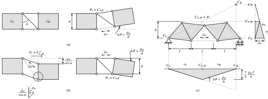
Figura 18.11: Effetto di una distorsione estensionale \varrho_w in una travatura reticolare piana. (a) caso generale, con polo proprio C \equiv P_i e rotazione relativa \Delta\theta = \varrho_w/d ; (b) polo improprio (a sinistra) e distorsione nel corrente superiore (a destra); (c) effetto globale su travatura vincolata: configurazione deformata, centri di rotazione C_L , C_{L,R} \equiv P_i , C_R e campi degli spostamenti verticali v^* e orizzontali u^* .
