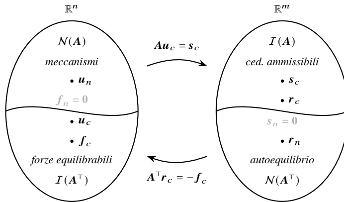
Figura 10.2: Struttura duale dei problemi cinematico Au = s e statico A^\top r = -f . Il problema cinematico ammette soluzione se e solo se s_c \in \mathcal{I}(A) , cioè s_n = 0 : il cedimento deve essere cinematicamente ammissibile. Il problema statico ammette soluzione se e solo se f_c \in \mathcal{I}(A^\top) , cioè f_n = 0 : la forza attiva deve essere equilibrabile dai vincoli. Le soluzioni generali sono u = u_c + u_n con u_n \in \mathcal{N}(A) (meccanismo) arbitrario, e r = r_c + r_n con r_n \in \mathcal{N}(A^\top) (stato di autoequilibrio) arbitrario.
