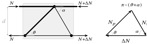
Figura 18.18: Maglia elementare del traliccio di Ritter-Mörsch e poligono delle forze al nodo del corrente superiore. Pannello sinistro : la variazione di sforzo \Delta N nei correnti — uguale in valore assoluto nel corrente superiore compresso e in quello inferiore teso — deve essere equilibrata dalle componenti orizzontali del puntone (tratto spesso, angolo \vartheta ) e della staffa (tratto sottile, angolo \alpha ). Pannello destro : poligono chiuso delle forze al nodo; l'angolo al vertice opposto a \Delta N vale \pi - (\vartheta + \alpha) , donde per il teorema dei seni le (18.22).
