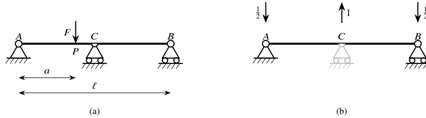
Figura 11.9: Trave iperstatica di grado 1 (Esempio 11.6): (a) sistema originale con carico F in P ; (b) sistema principale (carrello in C in grigio) e stato di autoequilibrio \mathbf{r}_1 : reazione unitaria verso l'alto in C , reazioni 1/2 verso il basso in A e B .
