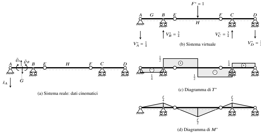
Figura 20.5: Trave di Gerber: applicazione del TFCV per il calcolo dello spostamento \eta_H in mezzeria della travata portata EF , sotto cedimento \bar{s}_A in A e distorsioni \bar{q}_v , \bar{q}_\theta in G.
