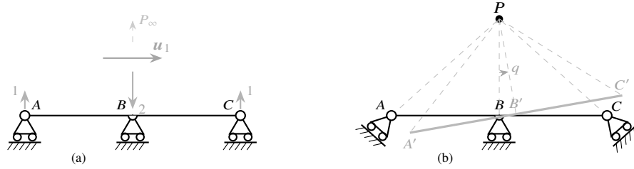
Figura 12.7: Degenerazione geometrica per un singolo corpo ( \nu = 0 , g_\ell = g = 1 ): (a) tre carrelli verticali paralleli — stato di autoequilibrio con reazioni (1, -2, 1) (freccie grigie) e meccanismo di traslazione orizzontale u_1 ; (b) tre carrelli con assi convergenti nel punto proprio P — meccanismo di rotazione attorno a P e linee d'azione dei vincoli (tratteggiate).
