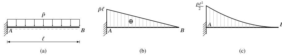
Figura 15.7: Mensola con carico uniformemente distribuito p(z) = \bar{p} (verso il basso), incastrata in A e libera in B : (a) schema strutturale; (b) diagramma del taglio T(z) , lineare decrescente, con valore \bar{p}\ell all'incastro e annullamento all'estremità libera; (c) diagramma del momento flettente M(z) , parabolico con concavità verso l'alto, sempre negativo, con valore minimo -\bar{p}\ell^2/2 all'incastro e annullamento all'estremità libera, dove il diagramma arriva con tangente orizzontale.
