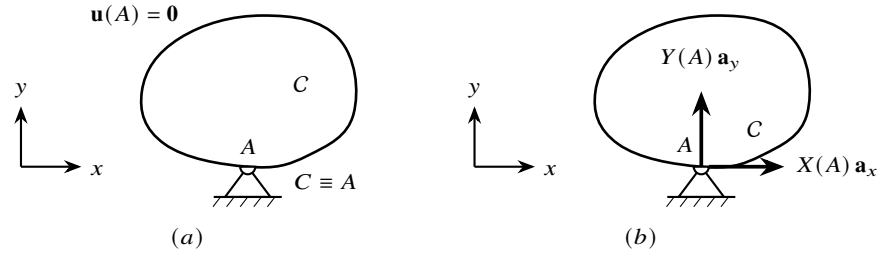
Figura 9.6: Cerniera esterna applicata al corpo C nel punto A . Prestazione cinematica (a): il punto A è fisso, \mathbf{u}(A) = \mathbf{0} , e il corpo ruota liberamente attorno ad esso; il centro di rotazione assoluto coincide con il punto di applicazione, C \equiv A . Prestazione statica (b): la reazione vincolare è una forza generica X(A) \mathbf{a}_x + Y(A) \mathbf{a}_y applicata in A , in dualità con le due componenti di spostamento bloccate; la coppia reattiva è identicamente nulla, in accordo con la molteplicità due.
