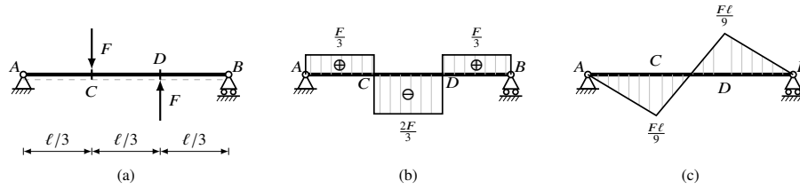
Figura 15.5: Trave appoggiata con forze concentrate emisimmetriche Y(C) = F in C e Y(D) = -F in D, C a distanza \ell/3 da A e D a distanza \ell/3 da B: (a) schema strutturale; (b) diagramma del taglio T(z) , uniforme a tratti e simmetrico, con valori F/3 in AC, -2F/3 in CD e F/3 in DB, e salti -F in C e +F in D; (c) diagramma del momento flettente M(z) , lineare a tratti ed emisimmetrico, con massimo F\ell/9 in C, annullamento in mezzeria e minimo -F\ell/9 in D.
