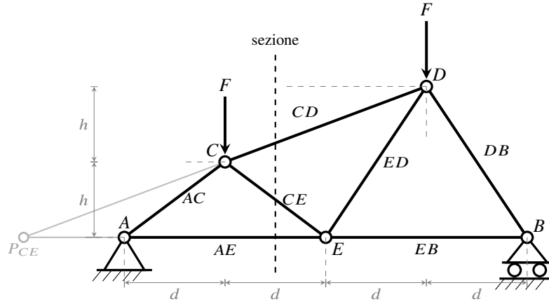
Figura 18.15: Capriata a correnti non parallele. Schema strutturale con la sezione canonica di Ritter (linea tratteggiata verticale) che taglia le aste CD , AE e CE . I prolungamenti in grigio delle rette d'azione di CD e AE si incontrano nel polo P_{CE} = (-d, 0) , esterno alla struttura. I poli P_{CD} \equiv E e P_{AE} \equiv C coincidono con nodi della travatura.
