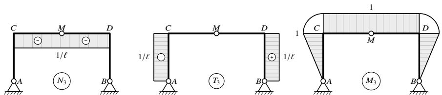
Figura 19.9: Autosoluzione 3 ( \chi_3 = 1 , coppia unitaria in M): diagrammi di N_3 , T_3 e M_3 sul portale a tre cerniere. Gli archetti in C e D indicano la continuità del momento flettente ai due nodi rigidi.
