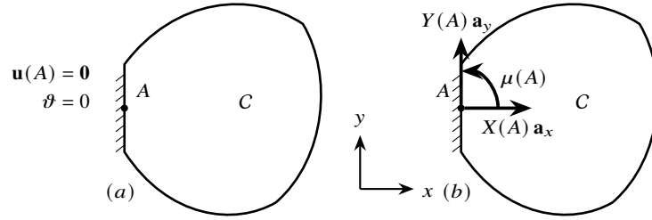
Figura 9.10: Incastro applicato al corpo C nel punto A . Prestazione cinematica (a): nessuno spostamento è ammesso, né traslazione né rotazione ( \mathbf{u}(A) = \mathbf{0} , \vartheta = 0 ); il corpo è completamente bloccato. Prestazione statica (b): la reazione vincolare è una forza generica X(A) \mathbf{a}_x + Y(A) \mathbf{a}_y e una coppia \mu(A) , applicate in A , in accordo con la molteplicità tre.
