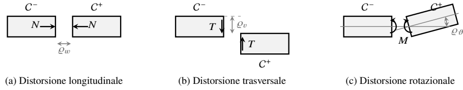
Figura 14.5: Distorsioni di concio e caratteristiche della sollecitazione duale: la coppia (\sigma, \varrho) entra nell'identità bilineare con segno discorde.
