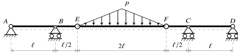
Figura 17.15: Trave di Gerber su quattro appoggi ( n_a = 4 , n_e = 5 , n_c = 2 ): cerniera in A , appoggi continui in B e C , carrello in D , cerniere interne in E e F . Luci: AB = CD = \ell , BE = FC = \ell/2 , EF = 2\ell . La campata portata EF è soggetta a un carico trasversale triangolare di intensità massima p nella sezione di mezzeria e nulla agli estremi E e F .
