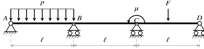
Figura 17.18: Trave continua a tre campate di uguale luce \ell : carico uniformemente distribuito p sul tratto AB , coppia concentrata \mu nella sezione C , forza concentrata F a mezziera del tratto CD . Il cerchio in A e D indica il perno; il semicerchio in B e C indica che la trave scorre sull'appoggio senza interruzione della continuità rotazionale.
