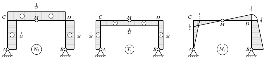
Figura 19.8: Autosoluzione 2 ( \chi_2 = 1 , coppia unitaria in B): diagrammi di N_2 , T_2 e M_2 sul portale a tre cerniere. Gli archetti in C e D indicano la continuità del momento flettente ai due nodi rigidi.
