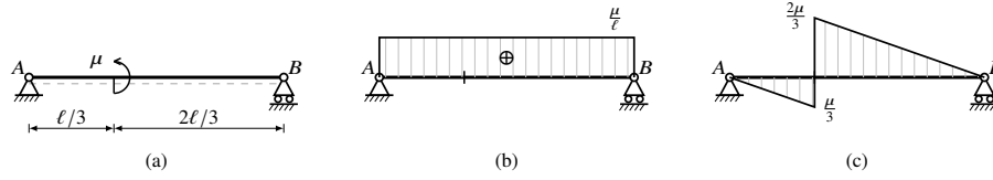
Figura 15.12: Trave appoggiata con coppia concentrata antioraria \mu applicata in C a distanza \ell/3 da A: (a) schema strutturale; (b) diagramma del taglio T(z) , uniforme pari a \mu/\ell su tutta la trave (la coppia concentrata non produce salto del taglio); (c) diagramma del momento flettente M(z) , lineare crescente a tratti, da 0 a \mu/3 in AC e da -2\mu/3 a 0 in CB, con salto -\mu in C.
