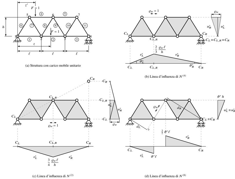
Figura 20.4: Travatura reticolare piana a correnti paralleli: linee d'influenza degli sforzi normali nelle aste 4 (corrente superiore), 2 (corrente inferiore) e 8 (diagonale), sotto carico unitario verticale mobile sui nodi dei due correnti. (a) Geometria della travatura, con luce totale 3\ell e altezza h fra i correnti. (b), (c), (d) Meccanismi virtuali duali (TSV) ottenuti imponendo una distorsione longitudinale q_w sull'asta in esame; il campo v^* sotto la travatura fornisce le ordinate della linea d'influenza per carichi verticali, il campo u^* a fianco le ordinate per carichi orizzontali.
