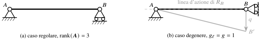
Figura 12.5: Trave appoggiata: (a) caso regolare, \text{rank}(A) = 3 (isostatico); (b) caso degenere, g_\ell = g = 1 . In (b) la linea d'azione del carrello (tratteggio grigio) coincide con la retta AB ; il meccanismo è rappresentato dalla configurazione deformata (grigio) e dal parametro lagrangiano q .
