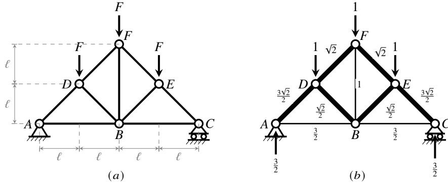
Figura 18.13: Capriata palladiana con carichi simmetrici. (a): schema strutturale con denominazione dei nodi (ogni asta è individuata dalla coppia dei nodi di estremità). (b): stato di sollecitazione, con i valori delle forze — carichi, reazioni e sforzi normali — al netto del fattore F . Tratto spesso: aste compresse — le falde AD , DF , CE , FE e le saette DB , EB (puntoni). Tratto sottile: aste tese — la catena AB , BC e il monaco BF (tiranti). Sotto gli appoggi le due reazioni verticali \frac{3}{2}F .
