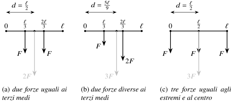
Figura 7.8: Sistemi di forze concentrate -F_k \mathbf{a}_y equiorientate su un intervallo di lunghezza \ell : la risultante (in grigio) è applicata nel baricentro dei punti di applicazione pesati con le rispettive intensità. (a) |\mathbf{f}| = 2F , d = \ell/2 . (b) |\mathbf{f}| = 3F , d = 5\ell/9 . (c) |\mathbf{f}| = 3F , d = \ell/2 .
