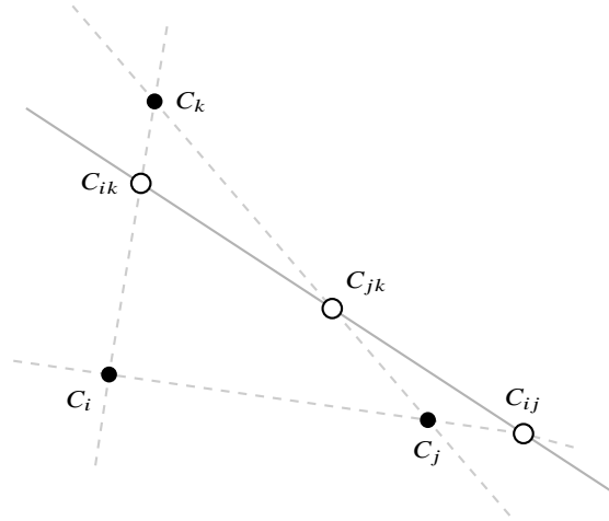
Figura 6.11: Teorema di allineamento dei centri di rotazione relativi. I tre corpi C_i, C_j, C_k hanno centri assoluti C_i, C_j, C_k (cerchi pieni). I centri di rotazione relativi C_{ij}, C_{ik}, C_{jk} — ciascuno punto di uguale spostamento per la coppia di corpi corrispondente — sono allineati (cerchi vuoti, retta grigia). Il centro C_{ij} cade all'esterno del segmento C_i C_j , coerentemente con il teorema di Menelao.
