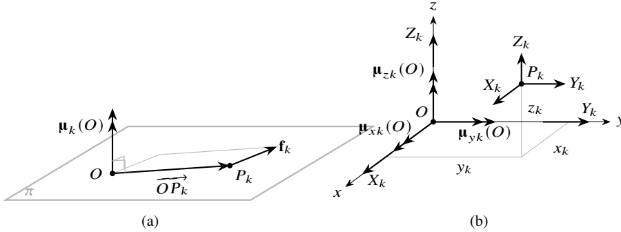
Figura 7.1: (a) Momento \mu_k(O) rispetto al polo O della forza (P_k, \mathbf{f}_k) , definito come \mu_k^O = \overrightarrow{OP_k} \times \mathbf{f}_k . (b) Componenti cartesiane x_k, y_k, z_k del vettore posizione \overrightarrow{OP_k} e componenti X_k, Y_k, Z_k della forza \mathbf{f}_k .
