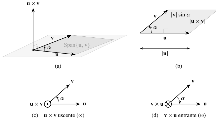
Figura 5.4: Rappresentazione geometrica del prodotto vettoriale \mathbf{u} \times \mathbf{v} . In (a) il vettore \mathbf{u} \times \mathbf{v} è ortogonale al piano \text{Span}\{\mathbf{u}, \mathbf{v}\} e orientato secondo la regola della mano destra; il suo modulo eguaglia l'area del parallelogramma costruito su \mathbf{u} e \mathbf{v} . In (b) tale area è letta come prodotto della base |\mathbf{u}| per l'altezza |\mathbf{v}| \sin \alpha , da cui |\mathbf{u} \times \mathbf{v}| = |\mathbf{u}| |\mathbf{v}| \sin \alpha . In (c) e (d) è illustrata l'antisimmetria \mathbf{u} \times \mathbf{v} = -(\mathbf{v} \times \mathbf{u}) : a parità di \mathbf{u} , \mathbf{v} e di angolo \alpha , il prodotto cambia verso — uscente dal piano ( \odot ) per \mathbf{u} \times \mathbf{v} , entrante ( \otimes ) per \mathbf{v} \times \mathbf{u} — coerentemente col senso di rotazione che porta il primo fattore sul secondo.
