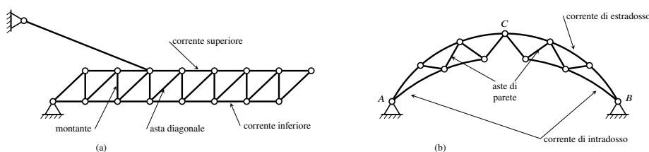
Figura 18.3: Parti della travatura reticolare piana. (a): travatura a correnti paralleli (mensola con tirante ancorato a parete); si distinguono il corrente superiore (o di estradosso), il corrente inferiore (o di intradosso) e le aste di parete, suddivise in montanti e diagonali. (b): arco reticolare a tre cerniere ( A , C , B ) a correnti curve; le stesse denominazioni si applicano con riferimento al corrente di estradosso e al corrente di intradosso, entrambi curvilinei, raccordati dalle aste di parete; il corrente di intradosso è interrotto alla chiave, dove il nodo C funge da cerniera tra i due semiarchi.
