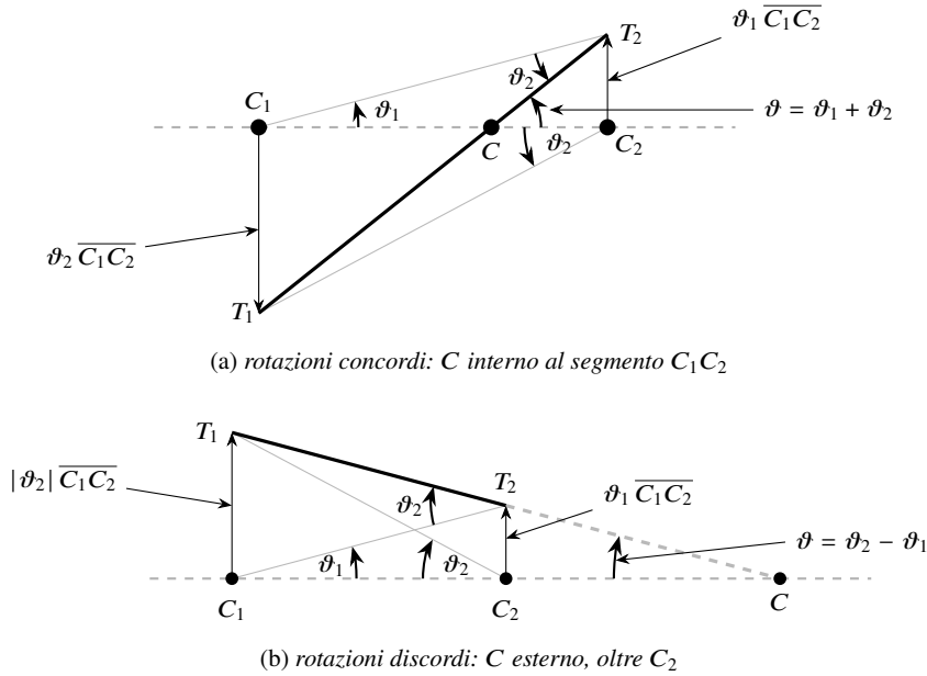
Figura 6.8: Composizione di due rotazioni infinitesime nel piano come diagramma degli spostamenti trasversali alla congiungente C_1C_2 : la retta spessa è v(x) = \vartheta_1 (x - x_{C_1}) + \vartheta_2 (x - x_{C_2}) e il centro risultante C è il suo zero, con \vartheta \overline{CC_1} = |\vartheta_2| \overline{C_1C_2} . (a) Concordi: C interno a C_1C_2 . (b) Discordi ( |\vartheta_2| > \vartheta_1 ): C esterno, oltre C_2 .
