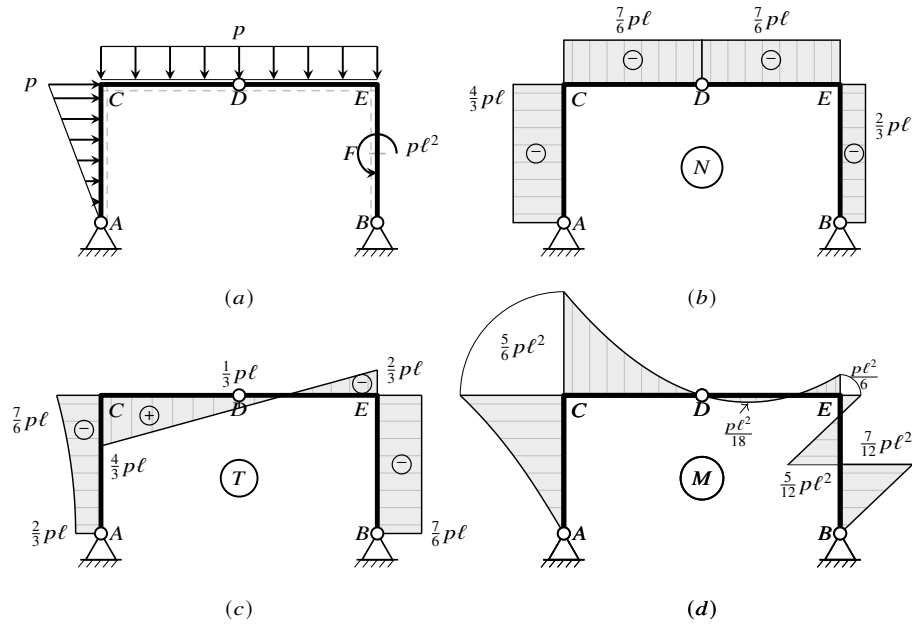
Figura 17.7: Arco a tre cerniere: (a) schema strutturale con fibre inferiori (tratteggio); (b) sforzo normale N (compressione in tutti i tratti); (c) taglio T : positivo verso la fibra inferiore; (d) momento flettente M : positivo verso la fibra inferiore. Il massimo momento positivo su DE , pari a p\ell^2/18 nel punto a \ell/3 da D , è di piccola entità rispetto agli altri valori e risulta appena visibile in scala.
