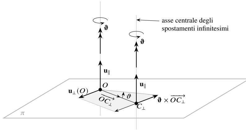
Figura 6.5: Costruzione geometrica dell'asse centrale degli spostamenti rigidi infinitesimi. Lo spostamento di O si scompone nella componente \mathbf{u}_\parallel , parallela a \mathfrak{D} e invariante per tutti i punti del corpo, e nella componente \mathbf{u}_\perp(O) , giacente nel piano \pi ortogonale a \mathfrak{D} . Il punto C_\perp , intersezione dell'asse centrale con \pi , è determinato dalla condizione \mathfrak{D} \times \overrightarrow{OC_\perp} = -\mathbf{u}_\perp(O) ; l'asse centrale è la retta per C_\perp parallela a \mathfrak{D} .
