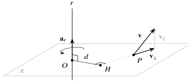
Figura 5.11: Riduzione al piano del momento assiale: per la doppia invarianza si sceglie il piano \pi per P ortogonale a r e, come polo, l'intersezione O = r \cap \pi . Decomposto \mathbf{v} = \mathbf{v}_{\parallel} + \mathbf{v}_{\perp} , la componente parallela non contribuisce e \mu_r = |\mathbf{v}_{\perp}| d è il momento piano di \mathbf{v}_{\perp} rispetto a O , positivo se la rotazione indotta è concorde con \mathbf{a}_r secondo la regola della mano destra.
