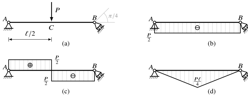
Figura 15.21: Trave con cerniera in A e carrello inclinato di \pi/4 in B, con forza concentrata P in mezzzeria C: (a) schema strutturale; (b) sforzo normale N , uniforme in compressione -P/2 ; (c) taglio T , pari a +P/2 nel tratto AC e -P/2 nel tratto CB, con salto -P in C; (d) momento flettente M , lineare a tratti con massimo P\ell/4 in C.
