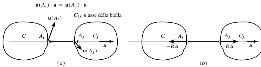
Figura 9.3: Biella interna fra i corpi C_i e C_j , con punti di applicazione A_i e A_j e versore d'asse \mathbf{a} = \overrightarrow{A_i A_j} / |\overrightarrow{A_i A_j}| . Prestazione cinematica (a): l'equazione di vincolo \mathbf{u}(A_i) \cdot \mathbf{a} = \mathbf{u}(A_j) \cdot \mathbf{a} impone l'uguaglianza delle componenti degli spostamenti di A_i e A_j lungo l'asse \mathbf{a} ; la componente trasversale e la rotazione relativa restano libere e non sono rappresentate. Prestazione statica (b): le reazioni scambiate fra i due corpi sono una coppia di forze uguali e opposte \pm R \mathbf{a} applicate in A_i e A_j , in accordo con la molteplicità uno.
