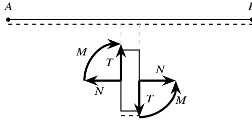
Figura 14.6: Concio di trave e convenzione di segno delle caratteristiche della sollecitazione. Sulla faccia destra (normale uscente +z^e ) N, T, M sono positivi se concordi con gli assi del riferimento intrinseco; sulla faccia sinistra (normale uscente -z^e ) i versi positivi sono opposti.
