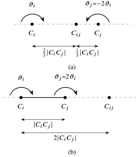
Figura 6.9: Allineamento dei centri di rotazione C_i , C_j e C_{ij} con |\vartheta_j| = 2|\vartheta_i| . (a) Rotazioni discordi ( \vartheta_i > 0, \vartheta_j = -2\vartheta_i ): C_{ij} cade all'interno del segmento C_i C_j , a distanza \frac{2}{3}|C_i C_j| da C_i . (b) Rotazioni concordi ( \vartheta_i > 0, \vartheta_j = 2\vartheta_i ): C_{ij} cade all'esterno, oltre C_j , a distanza 2|C_i C_j| da C_i .
