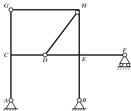
Figura 12.1: Esempio di struttura a connessioni eterogenee. Vincoli esterni: cerniere al suolo in A e B, carrello verticale in F. La traversa intermedia C–D–E–F è continua attraverso C ed E ed è sconsnessa in D con cerniera interna. La traversa G–H termina in G con cerniera d'estremità. In H la traversa G–H e il tratto E–H sono continui, mentre la diagonale D–H vi si connette con cerniera d'estremità.
