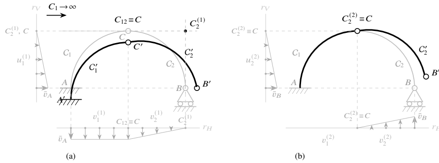
Figura 11.15: Arco a tutto sesto con incastro: contributi separati dei due cedimenti al metodo grafo-analitico. (a) Contributo \bar{v}_A : C_1 trasla verso il basso ( C_1 punto improprio di x ); C_2 ruota attorno a C_2^{(1)} (intersezione dell'orizzontale per C con la verticale per B ); su r_H sono riportate le tracce di C_{12} \equiv C e C_2^{(1)} e i campi u e v di C_1 e C_2 . (b) Contributo \bar{v}_B : C_1 fisso, C fisso; C_2 ruota attorno a C_2^{(2)} \equiv C ; su r_H sono riportate la traccia di C_2^{(2)} \equiv C e i campi u e v di C_2 .
