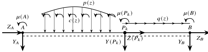
Figura 14.3: Azioni esterne su una trave rettilinea piana: carichi distribuiti p(z), q(z), c(z) definiti a tratti; forze e coppia concentrate Z(P_k), Y(P_k), \mu(P_k) in un punto interno P_k ; forze e coppie agli estremi Z_A, Y_A, \mu(A) in A e Z_B, Y_B, \mu(B) in B .
