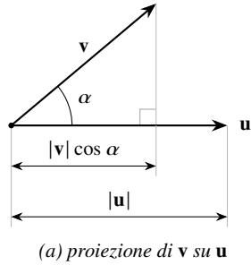
Figura 5.3: Rappresentazione geometrica del prodotto scalare.
