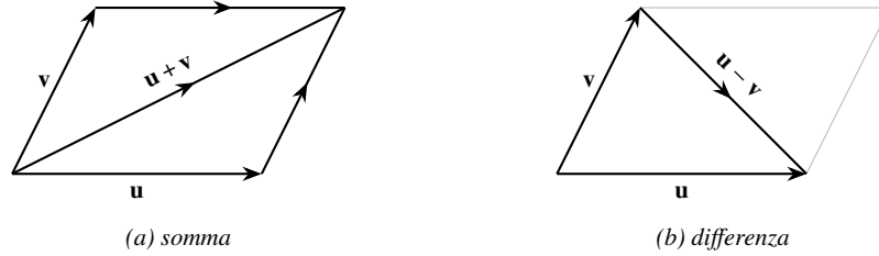
Figura 5.1: Somma e differenza di due vettori.
