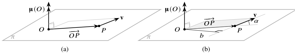
Figura 5.7: Momento polare di un vettore applicato: (a) definizione come prodotto vettoriale \overrightarrow{OP} \times \mathbf{v} ; (b) calcolo come prodotto del modulo |\mathbf{v}| per il braccio b .
