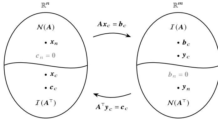
Figura 4.3: Struttura dei problemi primale A\mathbf{x} = \mathbf{b} e duale A^T\mathbf{y} = \mathbf{c} . Il pedice c denota la componente complementare al nucleo : \mathbf{x}_c \in I(A^T) , \mathbf{b}_c \in I(A) , \mathbf{y}_c \in I(A) , \mathbf{c}_c \in I(A^T) . Il pedice n denota la componente nel nucleo: \mathbf{x}_n \in N(A) , \mathbf{y}_n \in N(A^T) . Il primale ammette soluzione se e solo se \mathbf{b}_n = \mathbf{0} ; il duale se e solo se \mathbf{c}_n = \mathbf{0} .
