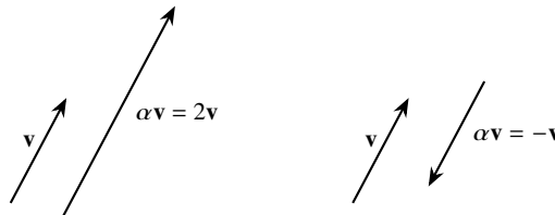
Figura 5.2: Prodotto di un vettore \mathbf{v} per uno scalare: \alpha = 2 (sinistra) e \alpha = -1 (destra).
