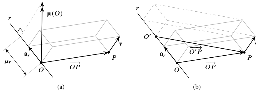
Figura 5.10: Momento assiale di un vettore applicato. (a) Il momento assiale è la proiezione \mu_r del momento polare \boldsymbol{\mu}(O) sulla retta r e coincide con il volume con segno del parallelepipedo di spigoli \overrightarrow{OP} , \mathbf{v} e \mathbf{a}_r . (b) Invarianza rispetto al punto scelto sulla retta: i parallelepipedi costruiti da O e da O' condividono la faccia in P generata da \mathbf{v} e \mathbf{a}_r , e le facce opposte giacciono entrambe nel piano per r parallelo a \mathbf{v} ; i volumi coincidono per scorrimento.
