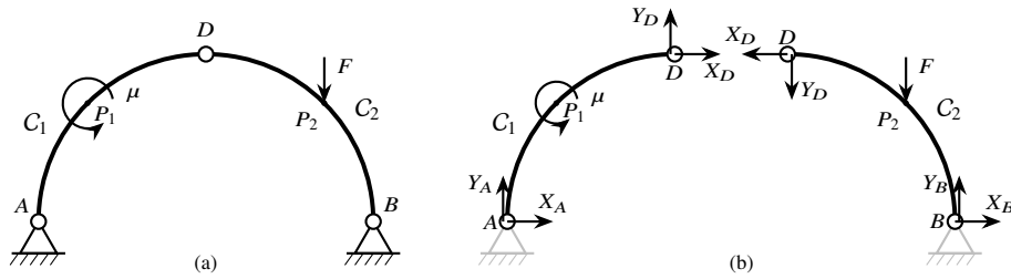
Figura 11.4: Arco a tre cerniere (Esempio 11.2): (a) dati del problema statico — carico verticale F in P_2 (punto medio dell'asse di C_2 ) e coppia \mu antioraria in P_1 (punto medio dell'asse di C_1 ); le frecce indicano il verso positivo dei carichi assegnati. (b) schemi dei corpi liberi di C_1 (sinistra) e C_2 (destra): reazioni esterne X_A, Y_A in A e X_B, Y_B in B ; reazioni interne X_D, Y_D in D , uguali e opposte sui due corpi.
