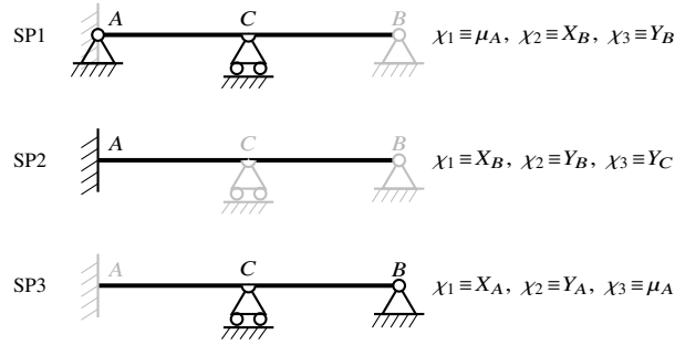
Figura 11.10: Trave iperstatica di grado 3 (Esempio 11.7): tre sistemi principali isostatici. I vincoli rimossi sono in grigio; le corrispondenti reazioni diventano le incognite iperstatiche \chi_1, \chi_2, \chi_3 .
