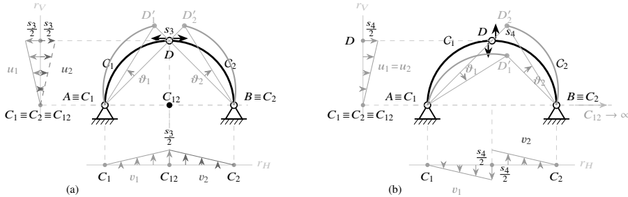
Figura 11.3: Soluzione grafica per i cedimenti interni in D. (a) cedimento s_3 (orizzontale): tre centri distinti, C_1 \equiv A , C_2 \equiv B fissati dai vincoli a cedimento nullo, C_{12} punto medio di AB. (b) cedimento s_4 (verticale): caso degenerare, C_{12} punto improprio della direzione orizzontale, e i due semiarchi ruotano della stessa quantità attorno ai rispettivi centri C_1 \equiv A e C_2 \equiv B .
