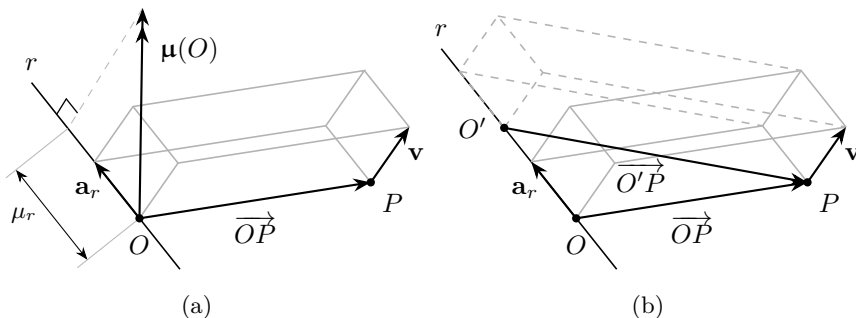
Figura 2.10. Momento assiale di un vettore applicato. (a) Il momento assiale è la proiezione \mu_r del momento polare \mu(O) sulla retta r e coincide con il volume con segno del parallelepipedo di spigoli \overrightarrow{OP} , \mathbf{v} e \mathbf{a}_r . (b) Invarianza rispetto al punto scelto sulla retta: i parallelepipedi costruiti da O e da O' condividono la faccia in P generata da \mathbf{v} e \mathbf{a}_r , e le facce opposte giacciono entrambe nel piano per r parallelo a \mathbf{v} ; i volumi coincidono per scorrimento.
