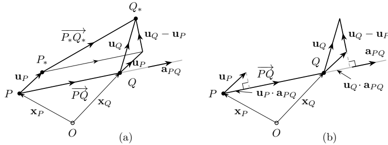
Figura 5.2. (a) Spostamenti rigidi e (b) interpretazione geometrica della condizione di ortogonalità fra il vettore posizione relativo \overrightarrow{PQ} e il vettore relativo degli spostamenti infinitesimi \mathbf{u}_Q - \mathbf{u}_P .
