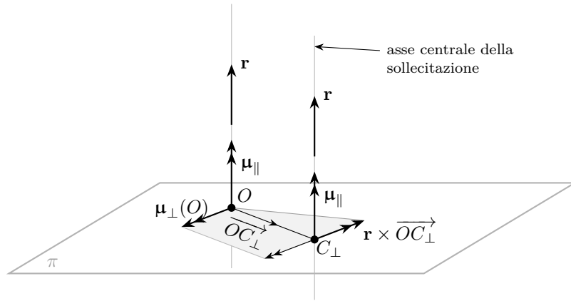
Figura 2.2. Costruzione geometrica dell'asse centrale del sistema di forze. Il momento rispetto a O si decompone nella componente \mu_{||}^O , parallela a \mathbf{r} e invariante per tutti i poli, e nella componente \mu_{\perp}^O , giacente nel piano \pi ortogonale a \mathbf{r} . Il punto C_{\perp} , intersezione dell'asse centrale con \pi , è determinato dalla condizione \mathbf{r} \times \overrightarrow{OC_{\perp}} = -\mu_{\perp}^O ; l'asse centrale è la retta per C_{\perp} parallela a \mathbf{r} .
