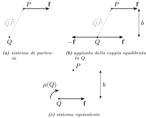
Figura 2.4. Trasporto di una forza in un punto non appartenente alla linea d'azione. (a) Sistema originale: forza \mathbf{f} applicata in P . (b) Aggiunta in Q della coppia equilibrata (\mathbf{f}, -\mathbf{f}) : la forza (P, \mathbf{f}) e (Q, -\mathbf{f}) formano una coppia di momento \boldsymbol{\mu} = \overrightarrow{QP} \times \mathbf{f} , con braccio b . (c) Sistema equivalente: forza \mathbf{f} applicata in Q più la coppia correttiva oraria di intensità \mu(Q) = |\mathbf{f}| b .
