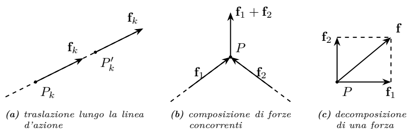
Figura 2.3. Operazioni elementari di equivalenza (I). (a) Traslazione della forza \mathbf{f}_k lungo la propria linea d'azione da P_k a P'_k : risultante e momento risultante restano invariati. (b) Composizione di due forze concorrenti in P : il sistema è equivalente alla risultante \mathbf{f}_1 + \mathbf{f}_2 applicata in P . (c) Decomposizione della forza \mathbf{f} applicata in P nelle componenti \mathbf{f}_1 e \mathbf{f}_2 secondo due direzioni indipendenti: operazione inversa alla composizione.
