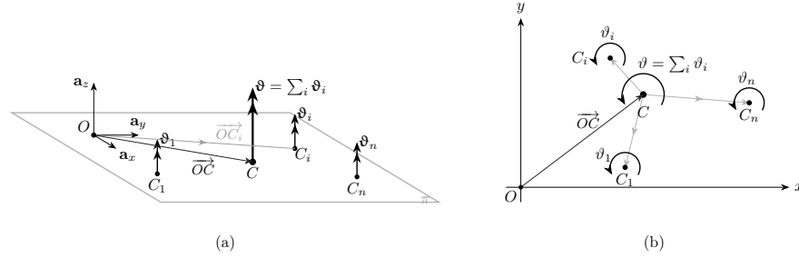
Figura 2.8. Composizione di n rotazioni infinitesime nel piano. (a) Vista tridimensionale: le rotazioni sono vettori assiali \boldsymbol{\vartheta}_i ortogonali al piano \pi , che si sommano nella risultante \boldsymbol{\vartheta} = \sum_i \boldsymbol{\vartheta}_i in C . (b) Vista nel piano (x, y) : ampiezze \vartheta_i come archi orientati (positivi se antiorari) e centro risultante C nel baricentro dei C_i . Il centro C è individuato da \overrightarrow{OC} = (\sum_i \vartheta_i \overrightarrow{OC_i}) / \vartheta o, in forma equivalente, da \sum_i \vartheta_i \overrightarrow{CC_i} = \mathbf{0} (freccie grigie in (b)).
