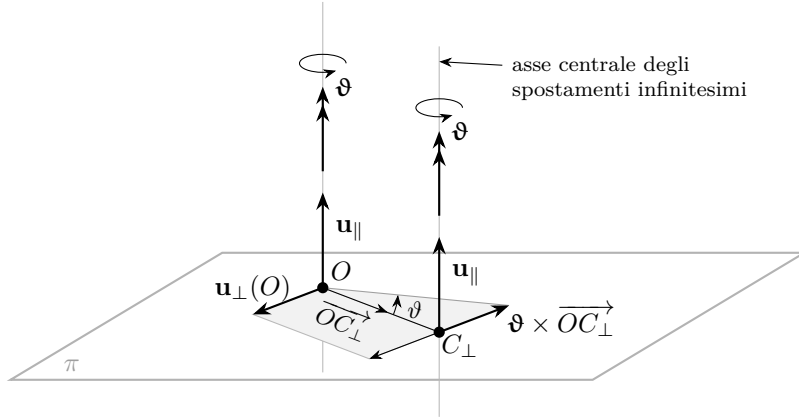
Figura 2.6. Costruzione geometrica dell'asse centrale degli spostamenti rigidi infinitesimi. Lo spostamento di O si decompone nella componente \mathbf{u}_\parallel , parallela a \boldsymbol{\vartheta} e invariante per tutti i punti del corpo, e nella componente \mathbf{u}_\perp(O) , giacente nel piano \pi ortogonale a \boldsymbol{\vartheta} . Il punto C_\perp , intersezione dell'asse centrale con \pi , è determinato dalla condizione \boldsymbol{\vartheta} \times \overrightarrow{OC}_\perp = -\mathbf{u}_\perp(O) ; l'asse centrale è la retta per C_\perp parallela a \boldsymbol{\vartheta} .
