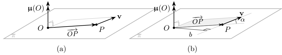
Figura 2.7. Momento polare di un vettore applicato: (a) definizione come prodotto vettoriale \vec{OP} \times \mathbf{v} ; (b) calcolo come prodotto del modulo |\mathbf{v}| per il braccio b .
