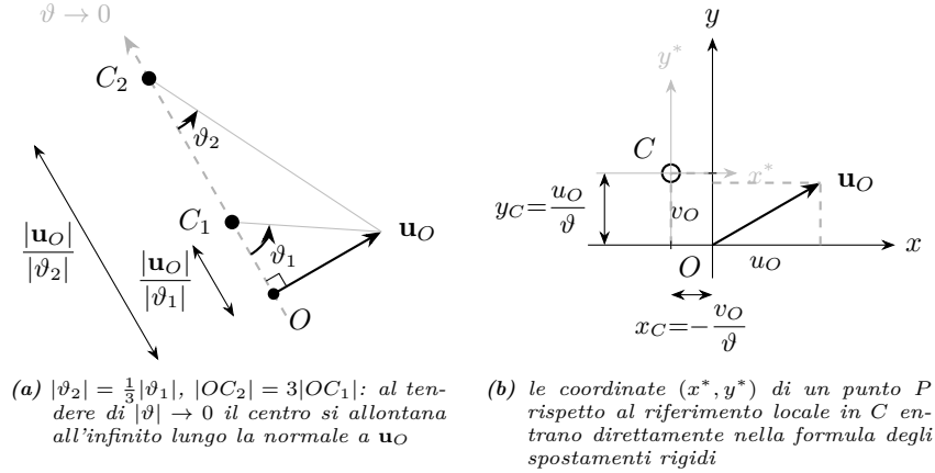
Figura 2.7. Centro di rotazione nel caso piano. (a) Costruzione geometrica: C si ottiene ruotando \mathbf{u}_O di 90^\circ nel verso di \vartheta e riscalando di 1/|\vartheta| . (b) Riferimento locale con origine in C e assi x^*, y^* paralleli a x, y : le coordinate (x^*, y^*) di un punto P entrano direttamente nella (2.58).
