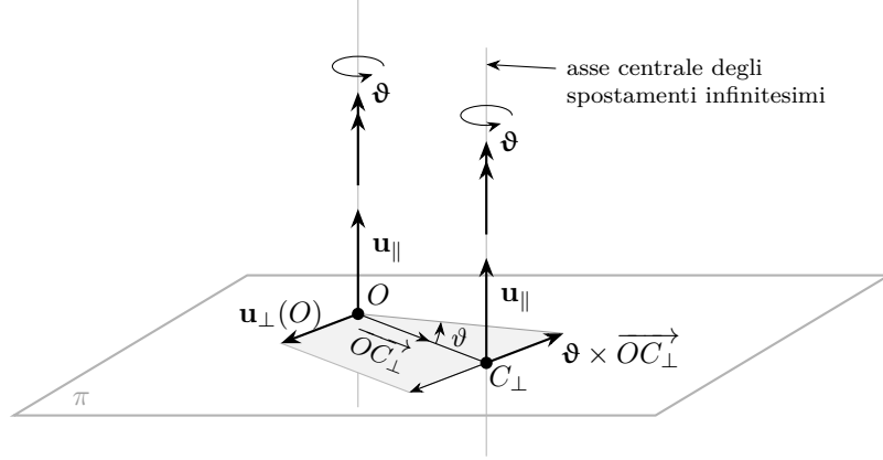
Figura 2.6. Costruzione geometrica dell'asse centrale degli spostamenti rigidi infinitesimi. Lo spostamento di O si decompone nella componente \mathbf{u}_{\parallel} , parallela a \mathfrak{D} e invariante per tutti i punti del corpo, e nella componente \mathbf{u}_{\perp}(O) , giacente nel piano \pi ortogonale a \mathfrak{D} . Il punto C_{\perp} , intersezione dell'asse centrale con \pi , è determinato dalla condizione \mathfrak{D} \times \overrightarrow{OC_{\perp}} = -\mathbf{u}_{\perp}(O) ; l'asse centrale è la retta per C_{\perp} parallela a \mathfrak{D} .
