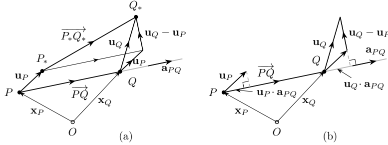
Figura 1.4. (a) Spostamenti rigidi e (b) interpretazione geometrica della condizione di ortogonalità fra il vettore posizione relativo \overrightarrow{PQ} e il vettore relativo degli spostamenti infinitesimi \mathbf{u}_Q - \mathbf{u}_P .
