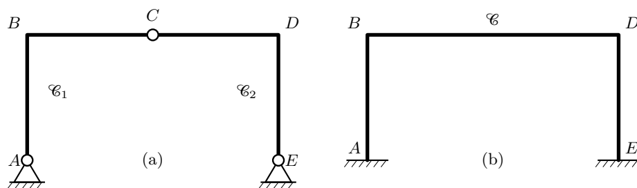
Figura 7.12. (a) Portale a tre cerniere e (b) e portale incastrato.
