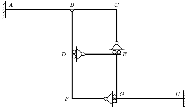
Figura 7.10. Struttura mista: due mensole ad asse spezzato \mathcal{S}_1 = ABCE (incastrata in A ) e \mathcal{S}_2 = HGED (incastrata in H ), collegate da una trave appoggiata \mathcal{S}_3 = BDFG (cerniera in B , carrello in G ). I carrelli in D ed E aggiungono due vincoli semplici allo schema isostatico di riferimento: \nu = -2 , iperstatica di grado 2.
