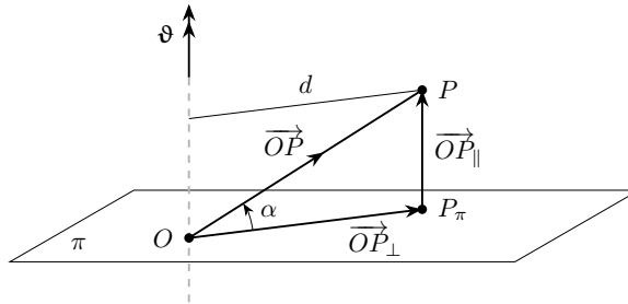
Figura 1.3. Interpretazione geometrica del termine rotazionale \boldsymbol{\vartheta} \times \overrightarrow{OP} : la componente \overrightarrow{OP}_\perp , ortogonale all'asse di rotazione, determina la distanza d del punto P dall'asse; lo spostamento rotazionale ha modulo |\boldsymbol{\vartheta}| d ed è tangente alla circonferenza di raggio d .
