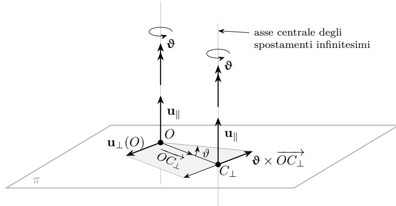
Figura 2.6. Costruzione geometrica dell'asse centrale degli spostamenti rigidi infinitesimi. Lo spostamento di O si decompone nella componente \mathbf{u}_{\parallel} , parallela a \boldsymbol{\vartheta} e invariante per tutti i punti del corpo, e nella componente \mathbf{u}_{\perp}(O) , giacente nel piano \pi ortogonale a \boldsymbol{\vartheta} . Il punto C_{\perp} , intersezione dell'asse centrale con \pi , è determinato dalla condizione \boldsymbol{\vartheta} \times \overrightarrow{OC_{\perp}} = -\mathbf{u}_{\perp}(O) ; l'asse centrale è la retta per C_{\perp} parallela a \boldsymbol{\vartheta} .
