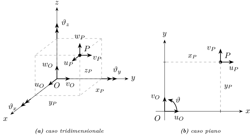
Figura 2.5. Parametri cinematici del corpo rigido e componenti dello spostamento di un punto generico P nel caso (a) tridimensionale (sei gradi di libertà: u_O , v_O , w_O , \vartheta_x , \vartheta_y , \vartheta_z ) e (b) piano (tre gradi di libertà: u_O , v_O , \vartheta ).
