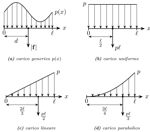
Figura 4.7. Riduzione di carichi distribuiti \mathbf{f}_L(x) = -p(x)\mathbf{a}_y con p(x) \geq 0 su un intervallo di lunghezza \ell : la risultante (freccia spessa) è applicata nel baricentro del diagramma di carico. (a) Caso generico p(x) : risultante |f| applicata a distanza d . (b) Carico uniforme: |f| = p\ell , d = \ell/2 . (c) Carico lineare: |f| = p\ell/2 , d = 2\ell/3 . (d) Carico parabolico: |f| = p\ell/3 , d = 3\ell/4 .
