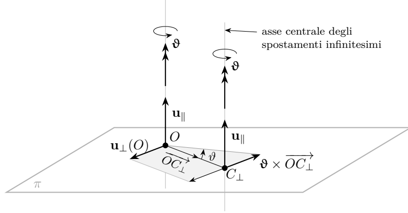
Figura 3.6. Costruzione geometrica dell'asse centrale degli spostamenti rigidi infinitesimi. Lo spostamento di O si scompone nella componente \mathbf{u}_{\parallel} , parallela a \boldsymbol{\vartheta} e invariante per tutti i punti del corpo, e nella componente \mathbf{u}_{\perp}(O) , giacente nel piano \pi ortogonale a \boldsymbol{\vartheta} . Il punto C_{\perp} , intersezione dell'asse centrale con \pi , è determinato dalla condizione \boldsymbol{\vartheta} \times \overrightarrow{OC_{\perp}} = -\mathbf{u}_{\perp}(O) ; l'asse centrale è la retta per C_{\perp} parallela a \boldsymbol{\vartheta} .
