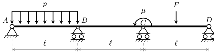
Figura 17.18. Trave continua a tre campate di uguale luce \ell : carico uniformemente distribuito p sul tratto AB , coppia concentrata \mu nella sezione C , forza concentrata F a mezzzeria del tratto CD . Il cerchio in A e D indica il perno; il semicerchio in B e C indica che la trave scorre sull'appoggio senza interruzione della continuità rotazionale.
