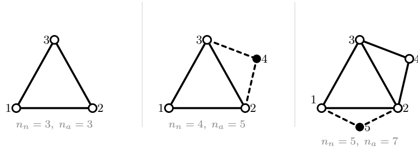
Figura 18.2. Costruzione gerarchica di una travatura reticolare internamente isostatica. A sinistra: triangolo base ( n_n = 3 , n_a = 3 ). Al centro: aggiunta del primo nodo ( n_n = 4 , n_a = 5 ). A destra: aggiunta del secondo nodo ( n_n = 5 , n_a = 7 ). In ciascun passo le due aste nuove sono tratteggiate e il nuovo nodo è indicato con un cerchio pieno.
