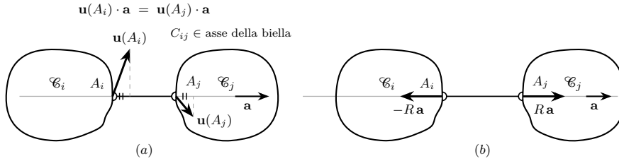
Figura 9.3. Biella interna fra i corpi \mathcal{C}_i e \mathcal{C}_j , con punti di applicazione A_i e A_j e versore d'asse \mathbf{a} = \overrightarrow{A_i A_j} / |\overrightarrow{A_i A_j}| . Prestazione cinematica (a): l'equazione di vincolo \mathbf{u}(A_i) \cdot \mathbf{a} = \mathbf{u}(A_j) \cdot \mathbf{a} impone l'uguaglianza delle componenti degli spostamenti di A_i e A_j lungo l'asse \mathbf{a} ; la componente trasversale e la rotazione relativa restano libere e non sono rappresentate. Prestazione statica (b): le reazioni scambiate fra i due corpi sono una coppia di forze uguali e opposte \pm R \mathbf{a} applicate in A_i e A_j , in accordo con la molteplicità uno.
