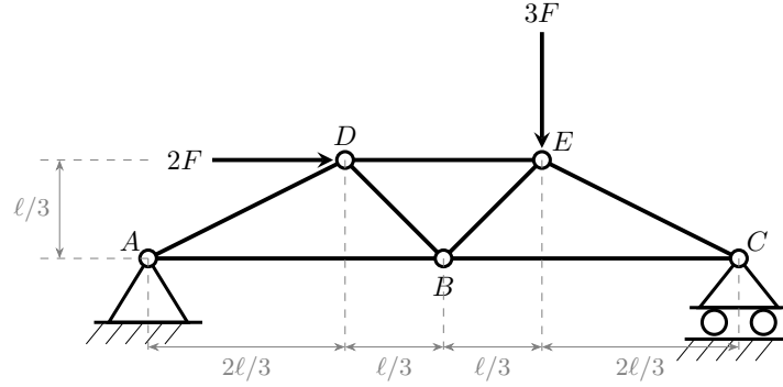
Figura 18.24. Travatura a tre maglie triangolari ADB , DBE , BCE . Geometria simmetrica rispetto alla mezzeria x = \ell ; carichi non simmetrici: forza orizzontale 2F in D e forza verticale 3F in E .
