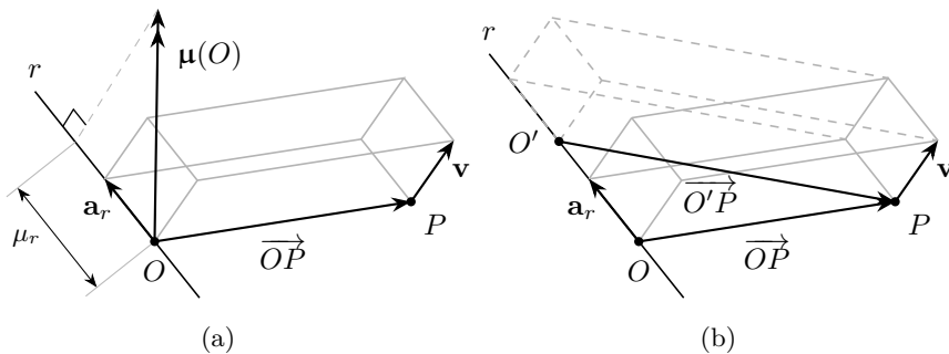
Figura 5.10. Momento assiale di un vettore applicato. (a) Il momento assiale è la proiezione \mu_r del momento polare \mu(O) sulla retta r e coincide con il volume con segno del parallelepipedo di spigoli \overrightarrow{OP} , \mathbf{v} e \mathbf{a}_r . (b) Invarianza rispetto al punto scelto sulla retta: i parallelepipedi costruiti da O e da O' condividono la faccia in P generata da \mathbf{v} e \mathbf{a}_r , e le facce opposte giacciono entrambe nel piano per r parallelo a \mathbf{v} ; i volumi coincidono per scorrimento.
