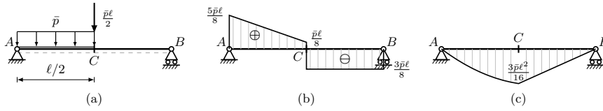
Figura 15.8. Trave appoggiata con carico uniformemente distribuito p(z) = \bar{p} (verso il basso) nel tratto AC di lunghezza \ell/2 e forza concentrata Y(C) = \bar{p}\ell/2 (verso il basso) in C : (a) schema strutturale; (b) diagramma del taglio T(z) , lineare decrescente nel tratto AC da 5\bar{p}\ell/8 in A a \bar{p}\ell/8 in C^- , con salto -\bar{p}\ell/2 in C , e uniforme pari a -3\bar{p}\ell/8 nel tratto CB ; (c) diagramma del momento flettente M(z) , parabolico con concavità verso l'alto nel tratto AC e lineare decrescente nel tratto CB , continuo in C con valore massimo 3\bar{p}\ell^2/16 e nullo agli estremi.
