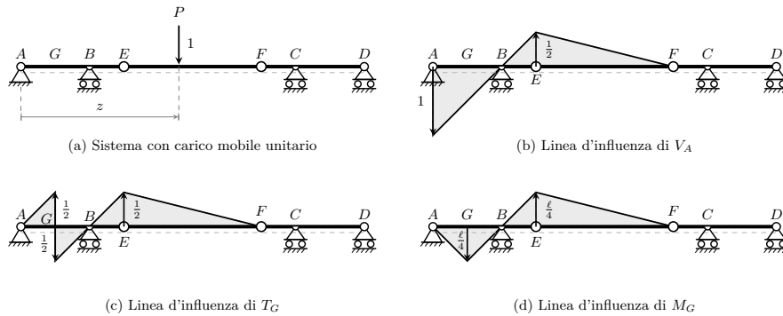
Figura 20.3. Trave di Gerber: linee di influenza di V_A (reazione in A ), T_G (taglio in mezzeria di AB ) e M_G (momento in mezzeria di AB ), sotto carico unitario verticale mobile. (a) Sistema con carico in posizione generica di ascissa z ; (b), (c), (d) linee di influenza costruite come spostamenti virtuali dei meccanismi duali (TSV). Le frecce indicano i valori delle ordinate virtuali nei vertici notevoli.
