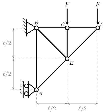
Figura 18.26. Mensola reticolare a tre maglie triangolari ABE , BCE , CDE , vincolata a una parete verticale. Carrello a piano di scorrimento verticale in A (reazione orizzontale) e cerniera in B ; carichi verticali F nei nodi C ed D .
