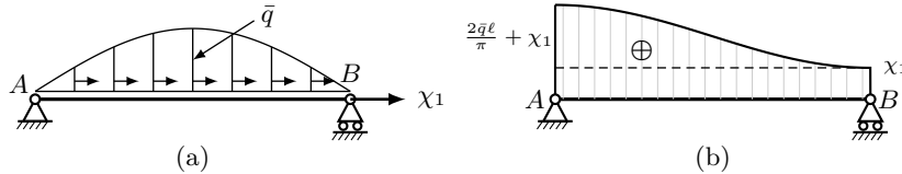
Figura 15.27. a) sistema principale soggetto al carico e alla forza iperstatica \chi_1 ; b) sforzo normale N = N_0 + \chi_1 N_1 , ottenuto traslando N_0 della costante \chi_1 (livello tratteggiato).
