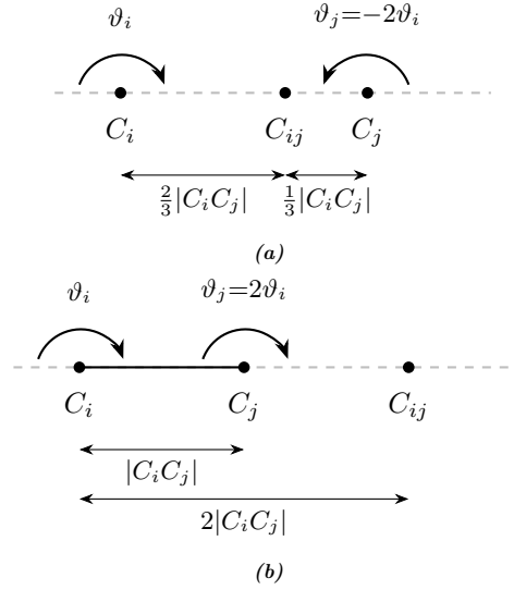
Figura 6.9. Allineamento dei centri di rotazione C_i , C_j e C_{ij} con |\vartheta_j| = 2|\vartheta_i| . (a) Rotazioni discordi ( \vartheta_i > 0 , \vartheta_j = -2\vartheta_i ): C_{ij} cade all'interno del segmento C_i C_j , a distanza \frac{2}{3}|C_i C_j| da C_i . (b) Rotazioni concordi ( \vartheta_i > 0 , \vartheta_j = 2\vartheta_i ): C_{ij} cade all'esterno, oltre C_j , a distanza 2|C_i C_j| da C_i .
