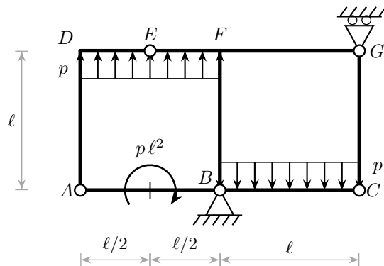
Figura 17.8. Anelli a tre cerniere: struttura chiusa a due celle quadrate \ell \times \ell con montante centrale BF in comune. Cerniere interne in A, E, B, C, G ; nodi rigidi in D ed F . Cerniera esterna in B , carrello verticale in G . Carico uniforme p verso l'alto su DF e verso il basso su BC ; coppia oraria p\ell^2 su AB .
