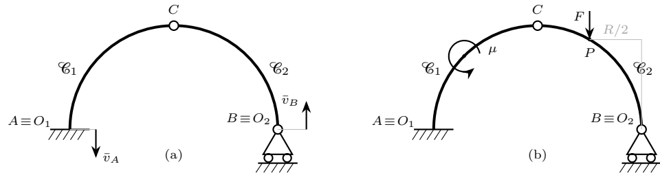
Figura 11.14. Arco a tutto sesto con incastro: poli O_1 \equiv A e O_2 \equiv B . (a) Dato cinematico: cedimento verticale \bar{v}_A verso il basso all'incastro in A e cedimento verticale \bar{v}_B verso l'alto al carrello in B . (b) Dato statico: coppia \mu antioraria su \mathcal{C}_1 e forza verticale F verso il basso su \mathcal{C}_2 , a distanza orizzontale R/2 da B .
