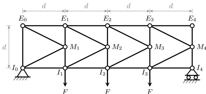
Figura 18.28. Travatura a K a quattro celle quadrate di lato d ; i nodi di mezzeria M_i stanno a metà altezza dei montanti. Cerniera in I_0 , carrello in I_4 , carichi F ai nodi d'intradosso interni.
