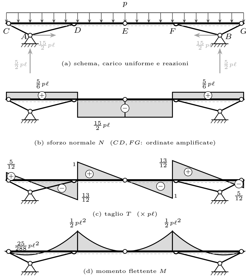
Figura 17.21. Caso (a), carico p su tutta la travata CDEFG — (a) schema e reazioni; (b) sforzo normale N sulle travi (le bielle, scariche, portano N uniforme: N_{AC} = N_{BG} = -\frac{5\sqrt{5}}{12} , N_{AD} = N_{BF} = -\frac{25\sqrt{17}}{12} , in p\ell ); (c) taglio T ; (d) momento flettente M , dal lato delle fibre tese. Scale indipendenti; M = 0 alle cerniere C, E, G ; i diagrammi N e M simmetrici rispetto a E , quello di T è emisimmetrico.
