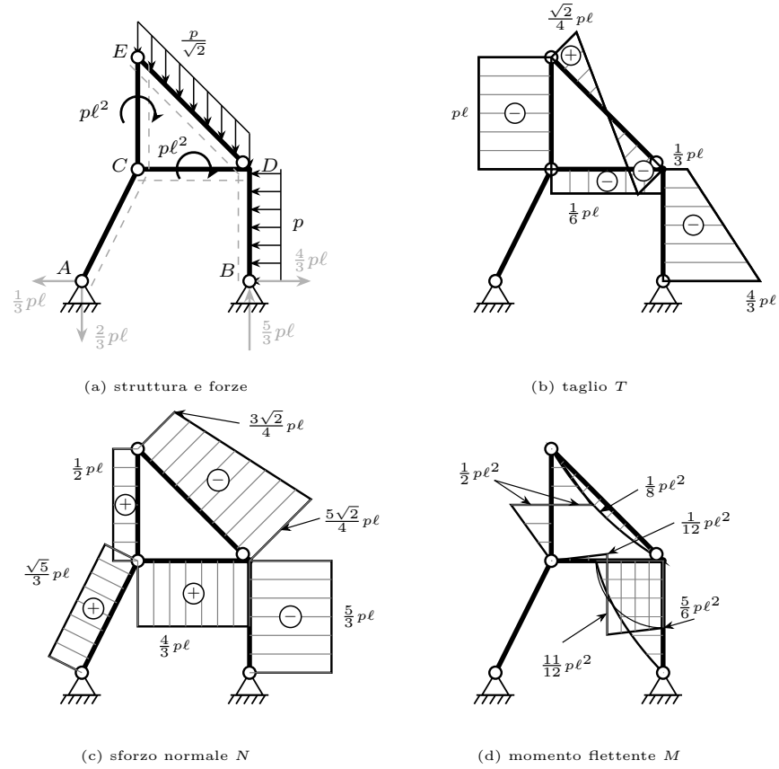
Figura 17.13. Sistemi composti a tre cerniere: (a) schema strutturale con i carichi, le reazioni vincolari e le fibre inferiori di riferimento; (b) taglio T ; (c) sforzo normale N ; (d) momento flettente M . Sull'asta inclinata ED le ordinate sono tracciate ortogonalmente all'asse; al nodo rigido D il diagramma del momento è continuo dal lato interno. I tre diagrammi adottano fattori di scala indipendenti.
