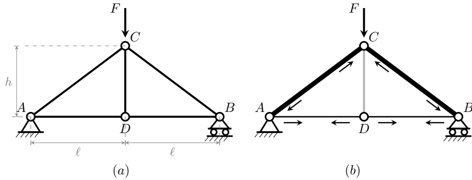
Figura 18.14. Capriata triangolare con carico al colmo. (a): schema strutturale con denominazione dei nodi. (b): stato di sollecitazione qualitativo. Tratto spesso: aste compresse AC e CB (puntoni); le frecce mostrano la compressione interna, con le estremità spinte verso l'esterno. Tratto sottile: aste tese AD e DB (tiranti); le frecce mostrano la trazione interna, con le estremità tirate verso il centro. In grigio il monaco CD : sforzo nullo per simmetria con carico al colmo.
