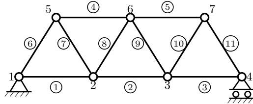
Figura 18.1. Travatura reticolare piana isostatica con n_n = 7 nodi, n_a = 11 aste e m_{\text{est}} = 3 (cerniera nel nodo 1, carrello nel nodo 4). I nodi sono numerati 1–7, le aste 1–11 con il numero cerchiato.
