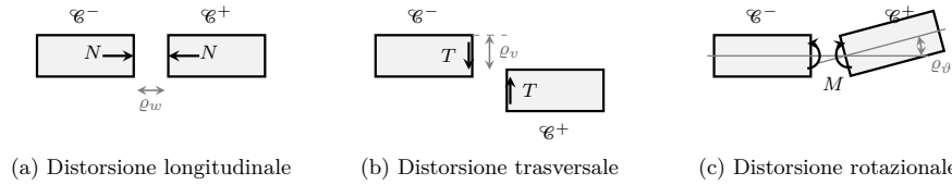
Figura 14.5. Distorsioni di concio e caratteristiche della sollecitazione duali: la coppia (\boldsymbol{\sigma}, \boldsymbol{\varrho}) entra nell'identità bilineare con segno discorde.
