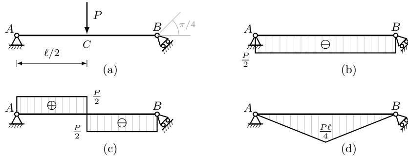
Figura 15.21. Trave con cerniera in A e carrello inclinato di \pi/4 in B, con forza concentrata P in mezzeria C: (a) schema strutturale; (b) sforzo normale N , uniforme in compressione -P/2 ; (c) taglio T , pari a +P/2 nel tratto AC e -P/2 nel tratto CB, con salto -P in C; (d) momento flettente M , lineare a tratti con massimo P\ell/4 in C.
