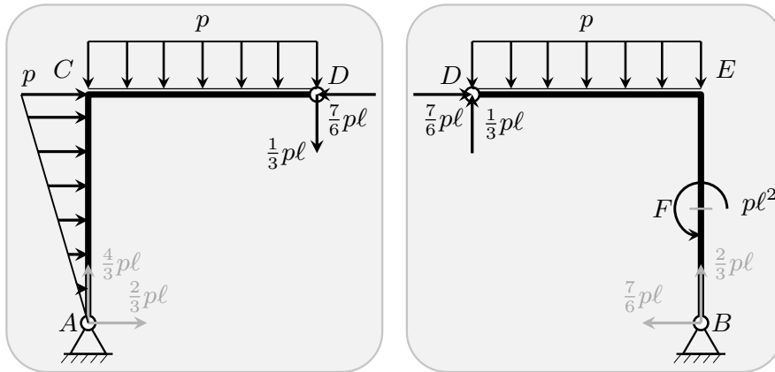
Figura 17.5. Arco a tre cerniere: isolamento dei due semiarci come corpi liberi.
