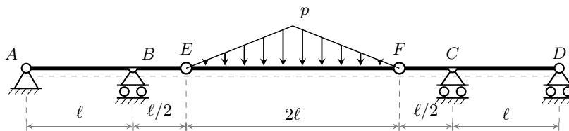
Figura 17.15. Trave di Gerber su quattro appoggi ( n_a = 4 , n_e = 5 , n_c = 2 ): cerniera in A , appoggi continui in B e C , carrello in D , cerniere interne in E e F . Luci: AB = CD = \ell , BE = FC = \ell/2 , EF = 2\ell . La campata portata EF è soggetta a un carico trasversale triangolare di intensità massima p nella sezione di mezzeria e nulla agli estremi E e F .
