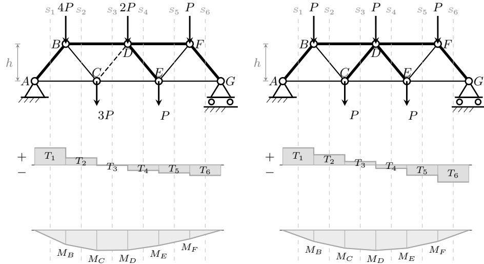
Figura 18.16. Analogia della trave equivalente per travature reticolari piane a correnti paralleli. Colonna sinistra: carichi asimmetrici 4P , 3P , 2P , P , P ai nodi B, C, D, E, F ; il diagramma del taglio ha cambio di segno tra T_2 e T_3 , e il poligono del momento ha massimo in C . Colonna destra: carichi uniformi P a tutti i nodi interni; il diagramma del taglio è antisimmetrico con gradini uguali, e il poligono del momento è simmetrico con massimo in D . I trattini verticali indicano i valori nodali M_B, \dots, M_F del momento flettente equivalente; le sezioni S_1, \dots, S_6 mostrano la corrispondenza tra taglio nel pannello e aste sezionate: lo sforzo nel corrente è proporzionale al momento M/h , quello nella diagonale al taglio T/\cos \alpha . Tratto spesso: asta compressa; tratto sottile: asta tesa; tratto tratteggiato: asta scarica (colonna sinistra, asta CD ).
