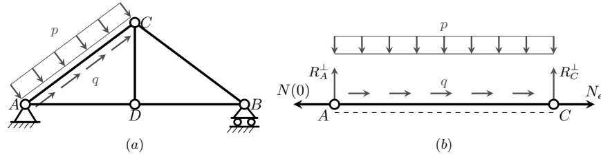
Figura 18.19. Asta reticolare AC soggetta a carichi generici. (a): schema strutturale della capriata con carico trasversale p (perpendicolare ad AC , sopra l'asta) e carico longitudinale q (radente ad AC da A verso C ). (b): asta AC isolata nel riferimento locale con z^e diretto da A verso C ; N_e e N(0) sono gli sforzi normali uscenti dalle due estremità; R_A^\perp e R_C^\perp sono le reazioni trasversali alle cerniere.
