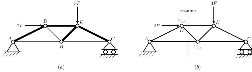
Figura 18.25. (a) Stato di sollecitazione: tratto spesso le aste compresse (puntoni AD, DE, BE, EC), tratto sottile le aste tese (tiranti AB, BC, DB). (b) Sezione di Ritter sul pannello centrale: il taglio attraversa AB, DB ed DE. I poli dei due correnti coincidono con nodi della travatura, P_{DE} \equiv B e P_{AB} \equiv D ; poiché i correnti AB e DE sono paralleli, il polo della diagonale DB è all'infinito e N_{DB} si ricava dall'equilibrio alla traslazione verticale.
