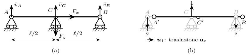
Figura 11.11. Trave con tre carrelli verticali paralleli: (a) dati del problema ; (b) meccanismo \mathbf{u}_1 (traslazione orizzontale) e stato di autoequilibrio \mathbf{r}_1 (reazioni verticali a risultante e momento nulli) .
