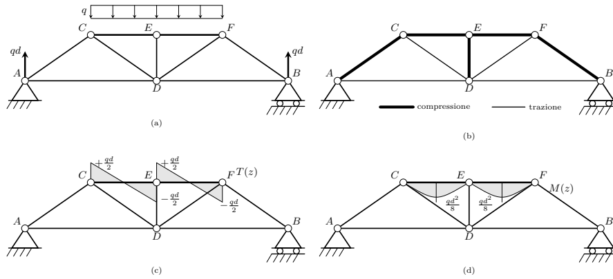
Figura 18.21. Travatura a correnti paralleli con carico distribuito q su CE ed EF . (a): schema di carico. (b): funzionamento strutturale — aste compresse a tratto spesso, aste tese a tratto sottile. (c): diagramma del taglio T(z) sulle aste CE ed EF . (d): diagramma del momento M(z) sulle aste CE ed EF .
