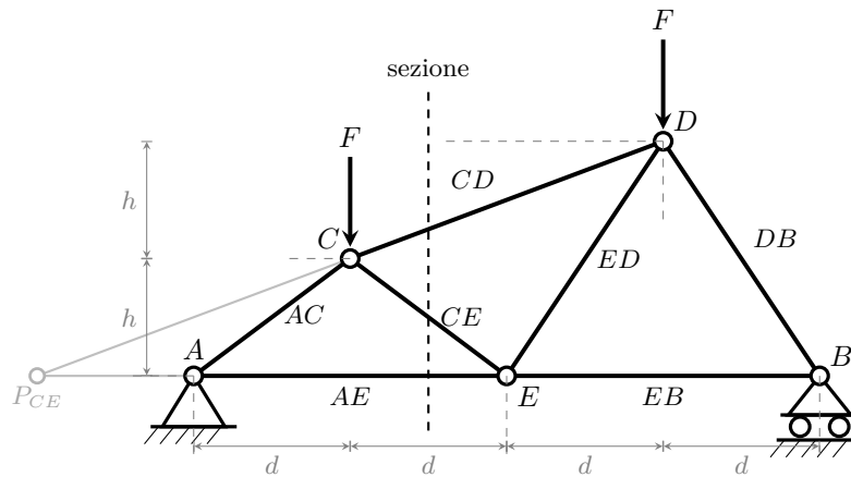
Figura 18.15. Capriata a correnti non paralleli. Schema strutturale con la sezione canonica di Ritter (linea tratteggiata verticale) che taglia le aste CD , AE e CE . I prolungamenti in grigio delle rette d'azione di CD e AE si incontrano nel polo P_{CE} = (-d, 0) , esterno alla struttura. I poli P_{CD} \equiv E e P_{AE} \equiv C coincidono con nodi della travatura.
