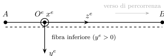
Figura 14.2. Riferimento intrinseco ( O^e; y^e, z^e ) di una trave rettilinea piana con estremi A e B . L'asse z^e è diretto nel verso di percorrenza da A a B ; l'asse y^e punta verso la fibra inferiore, indicata dalla linea tratteggiata parallela alla linea d'asse; l'asse x^e , uscente dal piano del foglio, completa il riferimento destrorso.
