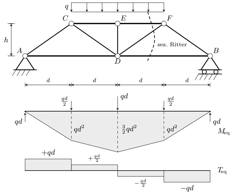
Figura 18.20. Travatura a correnti paralleli con carico distribuito sul corrente superiore. In alto: schema strutturale con sezione di Ritter tratteggiata nel pannello centrale. In basso: trave equivalente con diagrammi M_{eq} e T_{eq} .
