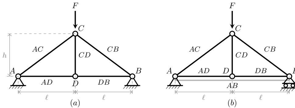
Figura 18.22. Varianti iperstatiche della capriata triangolare. (a) Iperstaticità esterna ( g_i^{\text{est}} = 1 ): il carrello in B è sostituito da una cerniera; il sistema principale si ottiene ripristinando il carrello. (b) Iperstaticità interna ( g_i^{\text{int}} = 1 ): l'asta ridondante AB (in grigio) è aggiunta alla capriata isostatica; il sistema principale si ottiene sopprimendo AB.
