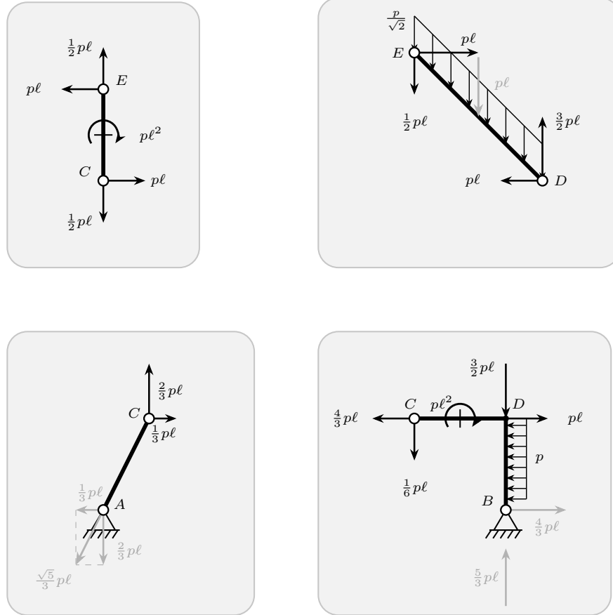
Figura 17.12. Sistemi composti a tre cerniere: esploso dei quattro corpi liberi con i carichi attivi e le forze scambiate alle connessioni, riportate nel riferimento globale. I trattini trasversali su CE e CD individuano i punti di applicazione delle coppie; su ED la freccia grigia p\ell è la risultante del carico distribuito. Sulla biella AC le componenti \frac{1}{3}p\ell e \frac{2}{3}p\ell compongono la risultante \frac{\sqrt{5}}{3}p\ell (in grigio), diretta lungo l'asse dell'asta. Le reazioni a terra in A e B sono in grigio.
