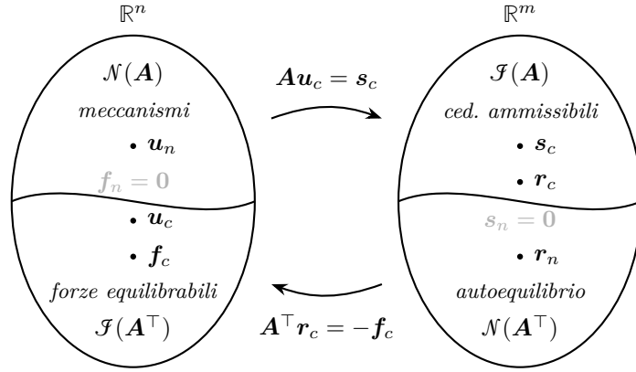
Figura 10.2. Struttura duale dei problemi cinematico \mathbf{A}\mathbf{u} = \mathbf{s} e statico \mathbf{A}^\top \mathbf{r} = -\mathbf{f} .
