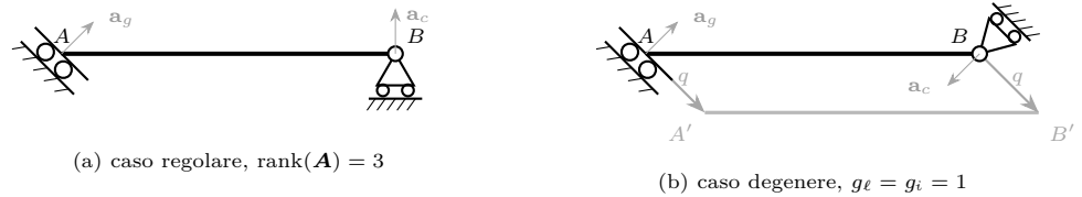
Figura 12.6. Trave con glifo in A e carrello in B : (a) caso regolare con assi \mathbf{a}_g e \mathbf{a}_c non paralleli ( \text{rank}(\mathbf{A}) = 3 , isostatico); (b) caso degenere con assi \mathbf{a}_g e \mathbf{a}_c collineari ( g_\ell = g_i = 1 ). In (b) il meccanismo è la traslazione del corpo nella direzione ortogonale agli assi, parametrizzata da q .
