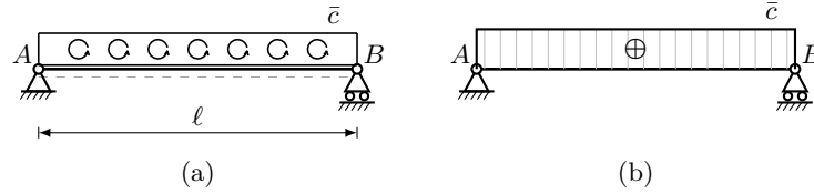
Figura 15.10. Trave appoggiata con coppie antiorarie uniformemente distribuite di intensità \bar{c} su tutta la lunghezza: (a) schema strutturale; (b) diagramma del taglio T(z) , uniforme pari a \bar{c} su tutta la trave. Il momento flettente è identicamente nullo, M(z) \equiv 0 , e non è riportato in figura: le coppie distribuite compensano esattamente il contributo del taglio ( M' = T - c = 0 ).
