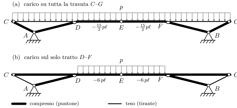
Figura 17.25. Confronto dei due funzionamenti sulla stessa struttura: tratto spesso = compressione (puntone), sottile = trazione (tirante). (a) carico sull'intera travata C-G : bielle d'impasta tutte compresse e corrente centrale DEF compresso ( N = -\frac{15}{2}p\ell ), con i soli tratti CD , FG tesi a catena locale degli anelli A-C-D e B-F-G . (b) carico sul solo tratto DF : l'intera navata C-G è compressa ( N = -6p\ell in mezzeria) con le bielle interne AD , BF ; si fanno tese le sole bielle d'estremità AC , BG . È lo specchio di (a), con i ruoli di catena e puntone scambiati fra navata e bielle.
