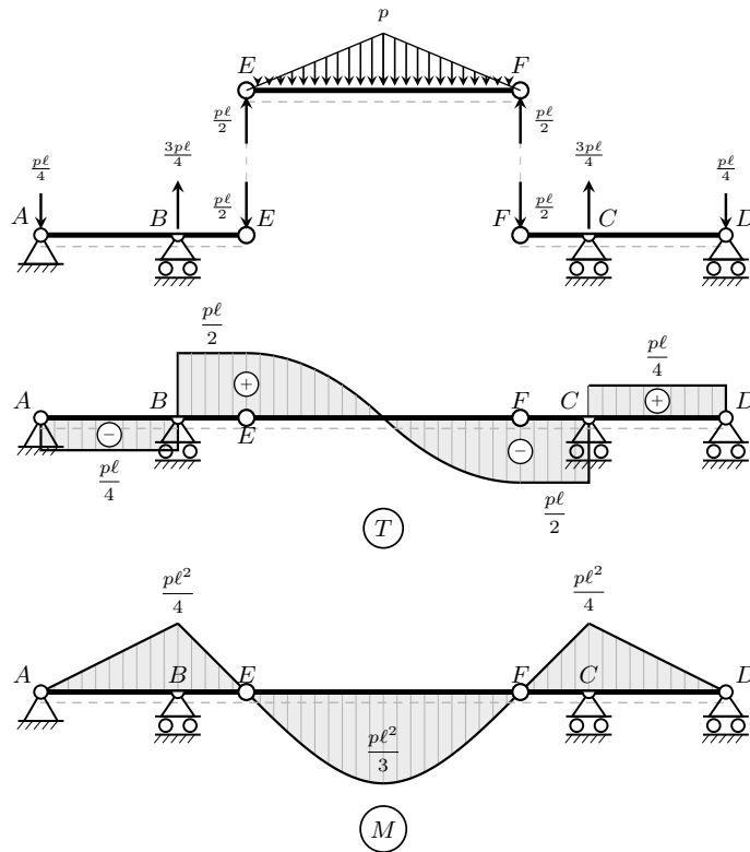
Figura 17.16. Trave di Gerber: schema delle reazioni (prima riga), taglio T (seconda riga) e momento M (terza riga). Le reazioni V_A = V_D = p\ell/4 verso il basso indicano che i perni A e D trattengono la trave. Il taglio è emisimmetrico; il momento è simmetrico, nullo in E e F , con massimo p\ell^2/3 (sagging) a mezzzeria di EF e valore p\ell^2/4 (hogging) agli appoggi B e C .
