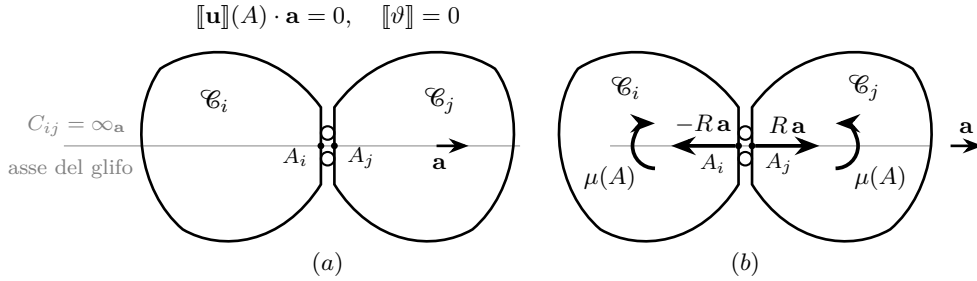
Figura 9.9. Glifo interno fra i corpi \mathcal{C}_i e \mathcal{C}_j con asse \mathbf{a} . Prestazione cinematica (a): le equazioni di vincolo [\![\mathbf{u}]\!](A) \cdot \mathbf{a} = 0 e [\![\vartheta]\!] = 0 impongono l'uguaglianza delle componenti di spostamento dei due corpi lungo \mathbf{a} e l'uguaglianza delle rotazioni \vartheta_i e \vartheta_j ; lo scorrimento relativo lungo \mathbf{a}^\perp resta libero. Il centro di rotazione relativo è all'infinito sulla retta dell'asse, C_{ij} = \infty_{\mathbf{a}} . Prestazione statica (b): i due corpi si scambiano una forza R\mathbf{a} diretta lungo l'asse e una coppia \mu(A) , uguali e opposte, in dualità rispettivamente con la componente di spostamento relativo lungo \mathbf{a} e con la rotazione relativa bloccate, in accordo con la molteplicità due.
