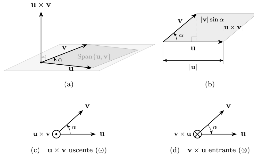
Figura 5.4. Rappresentazione geometrica del prodotto vettoriale \mathbf{u} \times \mathbf{v} . In (a) il vettore \mathbf{u} \times \mathbf{v} è ortogonale al piano \text{Span}\{\mathbf{u}, \mathbf{v}\} e orientato secondo la regola della mano destra; il suo modulo eguaglia l'area del parallelogramma costruito su \mathbf{u} e \mathbf{v} . In (b) tale area è letta come prodotto della base |\mathbf{u}| per l'altezza |\mathbf{v}| \sin \alpha , da cui |\mathbf{u} \times \mathbf{v}| = |\mathbf{u}| |\mathbf{v}| \sin \alpha . In (c) e (d) è illustrata l'antisimmetria \mathbf{u} \times \mathbf{v} = -(\mathbf{v} \times \mathbf{u}) : a parità di \mathbf{u} , \mathbf{v} e di angolo \alpha , il prodotto cambia verso — uscente dal piano ( \odot ) per \mathbf{u} \times \mathbf{v} , entrante ( \otimes ) per \mathbf{v} \times \mathbf{u} — coerentemente col senso di rotazione che porta il primo fattore sul secondo.
