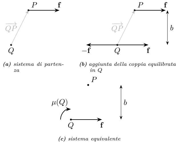
Figura 7.6. Trasporto di una forza in un punto non appartenente alla linea d'azione.
