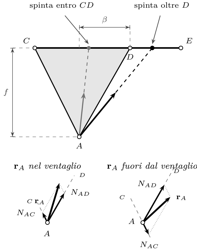
Figura 17.24. Sintesi del segno al nodo A . ( In alto ) Lettura geometrica: la retta d'azione di \mathbf{r}_A , prolungata fino all'impalcato, cade entro il segmento CD (spinta nel ventaglio, AC compressa) oppure oltre D ( AC tesa, impalcato compresso); il triangolo A-C-D è l'anello a tre cerniere d'imposta. Sono quotati lo sbalzo \beta della biella interna e il ribassamento f , i due parametri della soglia H_A/V_A = \beta/f . ( In basso ) Poligoni di equilibrio del nodo A : a sinistra \mathbf{r}_A è nel ventaglio e le bielle AC , AD sono entrambe compresse (carico su CG ); a destra \mathbf{r}_A ne esce oltre AD e la biella esterna AC si inverte in tirante (carico su DF ). In ciascun poligono la reazione \mathbf{r}_A è scomposta lungo le rette delle due bielle (parallelogramma): le componenti N_{AC} , N_{AD} vi giacciono e quella di N_{AD} , prolungata, passa per D . Una componente concorde con la propria biella, verso C o D , indica biella compressa; discorde, biella tesa.
