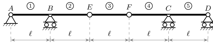
Figura 17.14. Trave di Gerber su quattro appoggi ( n_a = 4 , n_e = 5 ) con due cerniere interne ( n_c = 2 ) in E e F, collocate a \ell dagli appoggi B e C. Gradi di libertà n = 15 , vincoli m = 15 , sistema isostatico ( \nu = 0 ).
