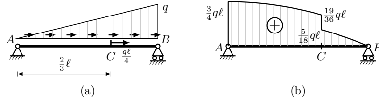
Figura 15.2. Trave con carico longitudinale triangolare q(z) = \bar{q}z/\ell e forza concentrata Z(C) = \bar{q}\ell/4 in C : (a) schema strutturale; (b) diagramma dello sforzo normale N(z) , parabolico in entrambi i tratti, con un salto -\bar{q}\ell/4 in C .
