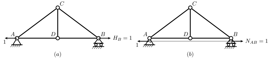
Figura 18.23. Autosoluzioni delle due varianti iperstatiche. (a) Caso 1 (iperstaticità esterna): forza unitaria H_B = 1 applicata in B sul sistema principale; la reazione del vincolo in A equilibra la forza unitaria direttamente. (b) Caso 2 (iperstaticità interna): l'asta AB (in grigio) è sconnessa in B e soggetta allo sforzo unitario N_{AB} = 1 ; la reazione del vincolo in A si applica alla sola asta AB , lasciando la struttura rimanente completamente scarica.
