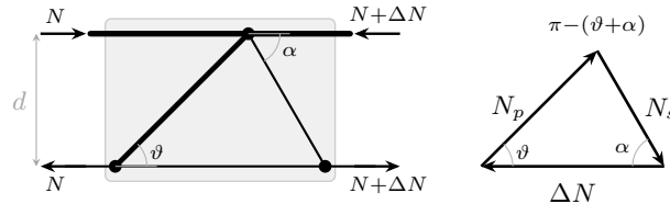
Figura 18.18. Maglia elementare del traliccio di Ritter-Mörsch e poligono delle forze al nodo del corrente superiore. Pannello sinistro: la variazione di sforzo \Delta N nei correnti — uguale in valore assoluto nel corrente superiore compresso e in quello inferiore teso — deve essere equilibrata dalle componenti orizzontali del puntone (tratto spesso, angolo \vartheta ) e della staffa (tratto sottile, angolo \alpha ). Pannello destro: poligono chiuso delle forze al nodo; l'angolo al vertice opposto a \Delta N vale \pi - (\vartheta + \alpha) , donde per il teorema dei seni le (18.22).
