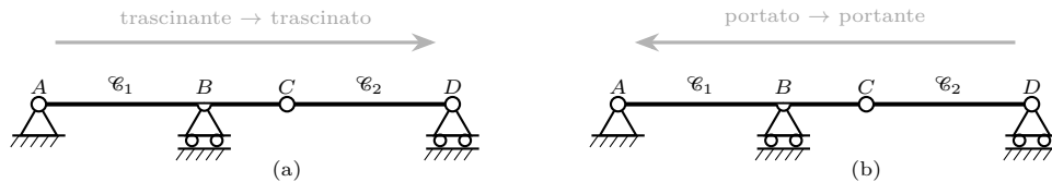
Figura 11.13. Gerarchia strutturale della trave di Gerber: (a) cascata cinematica, dal trascinante \mathcal{C}_1 al trascinato \mathcal{C}_2 (freccia da sinistra a destra); (b) cascata statica, dal portato \mathcal{C}_2 al portante \mathcal{C}_1 (freccia da destra a sinistra). Le due cascate percorrono la stessa gerarchia in direzioni opposte.
