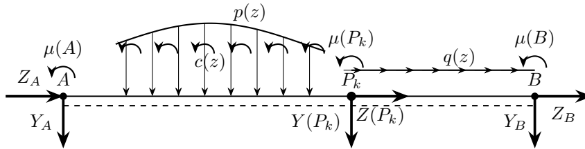
Figura 14.3. Azioni esterne su una trave rettilinea piana: carichi distribuiti p(z) , q(z) , c(z) definiti a tratti; forze e coppie concentrate Z(P_k) , Y(P_k) , \mu(P_k) in un punto interno P_k ; forze e coppie agli estremi Z_A, Y_A, \mu(A) in A e Z_B, Y_B, \mu(B) in B .
