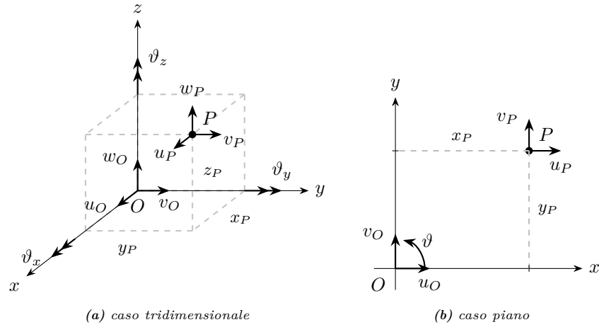
Figura 6.4. Parametri cinematici del corpo rigido e componenti dello spostamento di un punto generico P nel caso (a) tridimensionale (sei gradi di libertà: u_O , v_O , w_O , \vartheta_x , \vartheta_y , \vartheta_z ) e (b) piano (tre gradi di libertà: u_O , v_O , \vartheta ).
