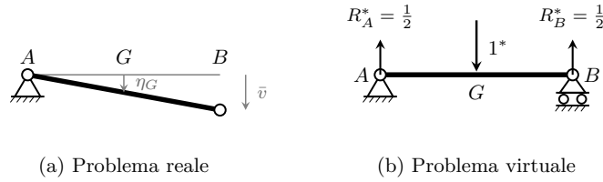
Figura 20.2. TFV per il calcolo dello spostamento \eta_G in una trave semplicemente appoggiata con cedimento in B .
