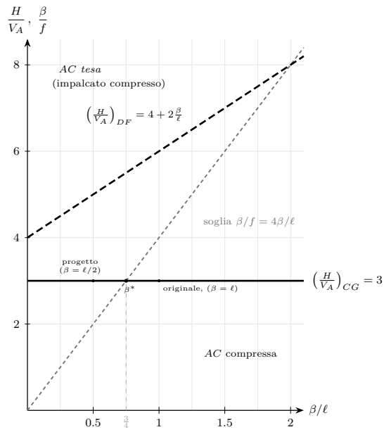
Figura 17.27. Commutazione del segno di N_{AC} al variare dello sbalzo interno \beta ( L = 4\ell , \alpha = \ell/2 , f = \ell/4 ). Per ciascuno scenario AC è tesa dove la curva H/V_A sta sopra la retta soglia \beta/f . Il peso proprio ( CG , costante = 3) supera la soglia solo per \beta < \beta^* = \frac{3}{4}\ell ; il carico centrale ( DF ) la supera sempre. Il dimensionamento \beta = \frac{1}{2}\ell cade nella regione favorevole, quello originario \beta = \ell no.
