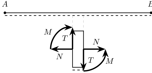
Figura 14.6. Concio di trave e convenzione di segno delle caratteristiche della sollecitazione. Sulla faccia destra (normale uscente +z^e ) N , T , M sono positivi se concordi con gli assi del riferimento intrinseco; sulla faccia sinistra (normale uscente -z^e ) i versi positivi sono opposti.
