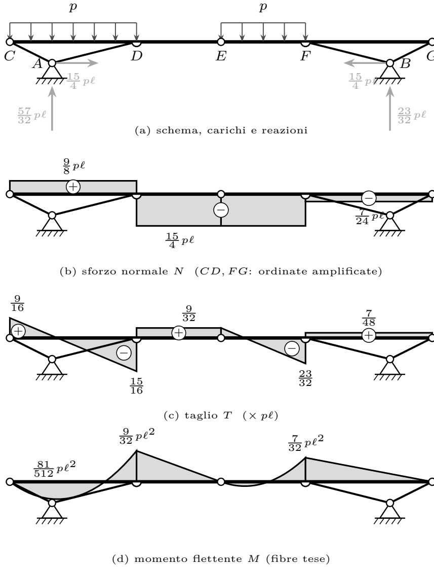
Figura 17.23. Caso (c), carico asimmetrico ( p su CD ed EF ) — (a) schema con carichi e reazioni; (b) sforzo normale N sulle travi (le bielle, scariche, portano N costante: N_{AC} = -\frac{9\sqrt{5}}{16} , N_{AD} = -\frac{39\sqrt{17}}{32} , N_{BF} = -\frac{83\sqrt{17}}{96} , N_{BG} = +\frac{7\sqrt{5}}{48} , in p\ell ); (c) taglio T ; (d) momento flettente M , dal lato delle fibre tese. Scale indipendenti; M = 0 alle cerniere C, E, G .
