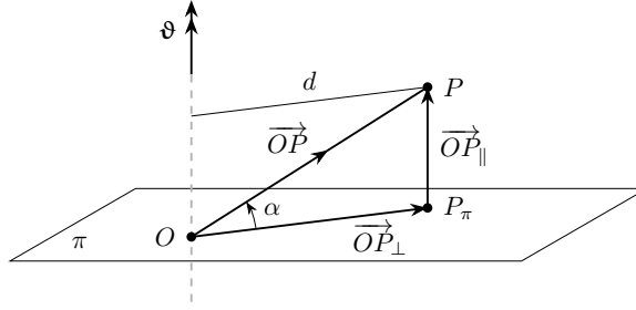
Figura 6.2. Interpretazione geometrica del termine rotazionale \Theta \times \overrightarrow{OP} : la componente \overrightarrow{OP}_\perp , ortogonale all'asse di rotazione, determina la distanza d del punto P dall'asse; lo spostamento rotazionale ha modulo |\Theta|d ed è tangente alla circonferenza di raggio d .
