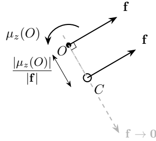
Figura 7.7. Centro di riduzione nel caso piano. Il sistema equivalente a una forza \mathbf{f} applicata in O con momento risultante \mu_z(O) si riduce alla sola forza \mathbf{f} applicata nel punto C della perpendicolare a \mathbf{f} passante per O , a distanza |\overline{OC}| = |\mu_z(O)|/|\mathbf{f}| . Al tendere di |\mathbf{f}| \rightarrow 0 a parità di \mu_z(O) il centro si allontana all'infinito: una coppia pura non ammette centro di riduzione.
