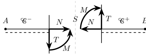
Figura 14.4. Caratteristiche della sollecitazione nella sezione S : sulla faccia destra di \mathcal{C}^- (normale uscente +z^e ) agiscono N , T , M nel verso positivo convenuto; sulla faccia sinistra di \mathcal{C}^+ le stesse grandezze agiscono con verso opposto per il terzo principio.
