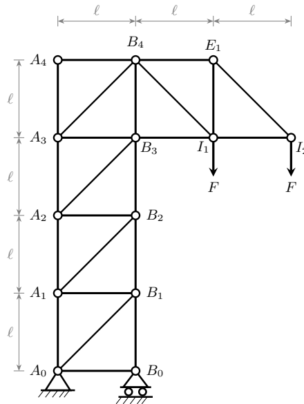
Figura 18.30. Schema reticolare di gru: fusto a quattro celle quadrate di lato \ell (correnti A posteriore, B anteriore) e braccio a sbalzo di due moduli innestato in sommità sul corrente anteriore. Cerniera in A_0 , carrello in B_0 ; carichi F ai nodi d'intradosso I_1 ed I_2 del braccio.
