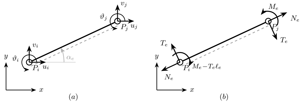
Figura 19.3. Trave di telaio e che connette i nodi P_i (iniziale) e P_j (finale), inclinata di \alpha_e rispetto all'asse globale x . La linea tratteggiata grigia indica la fibra inferiore e definisce il verso di percorrenza da P_i a P_j . (a) Cinematica: spostamenti nodali (u_i, v_i, \vartheta_i) e (u_j, v_j, \vartheta_j) nel riferimento globale (x, y) . (b) Statica: caratteristiche della sollecitazione N_e, T_e, M_e alle due sezioni di estremità con il verso convenzionale positivo; in P_i il momento vale M_e - T_e \ell_e in assenza di carichi distribuiti.
