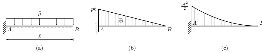
Figura 15.7. Mensola con carico uniformemente distribuito p(z) = \bar{p} (verso il basso), incastrata in A e libera in B : (a) schema strutturale; (b) diagramma del taglio T(z) , lineare decrescente, con valore \bar{p}\ell all’incastro e annullamento all’estremità libera; (c) diagramma del momento flettente M(z) , parabolico con concavità verso l’alto, sempre negativo, con valore minimo -\bar{p}\ell^2/2 all’incastro e annullamento all’estremità libera, dove il diagramma arriva con tangente orizzontale.
