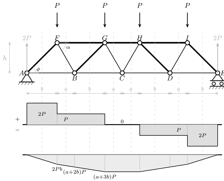
Figura 18.17. Traliccio di Ritter-Mörsch con carichi P applicati ai nodi del corrente superiore ( F, G, H, I ) e reazioni 2P agli appoggi A ed E . Le quote orizzontali indicano le proiezioni delle diagonali: b = \cot \vartheta per i puntoni (tratto spesso, compressi) e a = \cot \alpha per le staffe (tratto sottile, tese). Il diagramma del taglio è positivo nella metà sinistra ( 2P nel primo pannello, P nel secondo) e nullo tra i nodi G e H ; per antisimmetria è negativo nella metà destra. Il poligono del momento ha tetto piatto di valore (a + 3b)P tra G e H , dove il taglio è nullo, e valori nodali (a + 2b)P in B e D , 2bP in F e I .
