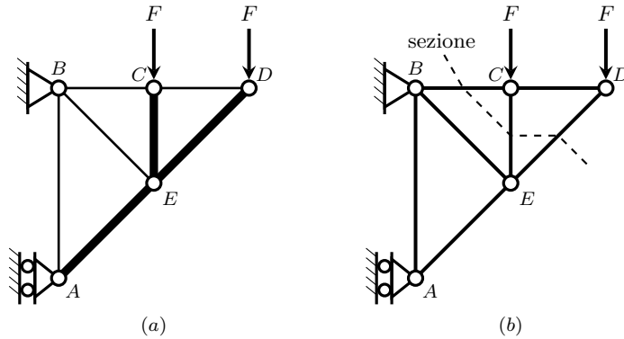
Figura 18.27. (a) Stato di sollecitazione: tratto spesso le aste compresse (puntoni AE , CE , DE ), tratto sottile le aste tese (tiranti AB , BC , CD , BE ). (b) Sezione di Ritter che isola la punta caricata \{C, D\} tagliando BC , CE ed DE . I tre poli coincidono con nodi della travatura: P_{BC} \equiv E , P_{CE} \equiv D , P_{DE} \equiv C .
