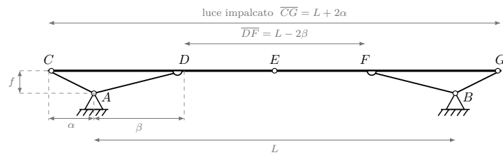
Figura 17.26. Parametri geometrici dell'arco a tre cerniere: ribassamento f , sbalzo esterno \alpha e interno \beta , luce degli appoggi L . Ne discendono \overline{CG} = L + 2\alpha e \overline{DF} = L - 2\beta ; il criterio \overline{DF} > \frac{1}{2}\overline{CG} assicura impalcato compresso sotto peso proprio.
