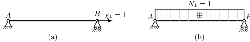
Figura 15.26. a) problema “1”: forza iperstatica unitaria \chi_1 = 1 in B ; b) sforzo normale N_1 , uniforme in trazione e pari a 1.
