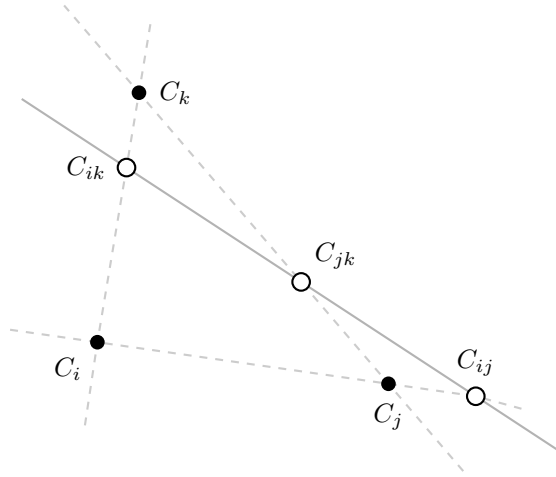
Figura 6.11. Teorema di allineamento dei centri di rotazione relativi. I tre corpi \mathcal{C}_i, \mathcal{C}_j, \mathcal{C}_k hanno centri assoluti C_i, C_j, C_k (cerchi pieni). I centri di rotazione relativi C_{ij}, C_{ik}, C_{jk} — ciascuno punto di uguale spostamento per la coppia di corpi corrispondente — sono allineati (cerchi vuoti, retta grigia). Il centro C_{ij} cade all'esterno del segmento C_i C_j , coerentemente con il teorema di Menelao.
