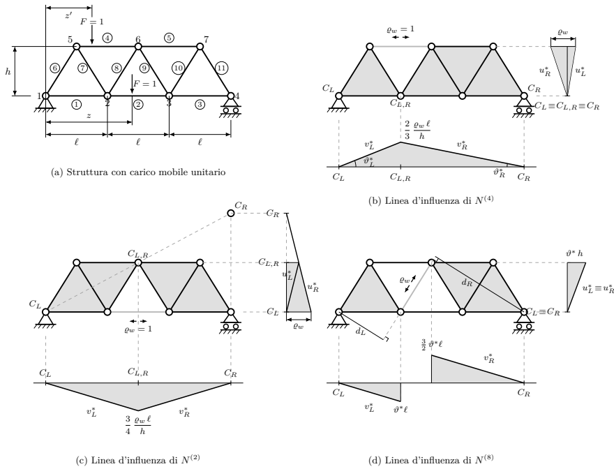
Figura 20.4. Travatura reticolare piana a correnti parallele: linee d'influenza degli sforzi normali nelle aste 4 (corrente superiore), 2 (corrente inferiore) e 8 (diagonale), sotto carico unitario verticale mobile sui nodi dei due correnti. (a) Geometria della travatura, con luce totale 3\ell e altezza h fra i correnti. (b), (c), (d) Meccanismi virtuali duali (TSV) ottenuti imponendo una distorsione longitudinale \varrho_w sull'asta in esame; il campo v^* sotto la travatura fornisce le ordinate della linea d'influenza per carichi verticali, il campo u^* a fianco le ordinate per carichi orizzontali.
