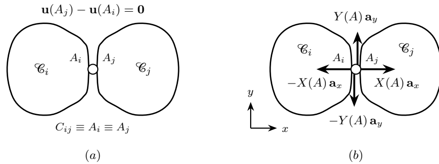
Figura 9.7. Cerniera interna fra i corpi \mathcal{C}_i e \mathcal{C}_j , applicata nel punto A che si identifica con i punti di applicazione A_i \in \mathcal{C}_i e A_j \in \mathcal{C}_j . Prestazione cinematica (a): l'equazione di vincolo \mathbf{u}(A_j) - \mathbf{u}(A_i) = \mathbf{0} impone l'uguaglianza degli spostamenti dei due corpi in A ; le rotazioni dei due corpi restano libere e non sono rappresentate. Il centro di rotazione relativo coincide con il punto di applicazione, C_{ij} \equiv A_i \equiv A_j . Prestazione statica (b): i due corpi si scambiano una forza generica X(A) \mathbf{a}_x + Y(A) \mathbf{a}_y applicata in A , in dualità con le due componenti di spostamento relativo bloccate; la coppia scambiata è identicamente nulla, in accordo con la molteplicità due.
