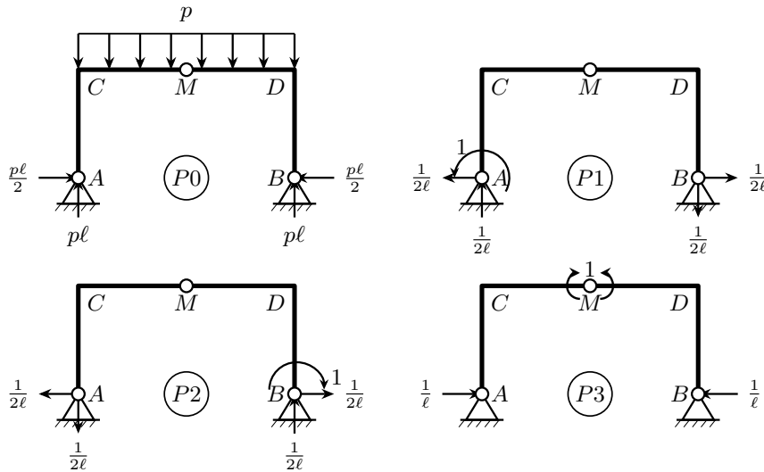
Figura 19.5. Portale a tre cerniere: reazioni vincolari nei quattro problemi di carico. Pannello P_0 : carico uniforme p sul traverso. Pannelli P_1, P_2, P_3 : coppie unitarie \chi_1, \chi_2, \chi_3 applicate rispettivamente in A, B e M.
