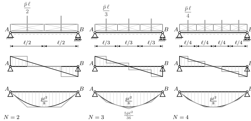
Figura 15.19. Sostituzione tra carico distribuito e carichi concentrati per la trave appoggiata, in partizioni di N = 2, 3, 4 tratti di uguale ampiezza (colonne, da sinistra a destra). Righe, dall'alto al basso: schema strutturale, diagramma del taglio T(z) , diagramma del momento flettente M(z) . In nero il caso continuo, in grigio il caso a partizione discreta. Nella riga (a) le diagonali in ciascuna sotto-area individuano il baricentro in cui è applicata la risultante \bar{p}\ell/N .
