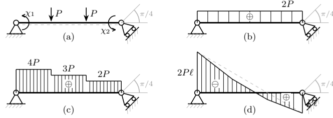
Figura 15.37. Soluzione, combinazione illustrativa \chi_1 = 2P\ell , \chi_2 = P\ell : trave reale (a); sforzo normale N = 2P (b); taglio T a gradini 4P, 3P, 2P (c); momento flettente M , spezzata da -2P\ell in A a +P\ell in B con cambio di segno in z = 5\ell/9 , con la retta di chiusura tratteggiata (d).
