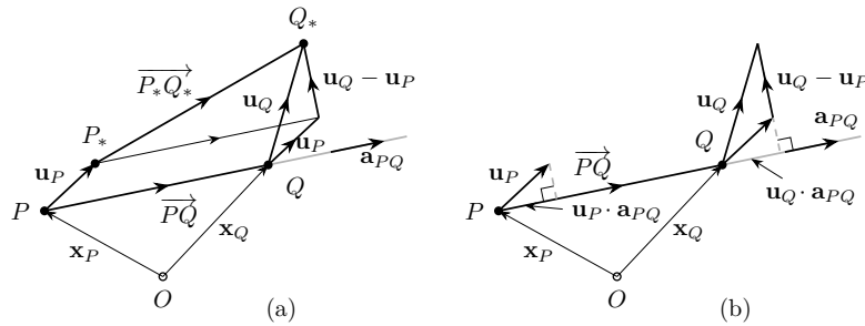
Figura 6.3. (a) Spostamenti rigidi e (b) interpretazione geometrica della condizione di ortogonalità fra il vettore posizione relativo \vec{PQ} e il vettore relativo degli spostamenti infinitesimi \mathbf{u}_Q - \mathbf{u}_P .
