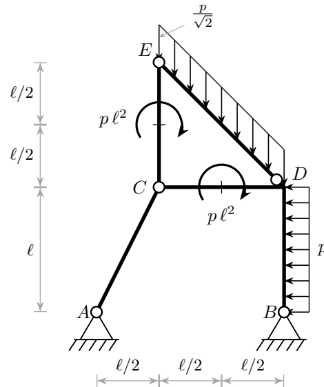
Figura 17.11. Sistemi composti a tre cerniere: arco inferiore ACDB (portante) e arco superiore CED (portato), con montante comune in chiave C e collegamento in D . Cerniere interne in C , E , D ; cerniere esterne in A e B ; nodo rigido in D . Coppie orarie p\ell^2 su CE e CD ; carico distribuito su ED (risultante p\ell ) e su DB .
