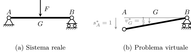
Figura 20.1. TSV per il calcolo della reazione R_A in una trave semplicemente appoggiata sotto carico F in mezzeria.
