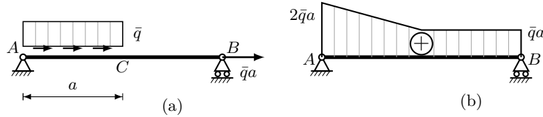
Figura 15.1. Trave con carico longitudinale distribuito \bar{q} nel tratto AC e forza concentrata \bar{q}a in B : (a) schema strutturale; (b) diagramma dello sforzo normale N(z) , in trazione su tutta la lunghezza.
