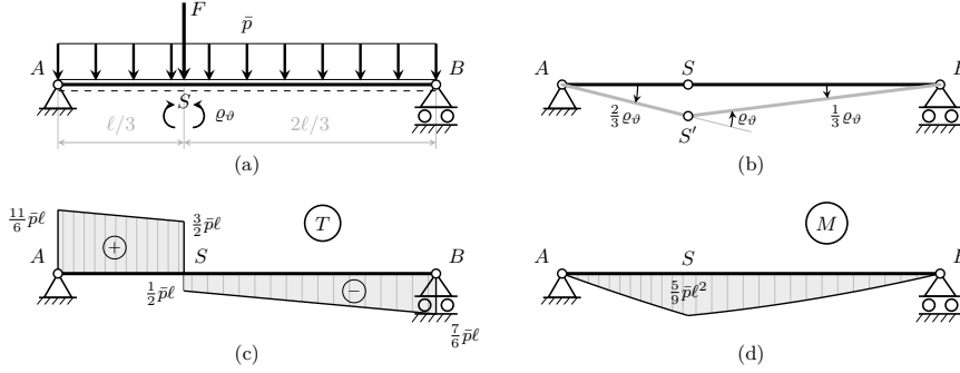
Figura 14.9. Trave appoggiata AB con distorsione rotazionale \vartheta_\vartheta > 0 in S = \ell/3 , carico distribuito uniforme p_0 e forza concentrata F = 2\bar{p}\ell in S . (a) Schema con geometria, vincoli, carichi e distorsione. (b) Configurazione deformata prodotta dalla sola distorsione \vartheta_\vartheta : i carichi non modificano la cinematica del corpo rigido. (c) Diagramma del taglio T(z) : lineare a tratti, con salto -F in S . (d) Diagramma del momento flettente M(z) : parabolico a tratti, continuo in S , nullo agli estremi. La distorsione non contribuisce ai diagrammi (c) e (d): in un sistema isostatico le distorsioni producono spostamenti ma non sollecitazioni (Oss. ??).
