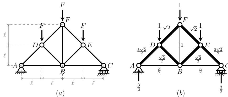
Figura 18.13. Capriata palladiana con carichi simmetrici. (a): schema strutturale con denominazione dei nodi (ogni asta è individuata dalla coppia dei nodi di estremità). (b): stato di sollecitazione, con i valori delle forze — carichi, reazioni e sforzi normali — al netto del fattore F . Tratto spesso: aste compresse — le falde AD , DF , CE , FE e le saette DB , EB (puntoni). Tratto sottile: aste tese — la catena AB , BC e il monaco BF (tiranti). Sotto gli appoggi le due reazioni verticali \frac{3}{2} .
