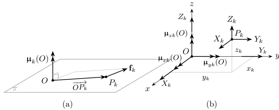
Figura 7.1. (a) Momento \boldsymbol{\mu}_k(O) rispetto al polo O della forza (P_k, \mathbf{f}_k) , definito come \boldsymbol{\mu}_k^O = \overrightarrow{OP_k} \times \mathbf{f}_k . (b) Componenti cartesiane x_k, y_k, z_k del vettore posizione \overrightarrow{OP_k} e componenti X_k, Y_k, Z_k della forza \mathbf{f}_k .
