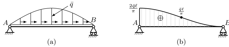
Figura 15.25. (a) problema “0”: sistema principale soggetto al solo carico; (b) sforzo normale N_0 , in trazione, decrescente da 2\bar{q}\ell/\pi in A a zero in B , con flesso in mezzeria.
