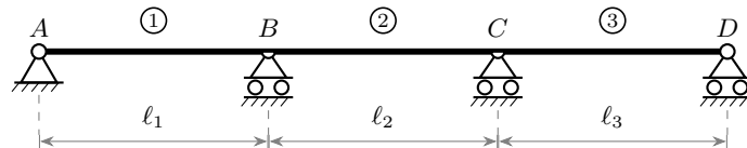
Figura 17.17. Trave continua a tre campate di luci \ell_1, \ell_2, \ell_3 ( n_e = 3 , n_a = 4 ): cerniera in A , appoggi intermedi in B e C , carrello in D . Il cerchio in A e D indica il perno della connessione; il semicerchio in B e C indica che la trave scorre sull'appoggio senza interruzione della continuità rotazionale. Gradi di libertà n = 9 , vincoli m = 11 , grado di iperstaticità g_i = 2 pari al numero di appoggi intermedi.
