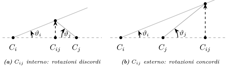
Figura 6.10. Cinematica grafica: determinazione di \vartheta_j dalla posizione dei centri e da \vartheta_i . La retta C_i C_{ij} C_j ruota di \vartheta_i attorno a C_i ; lo spostamento verticale di C_{ij} è proporzionale alla sua distanza da C_i . La retta grigia da C_j alla posizione ruotata di C_{ij} evidenzia per similitudine il rapporto |\vartheta_j|/|\vartheta_i| = |C_j C_{ij}|/|C_i C_{ij}| .
