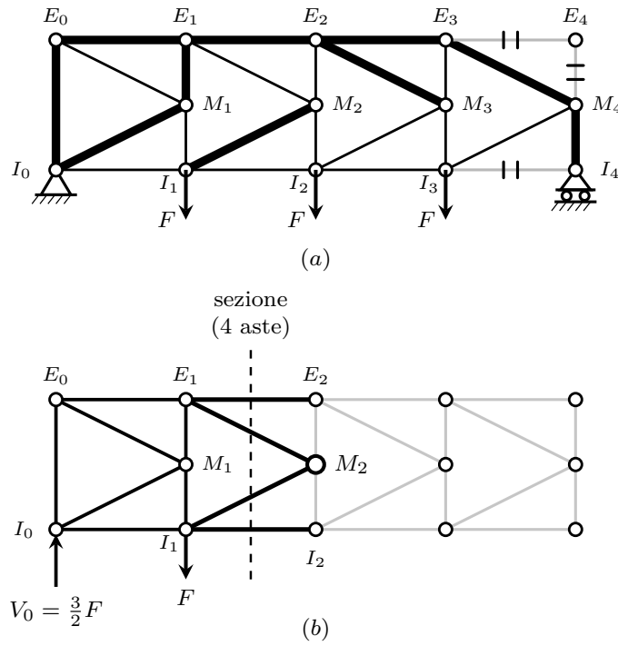
Figura 18.29. (a) Stato di sollecitazione: tratto spesso le aste compresse, tratto sottile le tese; i due trattini trasversali marcano le aste scariche ( E_3E_4 , I_3I_4 , E_4M_4 ). In ciascuna maglia a K un braccio è teso e l'altro compresso, con sforzi uguali e opposti. (b) Sezione del pannello centrale: il taglio interseca quattro aste ( E_1E_2 , I_1I_2 e i bracci M_2E_1 , M_2I_1 ). Il troncone di sinistra (in nero) si risolve aggiungendo alle tre equazioni di Ritter l'equilibrio del mid-nodo M_2 .
