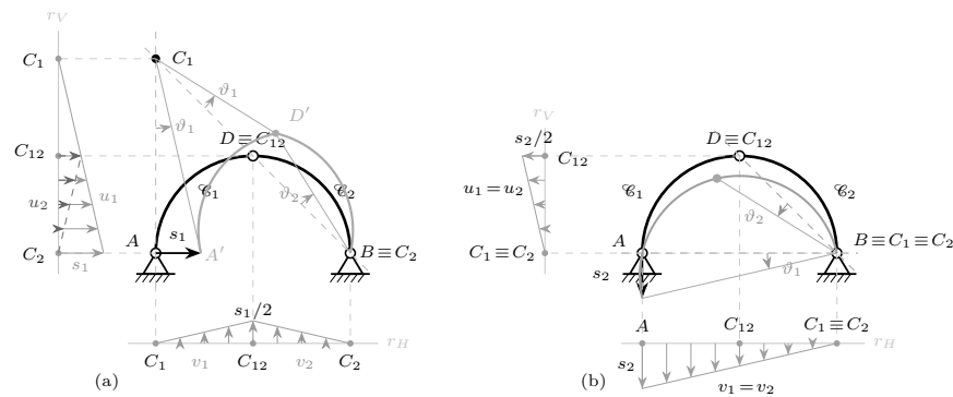
Figura 11.2. Soluzione grafica per i cedimenti esterni in A. (a) cedimento s_1 (orizzontale): tre centri distinti, C_1 all'intersezione fra la verticale per A e la retta BD. (b) cedimento s_2 (verticale): caso degenero, C_1 \equiv C_2 \equiv B , e il sistema ruota rigidamente attorno a B.
