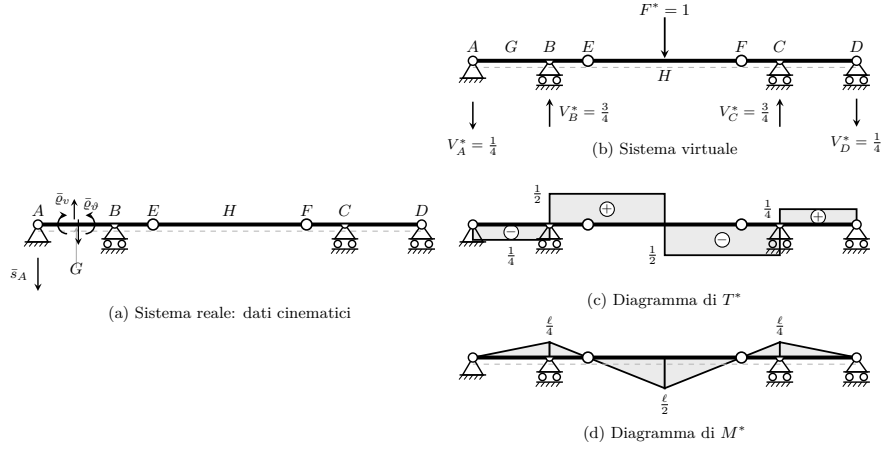
Figura 20.5. Trave di Gerber: applicazione del TFFV per il calcolo dello spostamento \eta_H in mezzzeria della travata portata EF , sotto cedimento \bar{s}_A in A e distorsioni \bar{\varrho}_v, \bar{\varrho}_\theta in G .
