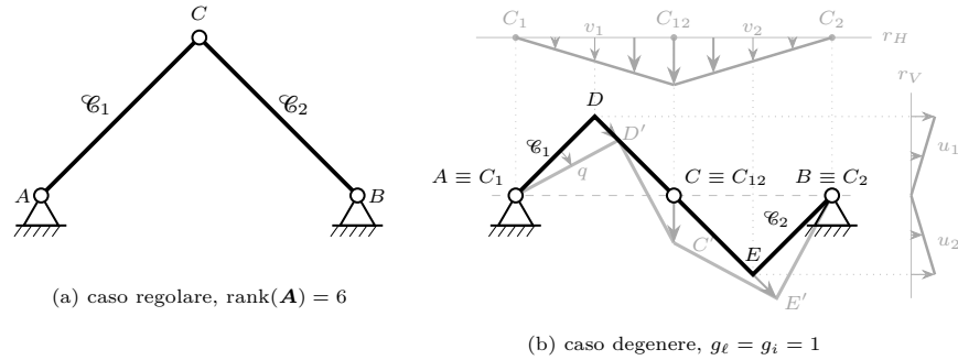
Figura 12.8. Arco a tre cerniere: (a) caso regolare, portale con A, C, B non collineari ( \text{rank}(\mathbf{A}) = 6 , isostatico); (b) caso degenere, struttura poligonale con A, C, B collineari ( g_\ell = g_i = 1 ), meccanismo parametrizzato da q e rette di proiezione r_H, r_V .
