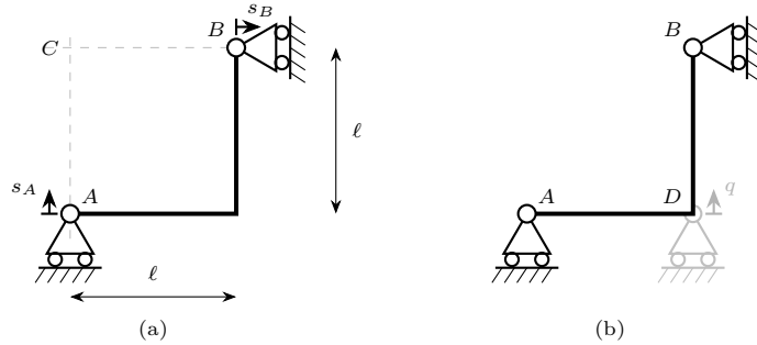
Figura 11.5. Corpo a L (Esempio 11.3): dati del problema cinematico (a) e sistema principale con carrello fittizio in D (grigio) e cedimento q (b).
