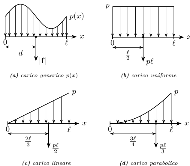
Figura 7.9. Riduzione di carichi distribuiti \mathbf{f}_L(x) = -p(x)\mathbf{a}_y con p(x) \geq 0 su un intervallo di lunghezza \ell : la risultante (freccia spessa) è applicata nel baricentro del diagramma di carico. (a) Caso generico p(x) : risultante |\mathbf{f}| applicata a distanza d . (b) Carico uniforme: |\mathbf{f}| = p\ell , d = \ell/2 . (c) Carico lineare: |\mathbf{f}| = p\ell/2 , d = 2\ell/3 . (d) Carico parabolico: |\mathbf{f}| = p\ell/3 , d = 3\ell/4 .
