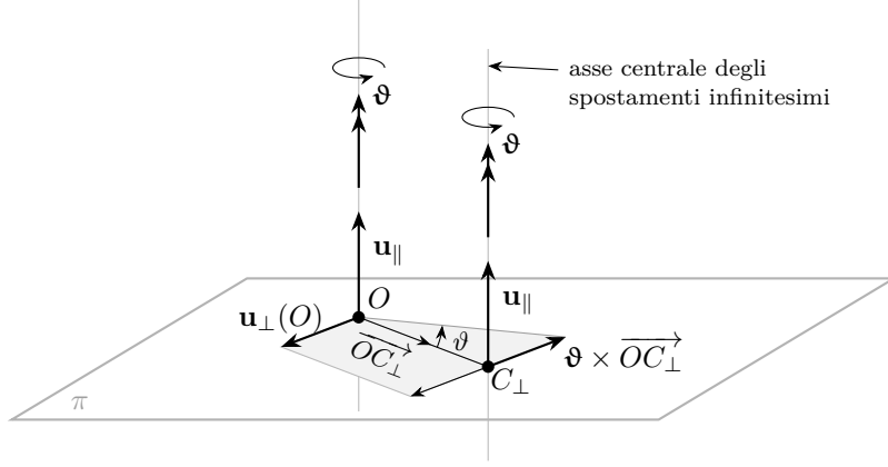
Figura 6.5. Costruzione geometrica dell'asse centrale degli spostamenti rigidi infinitesimi. Lo spostamento di O si decompone nella componente \mathbf{u}_{||} , parallela a \boldsymbol{\vartheta} e invariante per tutti i punti del corpo, e nella componente \mathbf{u}_{\perp}(O) , giacente nel piano \pi ortogonale a \boldsymbol{\vartheta} . Il punto C_{\perp} , intersezione dell'asse centrale con \pi , è determinato dalla condizione \boldsymbol{\vartheta} \times \overrightarrow{OC_{\perp}} = -\mathbf{u}_{\perp}(O) ; l'asse centrale è la retta per C_{\perp} parallela a \boldsymbol{\vartheta} .
