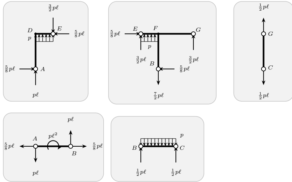
Figura 17.9. Anelli a tre cerniere: esploso dei cinque corpi liberi con i carichi attivi e le forze scambiate alle connessioni interne. La spinta \frac{5}{8}p\ell si chiude nell'anello portato ABFD ; la coppia attiva raggiunge il suolo attraverso il montante teso BF .
