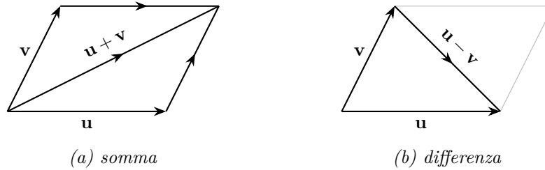
Figura 5.1. Somma e differenza di due vettori.
