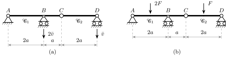
Figura 10.4. Trave di Gerber (Esempio 10.2): dato cinematico (a) e dato statico (b). Cerniera in A, carrello (intermedio) in B, cerniera interna in C, carrello (terminale) in D; poli O_1 \equiv A e O_2 \equiv C .
