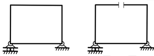
Figura 12.2. Portale rettangolare (schema ripreso nel Vol. II per il caso deformabile): maglia chiusa (sinistra, \nu = -3 ) e maglia aperta con taglio completo nella traversa superiore (destra, \nu = 0 ). Il taglio rimuove esattamente 3(p - 1) = 3 gradi di iperstaticità.
