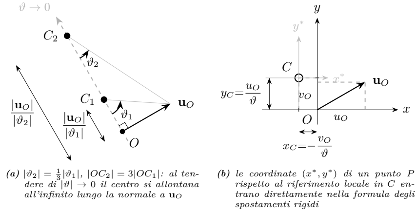
Figura 6.6. Centro di rotazione nel caso piano. (a) Costruzione geometrica: C si ottiene ruotando \mathbf{u}_O di 90^\circ nel verso di \vartheta e riscalando di 1/|\vartheta| . (b) Riferimento locale con origine in C e assi x^*, y^* paralleli a x, y : le coordinate (x^*, y^*) di un punto P entrano direttamente nella (6.38).
