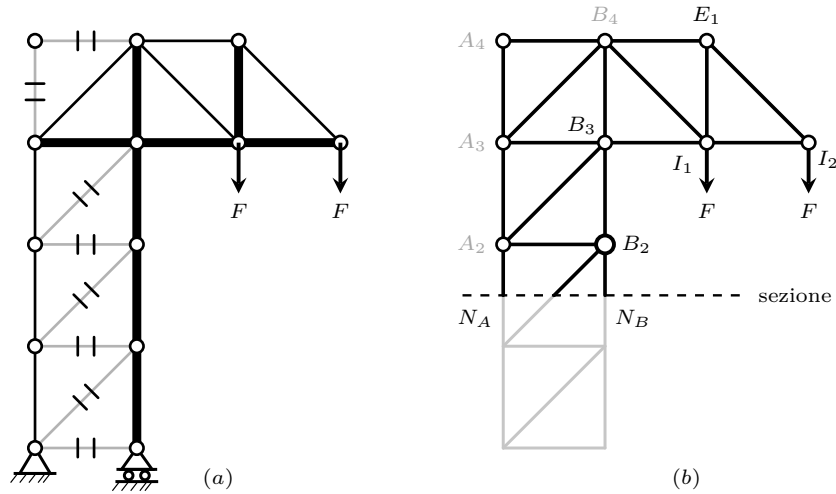
Figura 18.31. (a) Stato di sollecitazione: tratto spesso le aste compresse, tratto sottile le tese; i due trattini trasversali marcano le aste scariche (le diagonali e i traversi del fusto al di sotto della connessione, e il tratto A_3A_4 ). (b) Sezione orizzontale che recide un interpiano del fusto: il troncone superiore porta le sole due forze F ; il momento rispetto al polo B_2 dà la trazione N_A del corrente posteriore, quello rispetto al corrente posteriore la compressione N_B dell'anteriore. Entrambi non dipendono dalla quota del taglio.
