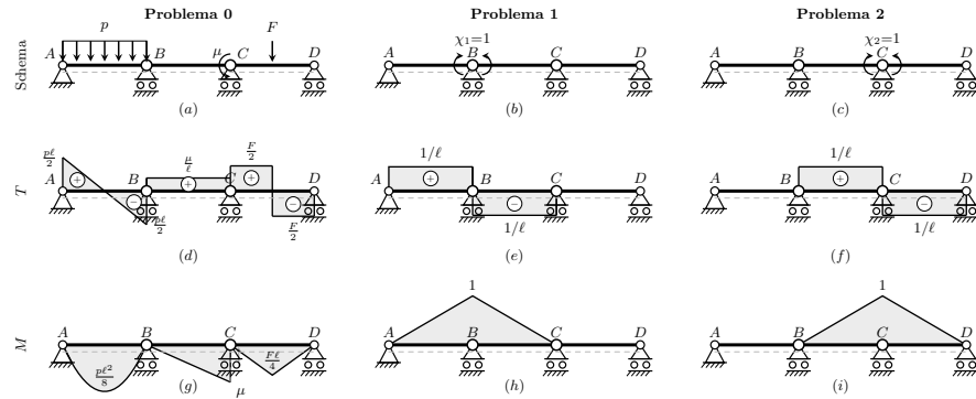
Figura 17.19. Trave continua a tre campate uguali \ell : scomposizione secondo il metodo delle forze ( N \equiv 0 ). Prima riga: (a) problema 0; (b) autosoluzione 1 ( \chi_1 = 1 , momento unitario in B); (c) autosoluzione 2 ( \chi_2 = 1 , momento unitario in C). I cerchietti indicano le cerniere interne del sistema principale; le fibre inferiori sono tratteggiate. Seconda riga: diagrammi di T con segno ( \oplus/\ominus ); (d) T_0 : lineare da +p\ell/2 a -p\ell/2 su AB, uniforme \mu/\ell su BC, gradino \pm F/2 su CD; (e) T_1 = \pm 1/\ell ; (f) T_2 = \pm 1/\ell . Terza riga: diagrammi di M ( M > 0 sotto, M < 0 sopra); (g) M_0 : parabola ( p\ell^2/8 ) su AB, triangolo con salto \Delta M = -\mu in C su BC, triangolo ( F\ell/4 ) su CD; (h) M_1 < 0 : tenda con vertice unitario in B; (i) M_2 < 0 : tenda con vertice unitario in C.
