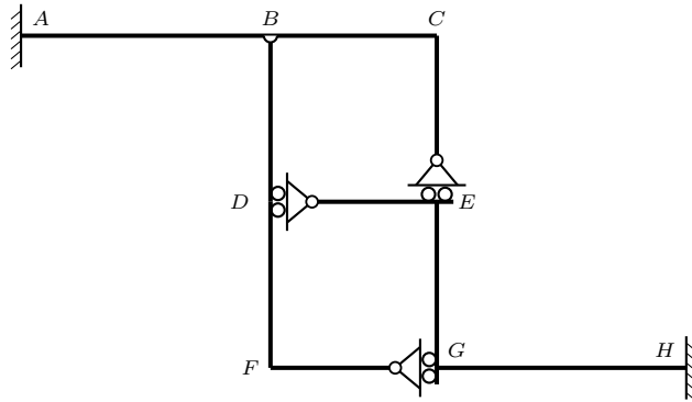
Figura 12.10. Struttura mista: due mensole ad asse spezzato \mathcal{S}_1 = ABCE (incastrata in A) e \mathcal{S}_2 = HGED (incastrata in H), collegate da una trave appoggiata \mathcal{S}_3 = BDFG (cerniera in B, carrello in G). I carrelli in D ed E aggiungono due vincoli semplici allo schema isostatico di riferimento: \nu = -2 , iperstatica di grado 2.
