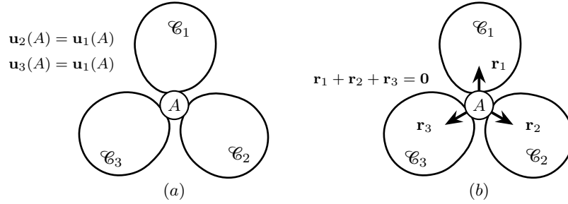
Figura 4.12. Cerniera multipla fra i corpi \mathcal{C}_1, \mathcal{C}_2, \mathcal{C}_3 nel punto A . Prestazione cinematica (a): le equazioni di vincolo \mathbf{u}_2(A) = \mathbf{u}_1(A) e \mathbf{u}_3(A) = \mathbf{u}_1(A) impongono l'uguaglianza degli spostamenti dei tre corpi in A ; le rotazioni dei tre corpi restano libere e non sono rappresentate. Il centro di rotazione relativo di ogni coppia di corpi coincide con A . Prestazione statica (b): i tre corpi si scambiano in A tre forze \mathbf{r}_1, \mathbf{r}_2, \mathbf{r}_3 di direzione arbitraria, soggette all'equilibrio del nodo \sum_i \mathbf{r}_i = \mathbf{0} ; nessuna coppia scambiata. Le incognite indipendenti sono le componenti di \mathbf{r}_2 e \mathbf{r}_3 (per un totale di 2(k-1) = 4 ), in accordo con la molteplicità.
