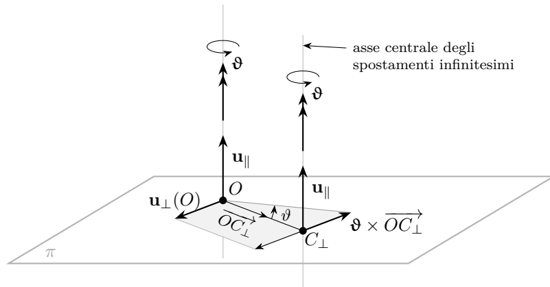
Figura 1.5. Costruzione geometrica dell'asse centrale degli spostamenti rigidi infinitesimi. Lo spostamento di O si decompone nella componente \mathbf{u}_{\parallel} , parallela a \boldsymbol{\vartheta} e invariante per tutti i punti del corpo, e nella componente \mathbf{u}_{\perp}(O) , giacente nel piano \pi ortogonale a \boldsymbol{\vartheta} . Il punto C_{\perp} , intersezione dell'asse centrale con \pi , è determinato dalla condizione \boldsymbol{\vartheta} \times \overrightarrow{OC_{\perp}} = -\mathbf{u}_{\perp}(O) ; l'asse centrale è la retta per C_{\perp} parallela a \boldsymbol{\vartheta} .
