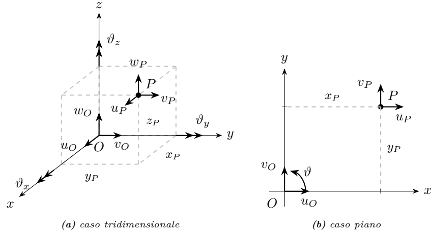
Figura 1.4. Parametri cinematici del corpo rigido e componenti dello spostamento di un punto generico P nel caso (a) tridimensionale (sei gradi di libertà: u_O , v_O , w_O , \vartheta_x , \vartheta_y , \vartheta_z ) e (b) piano (tre gradi di libertà: u_O , v_O , \vartheta ).
