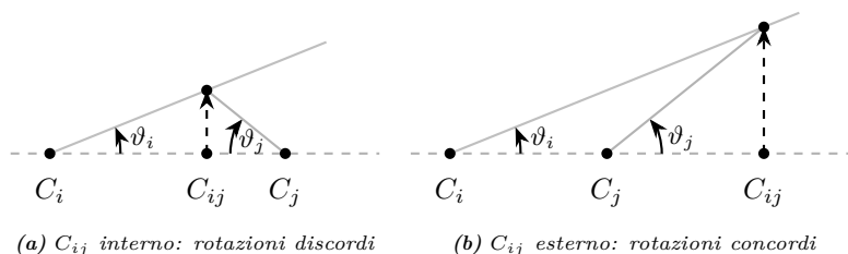
Figura 1.10. Cinematica grafica: determinazione di \vartheta_j dalla posizione dei centri e da \vartheta_i . La retta C_i C_{ij} C_j ruota di \vartheta_i attorno a C_i ; lo spostamento verticale di C_{ij} è proporzionale alla sua distanza da C_i . La retta grigia da C_j alla posizione ruotata di C_{ij} evidenzia per similitudine il rapporto |\vartheta_j|/|\vartheta_i| = |C_j C_{ij}|/|C_i C_{ij}| .
