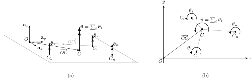
Figura 1.7. Composizione di n rotazioni infinitesime nel piano. (a) Vista tridimensionale: le rotazioni sono vettori assiali \vartheta_i ortogonali al piano \pi , che si sommano nella risultante \vartheta = \sum_i \vartheta_i in C . (b) Vista nel piano (x, y) : ampiezze \vartheta_i come archi orientati (positivi se antiorari) e centro risultante C nel baricentro dei C_i . Il centro C è individuato da \overrightarrow{OC} = (\sum_i \vartheta_i \overrightarrow{OC_i}) / \vartheta o, in forma equivalente, da \sum_i \vartheta_i \overrightarrow{CC_i} = \mathbf{0} (freccie grigie in (b)).
