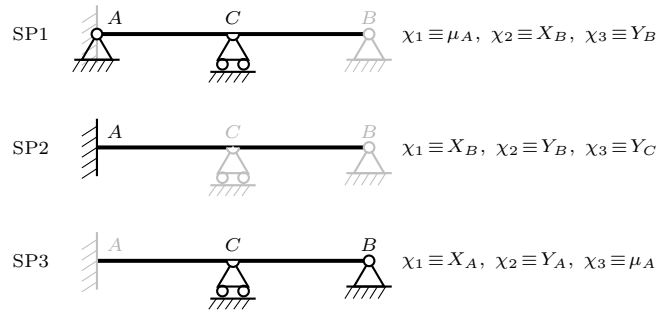
Figura 6.10. Trave iperstatica di grado 3 (Esempio 6.7): tre sistemi principali isostatici. I vincoli rimossi sono in grigio; le corrispondenti reazioni diventano le incognite iperstatiche \chi_1 , \chi_2 , \chi_3 .
