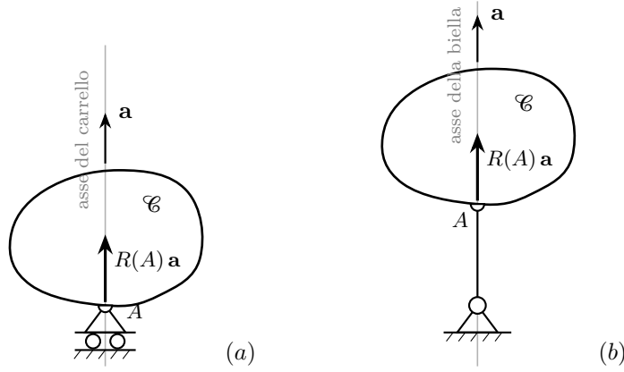
Figura 4.2. Prestazione statica del carrello (a) e della biella (b): la reazione vincolare si riduce alla sola forza R(A)\mathbf{a} diretta lungo l'asse, in dualità con la componente di spostamento bloccata; le componenti reattive nulle (coppia e forza in \mathbf{a}^\perp ) non sono rappresentate, in accordo con la molteplicità uno. Nella biella, la forza è trasmessa al corpo \mathcal{C} dall'asta lungo il proprio asse.
