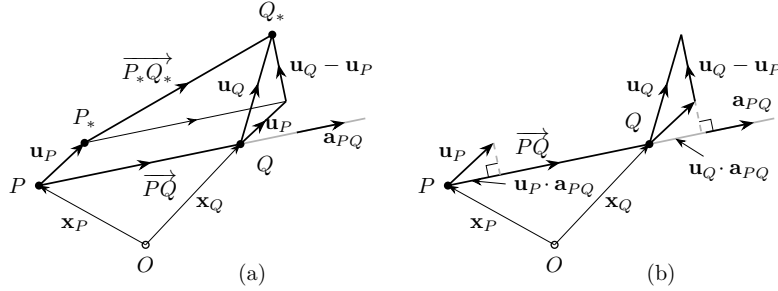
Figura 1.3. (a) Spostamenti rigidi e (b) interpretazione geometrica della condizione di ortogonalità fra il vettore posizione relativo \overrightarrow{PQ} e il vettore relativo degli spostamenti infinitesimi \mathbf{u}_Q - \mathbf{u}_P .
