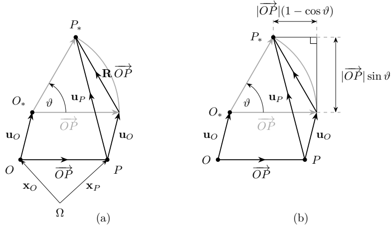
Figura 1.1. (a) Rappresentazione geometrica di una traslazione e di una rotazione finita nel piano, dove il punto O si sposta in O_* e il punto P si sposta in P_* , con origine del sistema di riferimento in \Omega . Il vettore \mathbf{u}(O) rappresenta la traslazione di O , mentre \mathbf{u}(P) è lo spostamento totale di P , e \mathbf{R}\overrightarrow{OP} è il vettore \overrightarrow{OP} ruotato di \vartheta . (b) Scomposizione dello spostamento del punto P in P_* come somma della traslazione \mathbf{u}(O) e della rotazione, con la componente rotazionale decomposta nelle direzioni ortogonale (|\overrightarrow{OP}| \sin \vartheta) e parallela (|\overrightarrow{OP}|(1 - \cos \vartheta)) rispetto al vettore posizione \overrightarrow{OP} .
