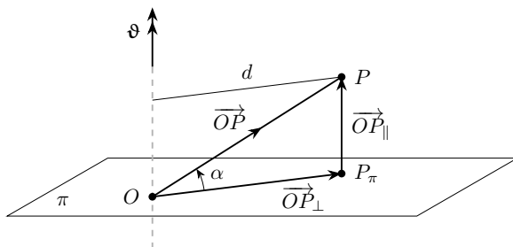
Figura 1.2. Interpretazione geometrica del termine rotazionale \boldsymbol{\vartheta} \times \overrightarrow{OP} : la componente \overrightarrow{OP}_\perp , ortogonale all'asse di rotazione, determina la distanza d del punto P dall'asse; lo spostamento rotazionale ha modulo |\boldsymbol{\vartheta}| d ed è tangente alla circonferenza di raggio d .
