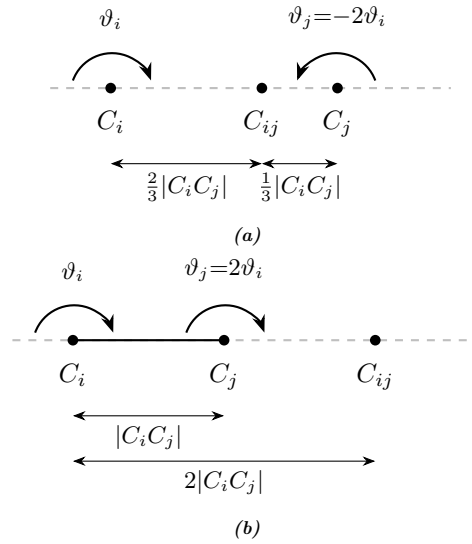
Figura 1.9. Allineamento dei centri di rotazione C_i , C_j e C_{ij} con |\vartheta_j| = 2|\vartheta_i| . (a) Rotazioni discordi ( \vartheta_i > 0 , \vartheta_j = -2\vartheta_i ): C_{ij} cade all'interno del segmento C_i C_j , a distanza \frac{2}{3}|C_i C_j| da C_i . (b) Rotazioni concordi ( \vartheta_i > 0 , \vartheta_j = 2\vartheta_i ): C_{ij} cade all'esterno, oltre C_j , a distanza 2|C_i C_j| da C_i .
