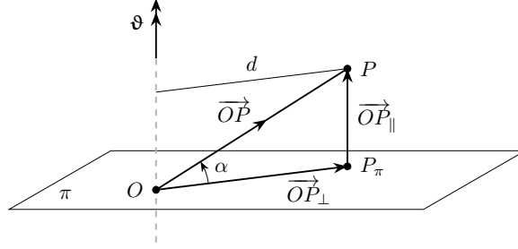
Figura 2.4. Interpretazione geometrica del termine rotazionale \vartheta \times \vec{OP} : la componente \vec{OP}_\perp , ortogonale all'asse di rotazione, determina la distanza d del punto P dall'asse; lo spostamento rotazionale ha modulo |\vartheta|d ed è tangente alla circonferenza di raggio d .
