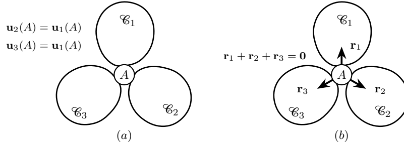
Figura 7.12. Cerniera multipla fra i corpi \mathcal{C}_1, \mathcal{C}_2, \mathcal{C}_3 nel punto A . Prestazione cinematica (a): le equazioni di vincolo \mathbf{u}_2(A) = \mathbf{u}_1(A) e \mathbf{u}_3(A) = \mathbf{u}_1(A) impongono l'uguaglianza degli spostamenti dei tre corpi in A ; le rotazioni dei tre corpi restano libere e non sono rappresentate. Il centro di rotazione relativo di ogni coppia di corpi coincide con A . Prestazione statica (b): i tre corpi si scambiano in A tre forze \mathbf{r}_1, \mathbf{r}_2, \mathbf{r}_3 di direzione arbitraria, soggette all'equilibrio del nodo \sum_i \mathbf{r}_i = \mathbf{0} ; nessuna coppia scambiata. Le incognite indipendenti sono le componenti di \mathbf{r}_2 e \mathbf{r}_3 (per un totale di 2(k-1) = 4 ), in accordo con la molteplicità.
