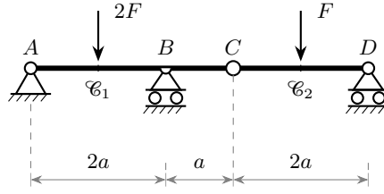
Figura 8.3. La trave di Gerber sotto carico attivo: una forza 2F verso il basso nel punto medio di AB , su \mathcal{C}_1 , e una forza F verso il basso nel punto medio di \mathcal{C}_2 . Stesso sistema di Fig. 8.1, qui nella lettura statica.
