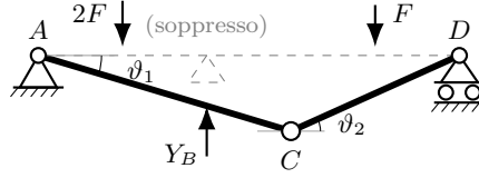
Figura 8.5. Il meccanismo usato per determinare Y_B : si sopprime il carrello in B . \mathcal{C}_1 ruota di \vartheta_1 attorno alla cerniera in A ; \mathcal{C}_2 accompagna il moto ruotando di \vartheta_2 = -\frac{3}{2}\vartheta_1 attorno a C , in modo da lasciare fermo il punto D , dove il carrello non è stato toccato.
