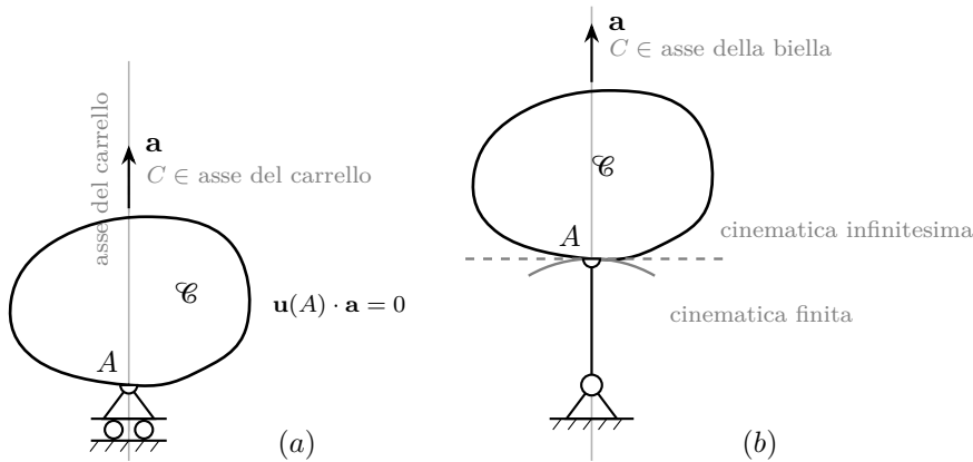
Figura 7.1. Vincolo semplice di carrello: simbolo convenzionale (a) e realizzazione meccanica tramite biella (b). L'equazione di vincolo \mathbf{u}(A) \cdot \mathbf{a} = 0 annulla la componente di spostamento di A lungo l'asse \mathbf{a} ; le componenti libere — traslazione lungo \mathbf{a}^\perp e rotazione — non sono rappresentate. Per la biella, la cinematica finita è un arco di circonferenza centrato nel perno al suolo; nell'ipotesi di spostamenti infinitesimi essa coincide con la tangente in A , e le prestazioni cinematiche della biella si riducono a quelle del carrello. In entrambi i casi il centro di rotazione assoluto giace sulla retta per A in direzione \mathbf{a} .
