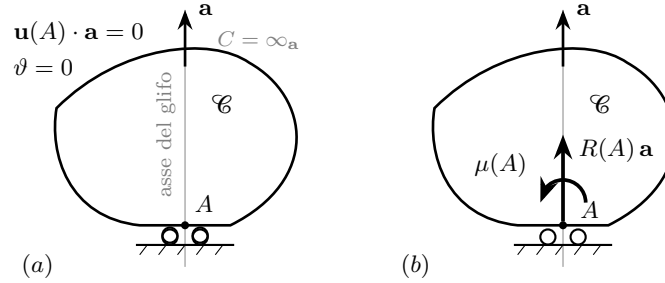
Figura 7.8. Glifo esterno applicato al corpo \mathcal{C} in A , con asse \mathbf{a} . Prestazione cinematica (a): le equazioni di vincolo \mathbf{u}(A) \cdot \mathbf{a} = 0 e \vartheta = 0 impediscono la traslazione di A lungo \mathbf{a} e la rotazione del corpo; il centro di rotazione assoluto è all’infinito sulla retta dell’asse, C = \infty_{\mathbf{a}} . Prestazione statica (b): la reazione vincolare consta di una forza R(A)\mathbf{a} diretta lungo l’asse e di una coppia \mu(A) , in dualità rispettivamente con la traslazione lungo \mathbf{a} e con la rotazione bloccate, in accordo con la molteplicità due.
