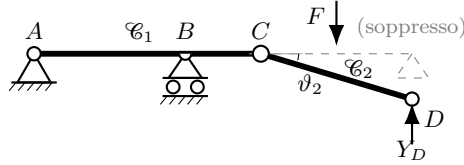
Figura 8.4. Il meccanismo usato per determinare Y_D : si sopprime (concettualmente) il carrello in D , in grigio nella sua posizione originaria. Cerniera in A e carrello in B bloccano \mathcal{C}_1 , che resta fermo; \mathcal{C}_2 è allora libero di ruotare, di un angolo virtuale \vartheta_2 , attorno al punto fisso C . Solo F e la reazione incognita Y_D compiono lavoro in questo moto.
