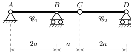
Figura 8.1. La trave Gerber: due corpi rigidi \mathcal{C}_1 , \mathcal{C}_2 connessi da una cerniera in C ; cerniera al suolo in A , carrelli verticali in B e D .
