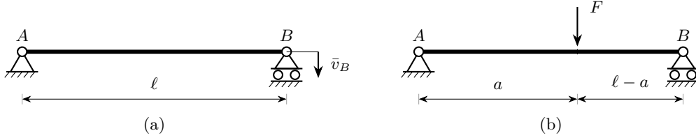
Figura 8.8. Trave semplicemente appoggiata (Esempio 8.1): dato cinematico (a) e dato statico (b). In entrambi i casi la cerniera è in A = (0, 0) e il carrello verticale in B = (\ell, 0) , con polo O \equiv A .
