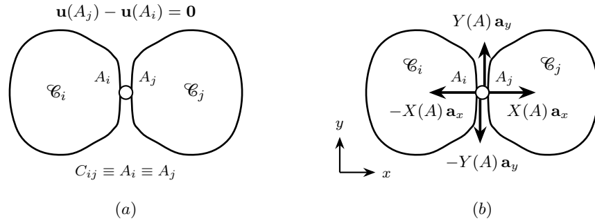
Figura 7.7. Cerniera interna fra i corpi \mathcal{C}_i e \mathcal{C}_j , applicata nel punto A che si identifica con i punti di applicazione A_i \in \mathcal{C}_i e A_j \in \mathcal{C}_j . Prestazione cinematica (a): l'equazione di vincolo \mathbf{u}(A_j) - \mathbf{u}(A_i) = \mathbf{0} impone l'uguaglianza degli spostamenti dei due corpi in A ; le rotazioni dei due corpi restano libere e non sono rappresentate. Il centro di rotazione relativo coincide con il punto di applicazione, C_{ij} \equiv A_i \equiv A_j . Prestazione statica (b): i due corpi si scambiano una forza generica X(A) \mathbf{a}_x + Y(A) \mathbf{a}_y applicata in A , in dualità con le due componenti di spostamento relativo bloccate; la coppia scambiata è identicamente nulla, in accordo con la molteplicità due.
