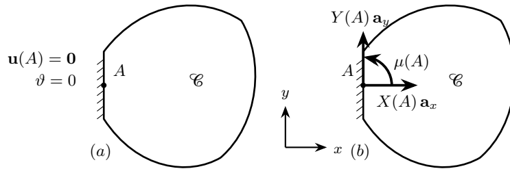
Figura 7.10. Incastro applicato al corpo \mathcal{C} nel punto A . Prestazione cinematica (a): nessuno spostamento è ammesso, né traslazione né rotazione ( \mathbf{u}(A) = \mathbf{0} , \vartheta = 0 ); il corpo è completamente bloccato. Prestazione statica (b): la reazione vincolare è una forza generica X(A)\mathbf{a}_x + Y(A)\mathbf{a}_y e una coppia \mu(A) , applicate in A , in accordo con la molteplicità tre.
