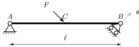
Figura 8.10. Trave appoggiata con carrello inclinato (Esempio 8.2 e Esempio 8.3): cerniera in A , carrello in B con asse \mathbf{a} a 45^\circ rispetto alla verticale, polo O \equiv A . Nel dato statico è applicata in C = (\ell/2, 0) una forza F inclinata di 45^\circ sull'orizzontale.
