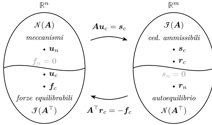
Figura 8.7. Struttura duale dei problemi cinematico \mathbf{A}\mathbf{u} = \mathbf{s} e statico \mathbf{A}^\top \mathbf{r} = -\mathbf{f} .
