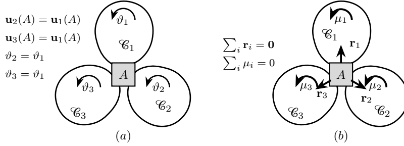
Figura 7.13. Incastro multiplo fra i corpi \mathcal{C}_1 , \mathcal{C}_2 , \mathcal{C}_3 nel punto A . Prestazione cinematica (a): le equazioni di vincolo \mathbf{u}_2(A) = \mathbf{u}_1(A) , \mathbf{u}_3(A) = \mathbf{u}_1(A) , \vartheta_2 = \vartheta_1 , \vartheta_3 = \vartheta_1 impongono l'uguaglianza degli spostamenti e delle rotazioni dei tre corpi in A ; i tre corpi si comportano come un unico corpo rigido nel nodo. Prestazione statica (b): i tre corpi si scambiano in A forze \mathbf{r}_1, \mathbf{r}_2, \mathbf{r}_3 e coppie \mu_1, \mu_2, \mu_3 di direzione e verso arbitrari, soggette all'equilibrio del nodo \sum_i \mathbf{r}_i = \mathbf{0} e \sum_i \mu_i = 0 . Le incognite indipendenti sono le componenti delle coppie e delle forze relative a \mathcal{C}_2 e \mathcal{C}_3 (per un totale di 3(k-1) = 6 ), in accordo con la molteplicità.
