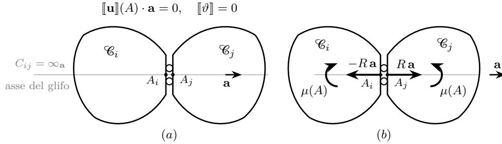
Figura 7.9. Glifo interno fra i corpi \mathcal{C}_i e \mathcal{C}_j con asse \mathbf{a} . Prestazione cinematica (a): le equazioni di vincolo [\![\mathbf{u}]\!](A) \cdot \mathbf{a} = 0 e [\![\vartheta]\!] = 0 impongono l'uguaglianza delle componenti di spostamento dei due corpi lungo \mathbf{a} e l'uguaglianza delle rotazioni \vartheta_i e \vartheta_j ; lo scorrimento relativo lungo \mathbf{a}^\perp resta libero. Il centro di rotazione relativo è all'infinito sulla retta dell'asse, C_{ij} = \infty_{\mathbf{a}} . Prestazione statica (b): i due corpi si scambiano una forza R\mathbf{a} diretta lungo l'asse e una coppia \mu(A) , uguali e opposte, in dualità rispettivamente con la componente di spostamento relativo lungo \mathbf{a} e con la rotazione relativa bloccate, in accordo con la molteplicità due.
