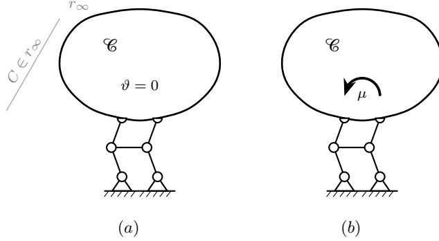
Figura 7.4. Bipendolo esterno applicato al corpo \mathcal{C} , realizzato meccanicamente come pantografo a doppio parallelogramma. Prestazione cinematica (a): l'equazione di vincolo \vartheta = 0 annulla la rotazione del corpo, lasciando libere le due componenti di traslazione, non rappresentate; il centro di rotazione assoluto giace sulla retta impropria r_\infty . Prestazione statica (b): la reazione vincolare si riduce alla sola coppia \mu , in dualità con la rotazione bloccata; la forza risultante è identicamente nulla, in accordo con la molteplicità uno.
