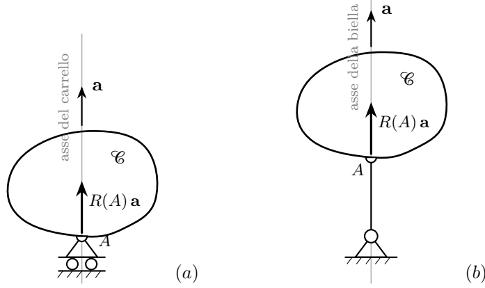
Figura 7.2. Prestazione statica del carrello (a) e della biella (b): la reazione vincolare si riduce alla sola forza R(A) \mathbf{a} diretta lungo l'asse, in dualità con la componente di spostamento bloccata; le componenti reattive nulle (coppia e forza in \mathbf{a}^\perp ) non sono rappresentate, in accordo con la molteplicità uno. Nella biella, la forza è trasmessa al corpo \mathcal{C} dall'asta lungo il proprio asse.
