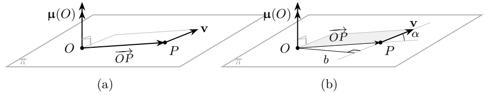
Figura 2.7. Momento polare di un vettore applicato: (a) definizione come prodotto vettoriale \vec{OP} \times \mathbf{v} ; (b) calcolo come prodotto del modulo |\mathbf{v}| per il braccio b .
