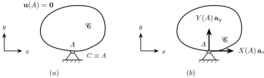
Figura 7.6. Cerniera esterna applicata al corpo \mathcal{C} nel punto A . Prestazione cinematica (a): il punto A è fisso, \mathbf{u}(A) = \mathbf{0} , e il corpo ruota liberamente attorno ad esso; il centro di rotazione assoluto coincide con il punto di applicazione, C \equiv A . Prestazione statica (b): la reazione vincolare è una forza generica X(A) \mathbf{a}_x + Y(A) \mathbf{a}_y applicata in A , in dualità con le due componenti di spostamento bloccate; la coppia reattiva è identicamente nulla, in accordo con la molteplicità due.
