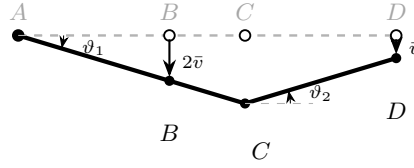
Figura 8.2. Configurazione deformata della trave di Gerber (in grigio tratteggiato la configurazione di riferimento, non deformata), soluzione del problema cinematico del Paragrafo ??; spostamenti esagerati per chiarezza. \mathcal{C}_1 ruota rigidamente attorno ad A dell'angolo \vartheta_1 = -\bar{v}/a (orario); \mathcal{C}_2 ruota, indipendentemente da \mathcal{C}_1 , dell'angolo \vartheta_2 = +\bar{v}/a (antiorario) attorno al punto C , che segue \mathcal{C}_1 senza distaccarsene. Il punto C non presenta alcuna discontinuità di spostamento — le due travi restano a contatto — ma la pendenza della configurazione deformata cambia bruscamente in C : è la manifestazione visibile dello svincolo rotazionale della cerniera interna.
