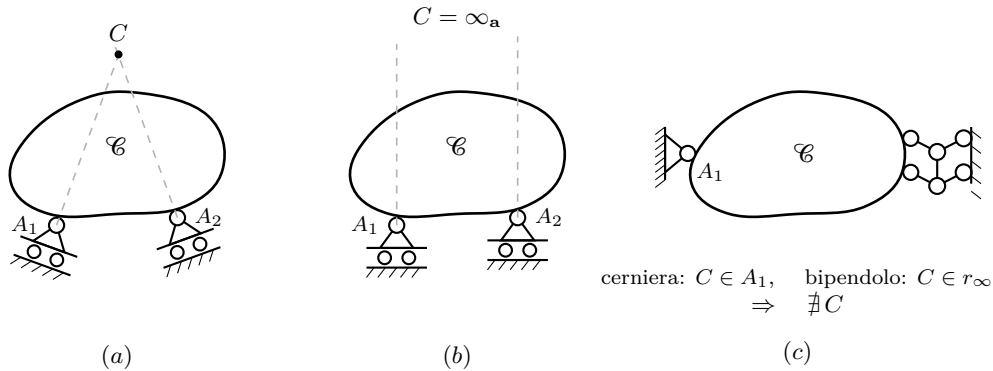
Figura 7.11. Il centro di rotazione assoluto di un vincolo composto come intersezione dei luoghi del centro dei vincoli componenti: (a) cerniera, (b) glifo, (c) incastro.
