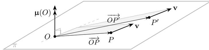
Figura 2.9. Invarianza del momento polare per traslazione del punto di applicazione lungo la linea d'azione.
