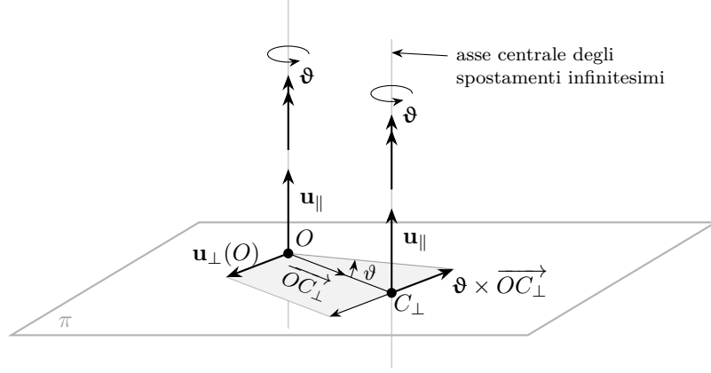
Figura 3.6. Costruzione geometrica dell'asse centrale degli spostamenti rigidi infinitesimi. Lo spostamento di O si decompone nella componente \mathbf{u}_{\parallel} , parallela a \boldsymbol{\vartheta} e invariante per tutti i punti del corpo, e nella componente \mathbf{u}_{\perp}(O) , giacente nel piano \pi ortogonale a \boldsymbol{\vartheta} . Il punto C_{\perp} , intersezione dell'asse centrale con \pi , è determinato dalla condizione \boldsymbol{\vartheta} \times \overrightarrow{OC_{\perp}} = -\mathbf{u}_{\perp}(O) ; l'asse centrale è la retta per C_{\perp} parallela a \boldsymbol{\vartheta} .
