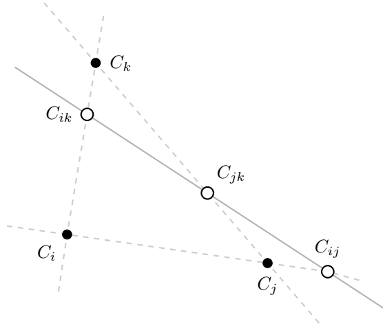
Figura 3.12. Teorema di allineamento dei centri di rotazione relativi. I tre corpi \mathcal{C}_i, \mathcal{C}_j, \mathcal{C}_k hanno centri assoluti C_i, C_j, C_k (cerchi pieni). I centri di rotazione relativi C_{ij}, C_{ik}, C_{jk} — ciascuno punto di uguale spostamento per la coppia di corpi corrispondente — sono allineati (cerchi vuoti, retta grigia). Il centro C_{ij} cade all'esterno del segmento C_i C_j , coerentemente con il teorema di Menelao.
