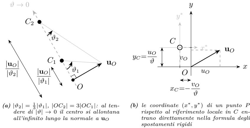
Figura 3.7. Centro di rotazione nel caso piano. (a) Costruzione geometrica: C si ottiene ruotando \mathbf{u}_O di 90^\circ nel verso di \vartheta e riscalando di 1/|\vartheta| . (b) Riferimento locale con origine in C e assi x^*, y^* paralleli a x, y : le coordinate (x^*, y^*) di un punto P entrano direttamente nella (3.59).
